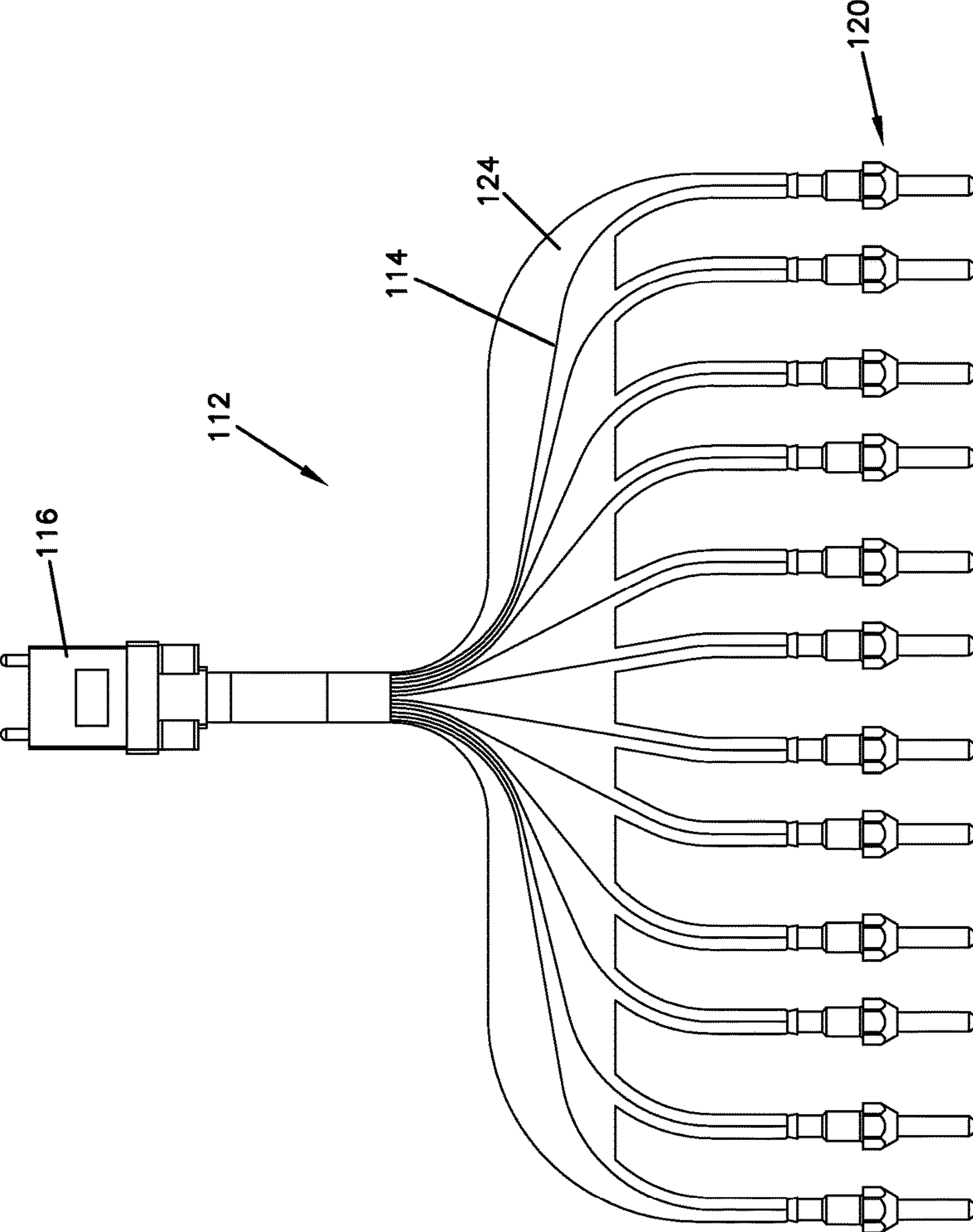
FIG. 34
