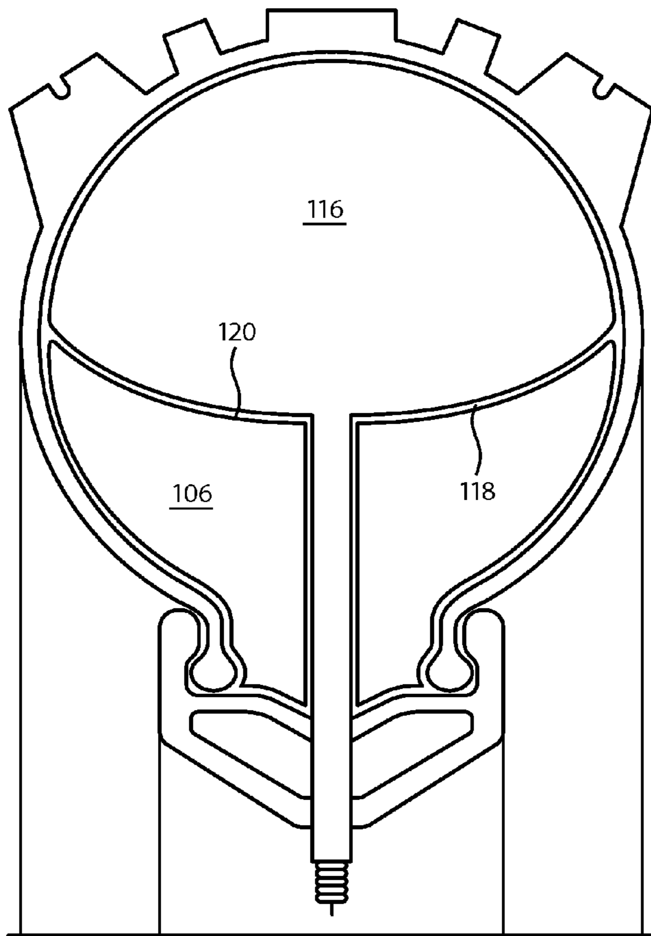
FIG. 4
