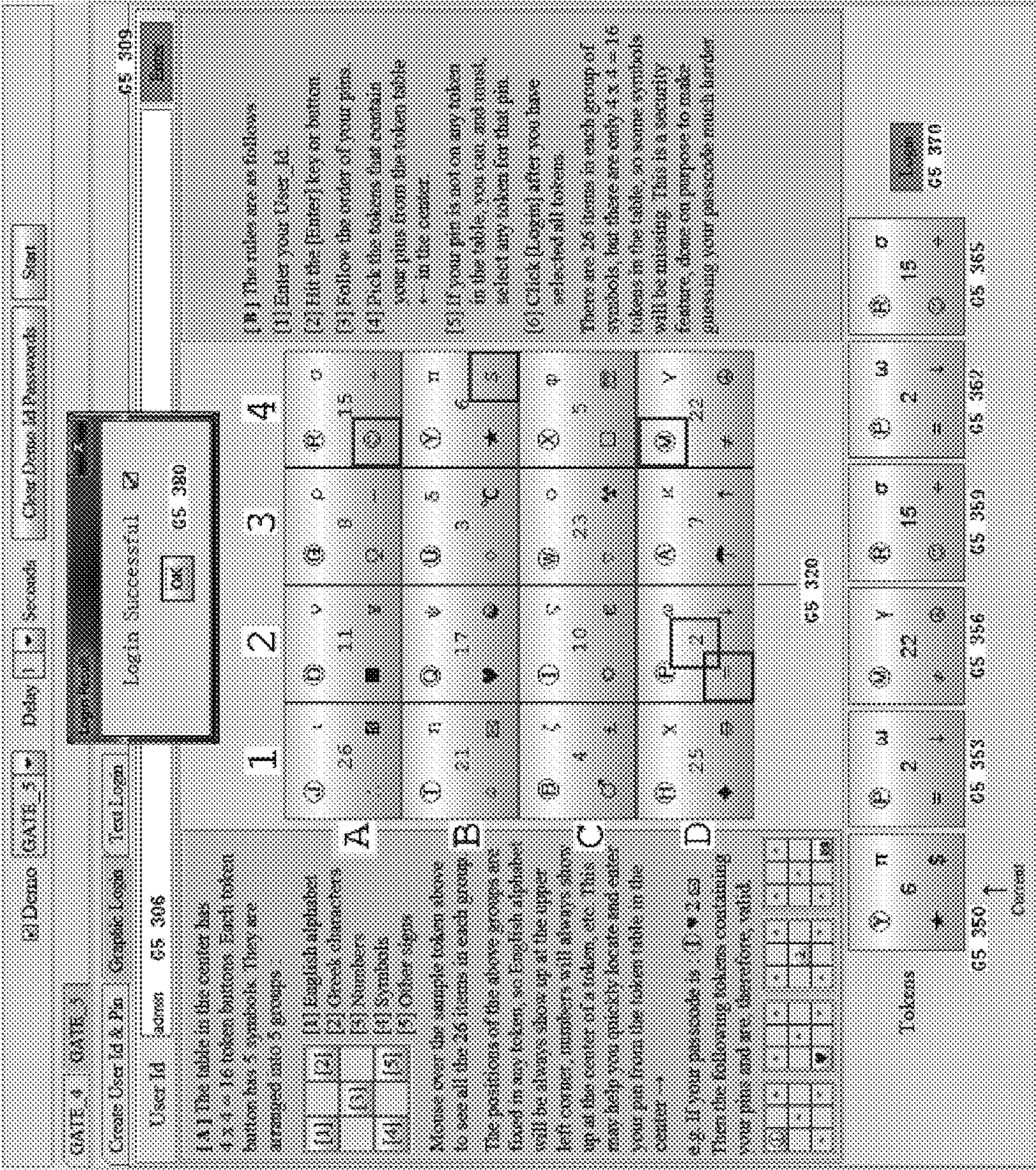
Fig. 12B GATE_5_Graphic_Login
