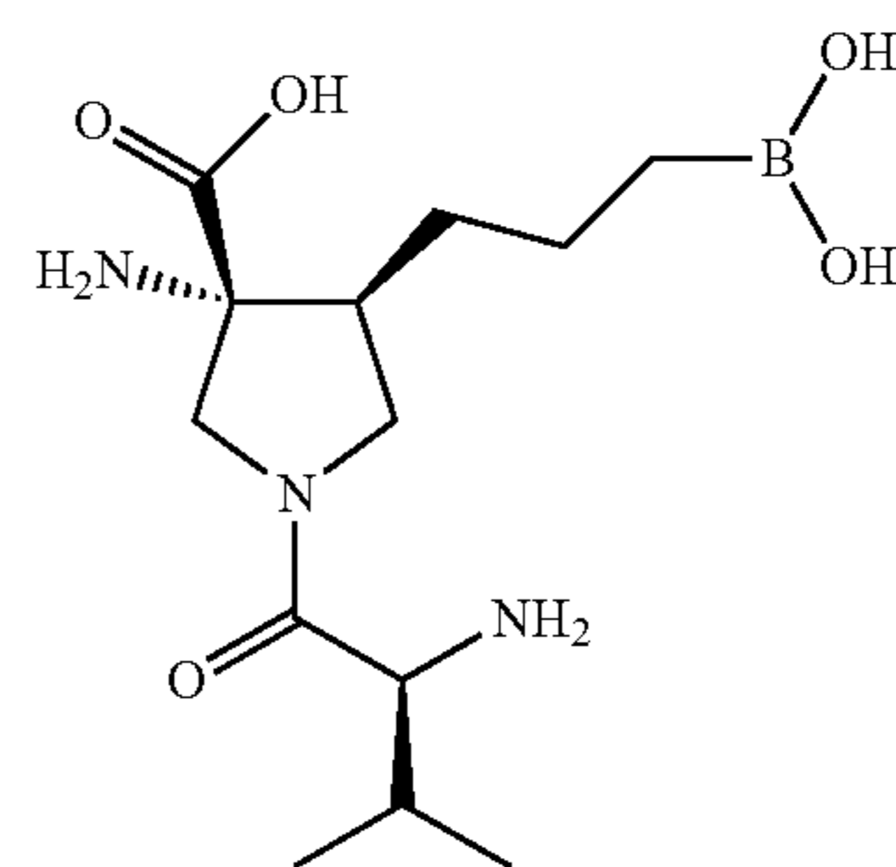
Valine AUC = 13701 IC 50 = 70 nM
