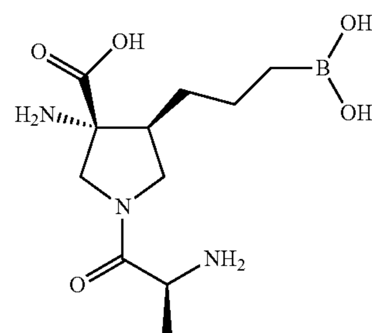
Alanine AUC = 13727 IC 50 = 93 nM
