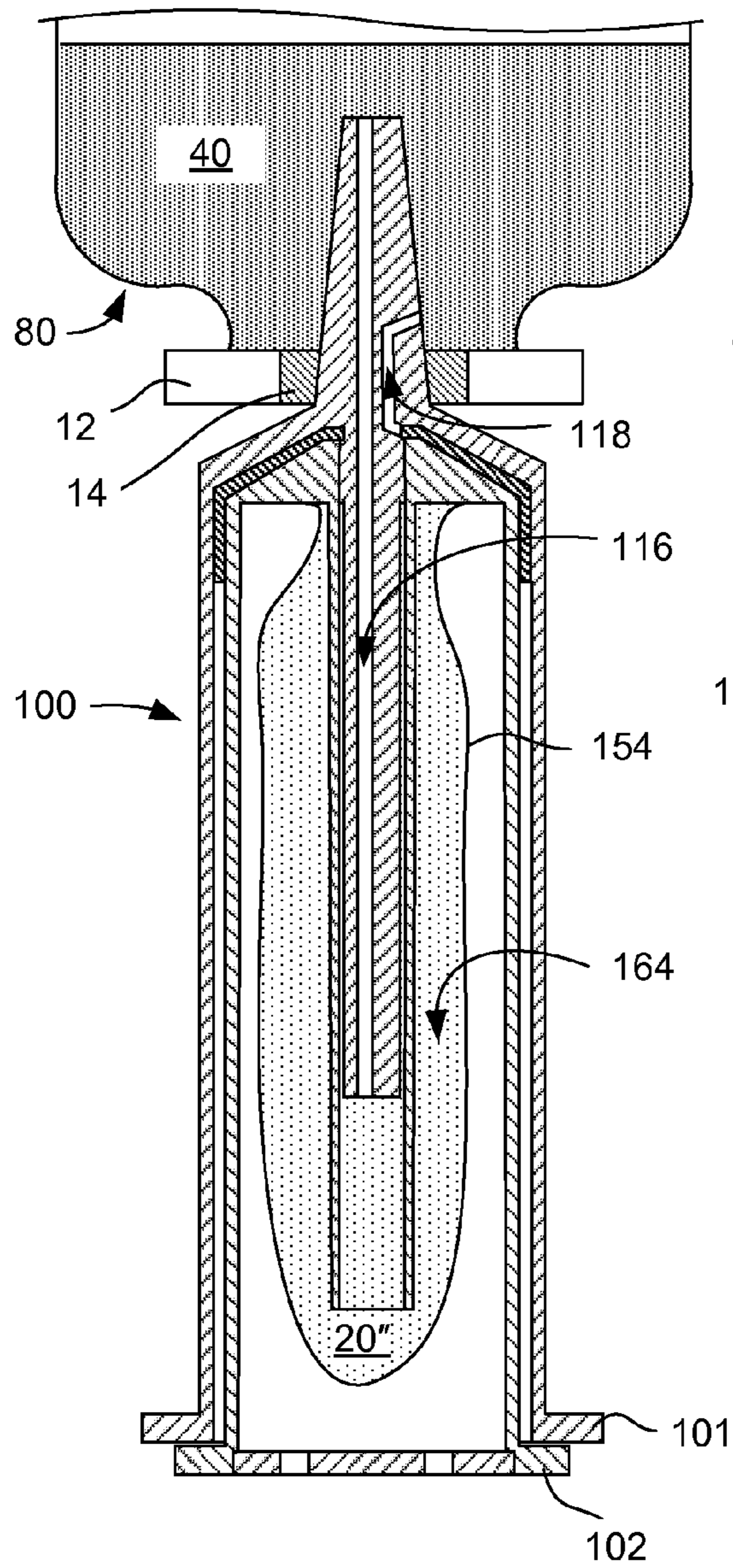
FIG. 3A
