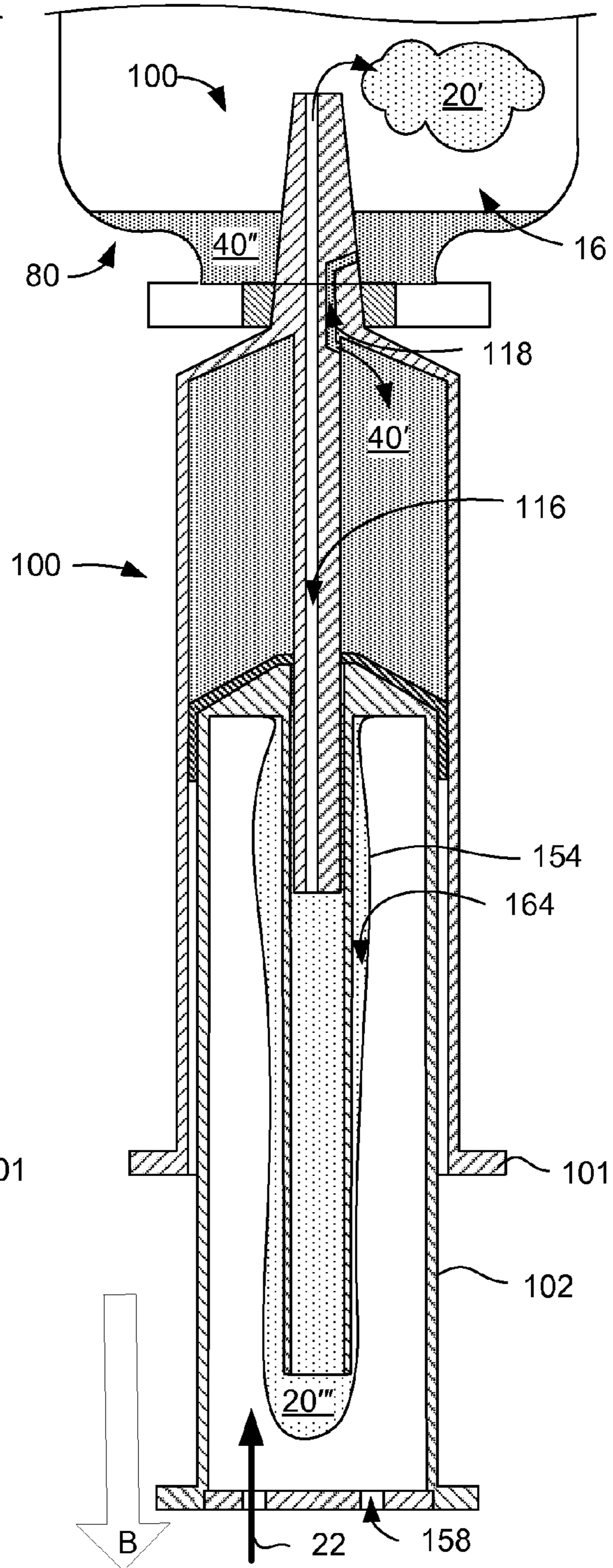
FIG. 3B
