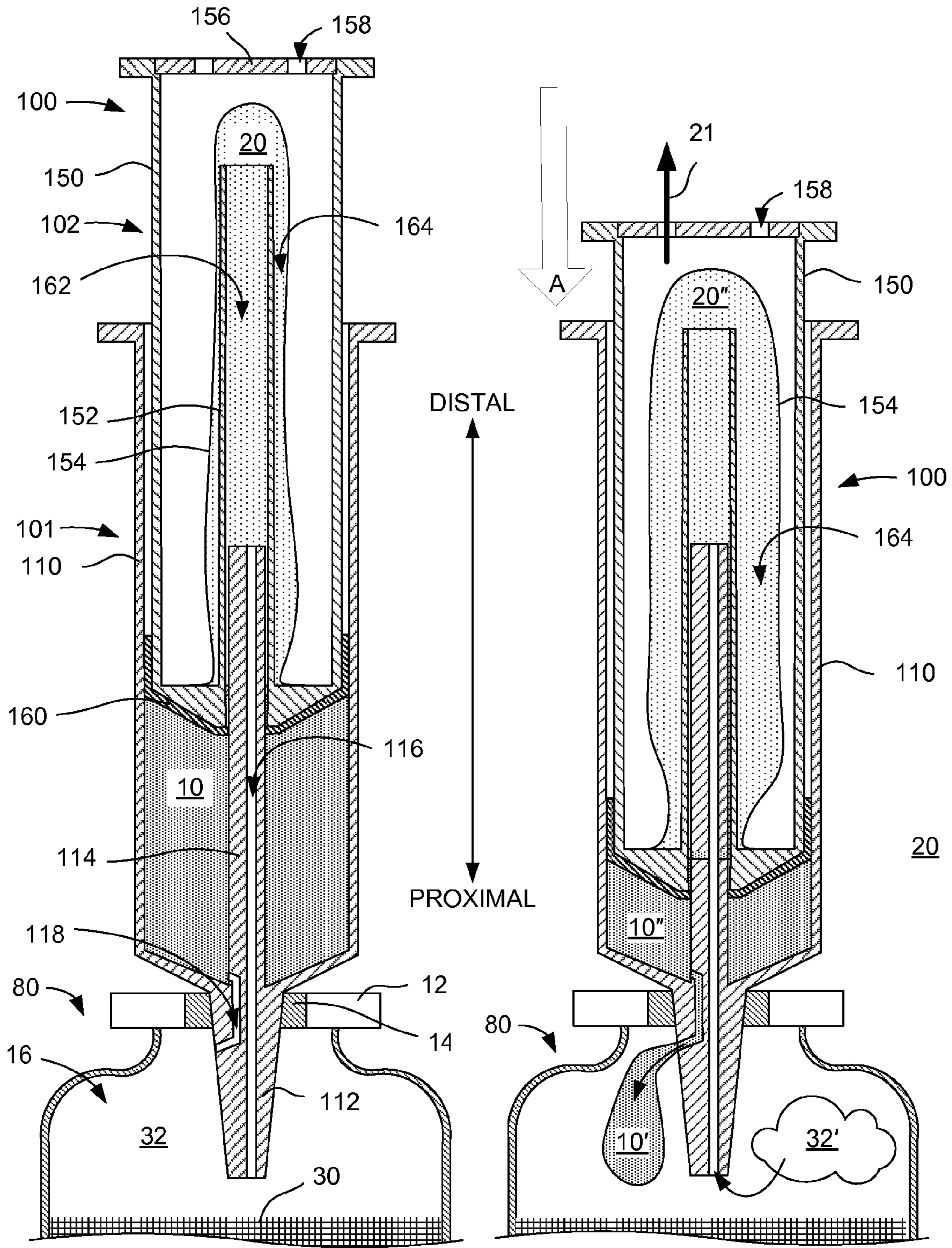
FIG. 2A
