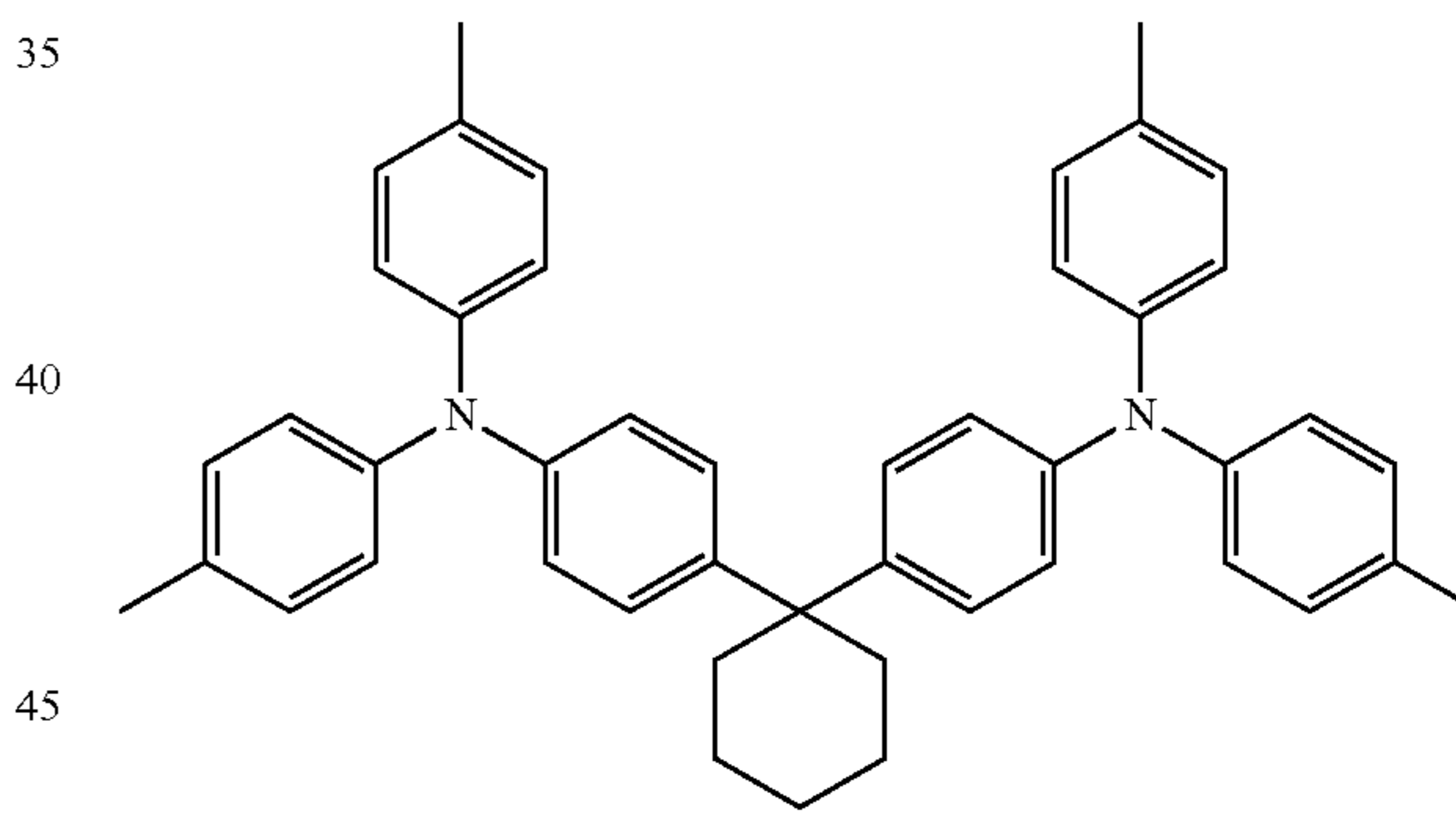
TAPC
