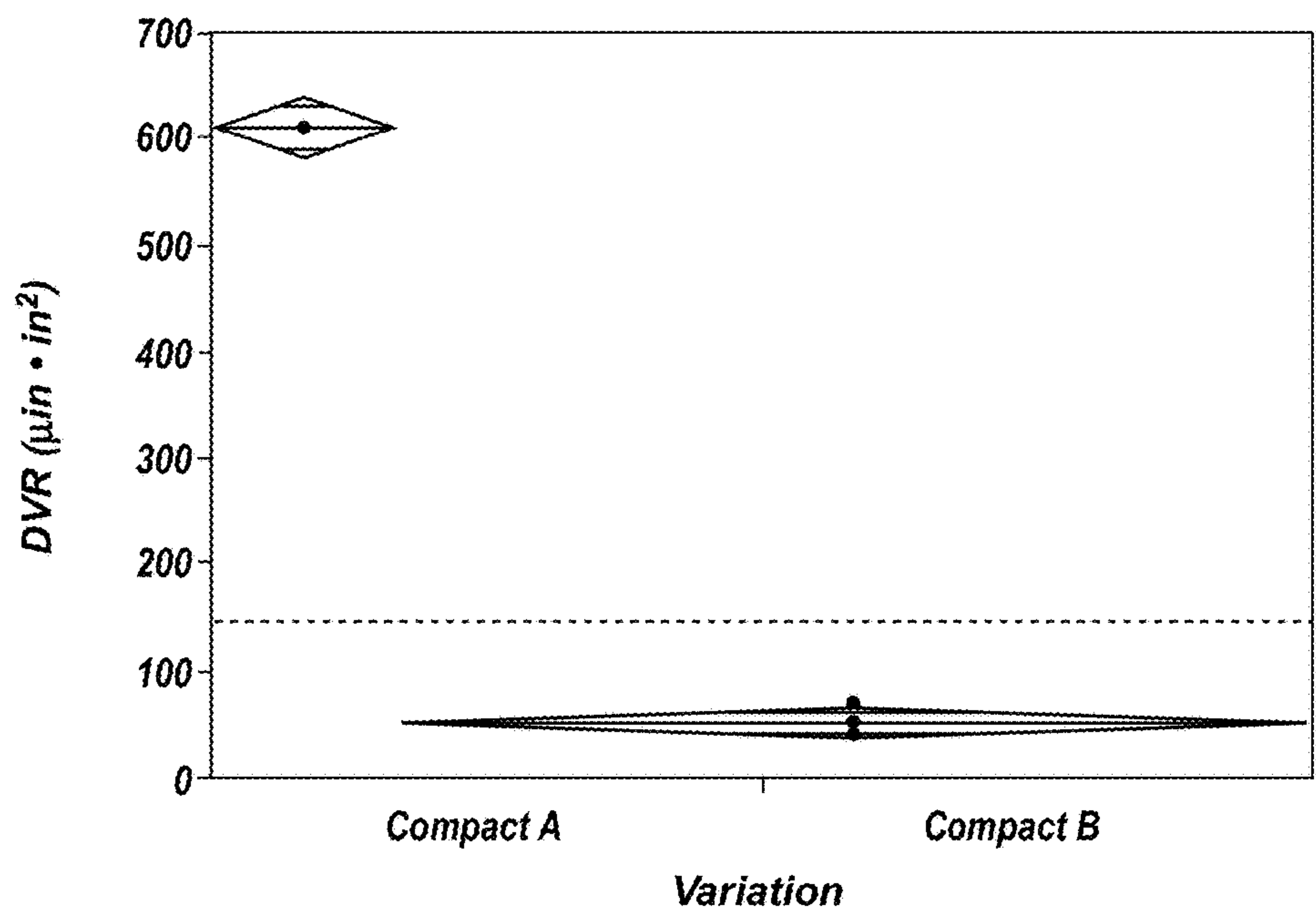
FIG. 5G
