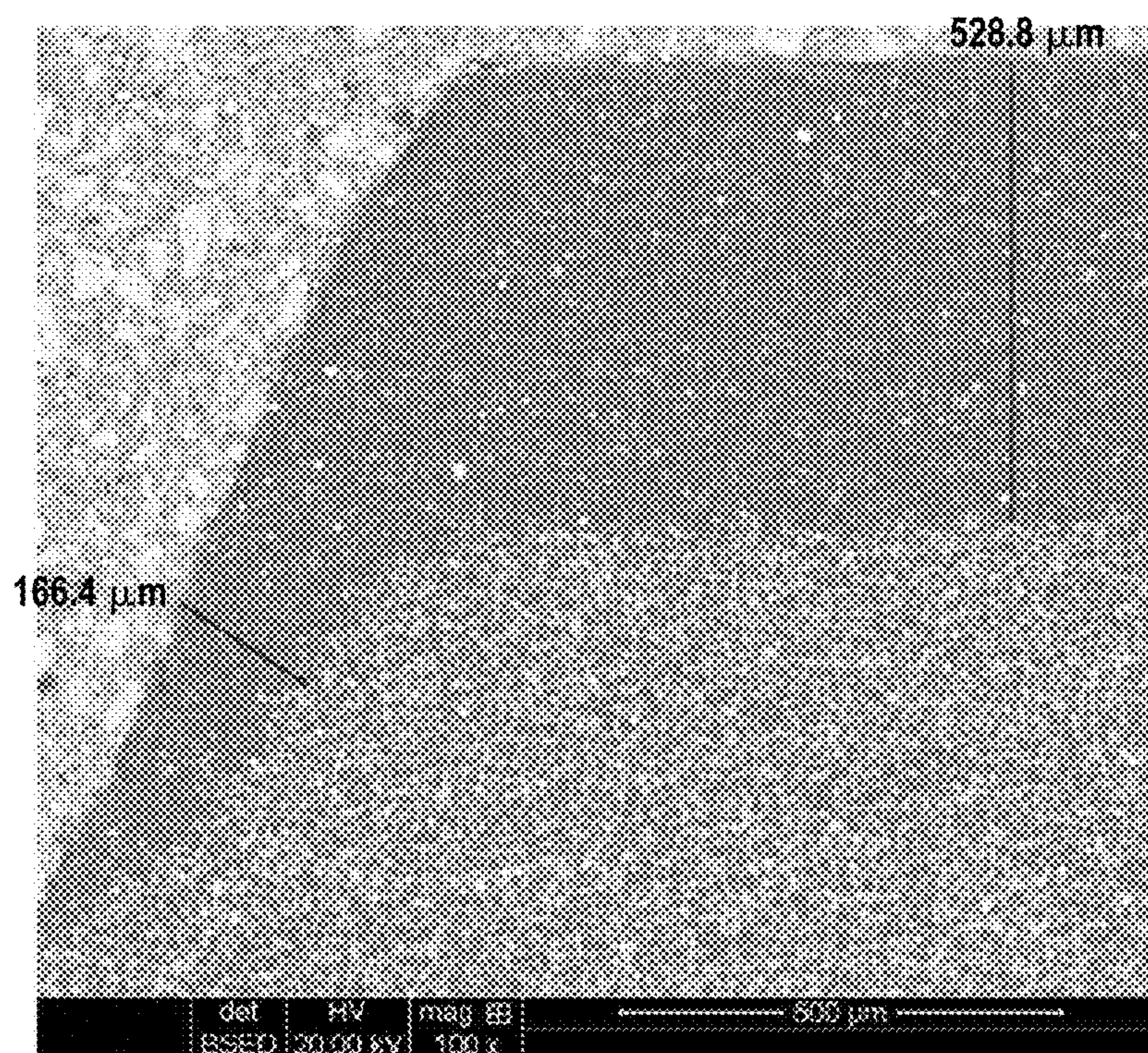
FIG. 4A
