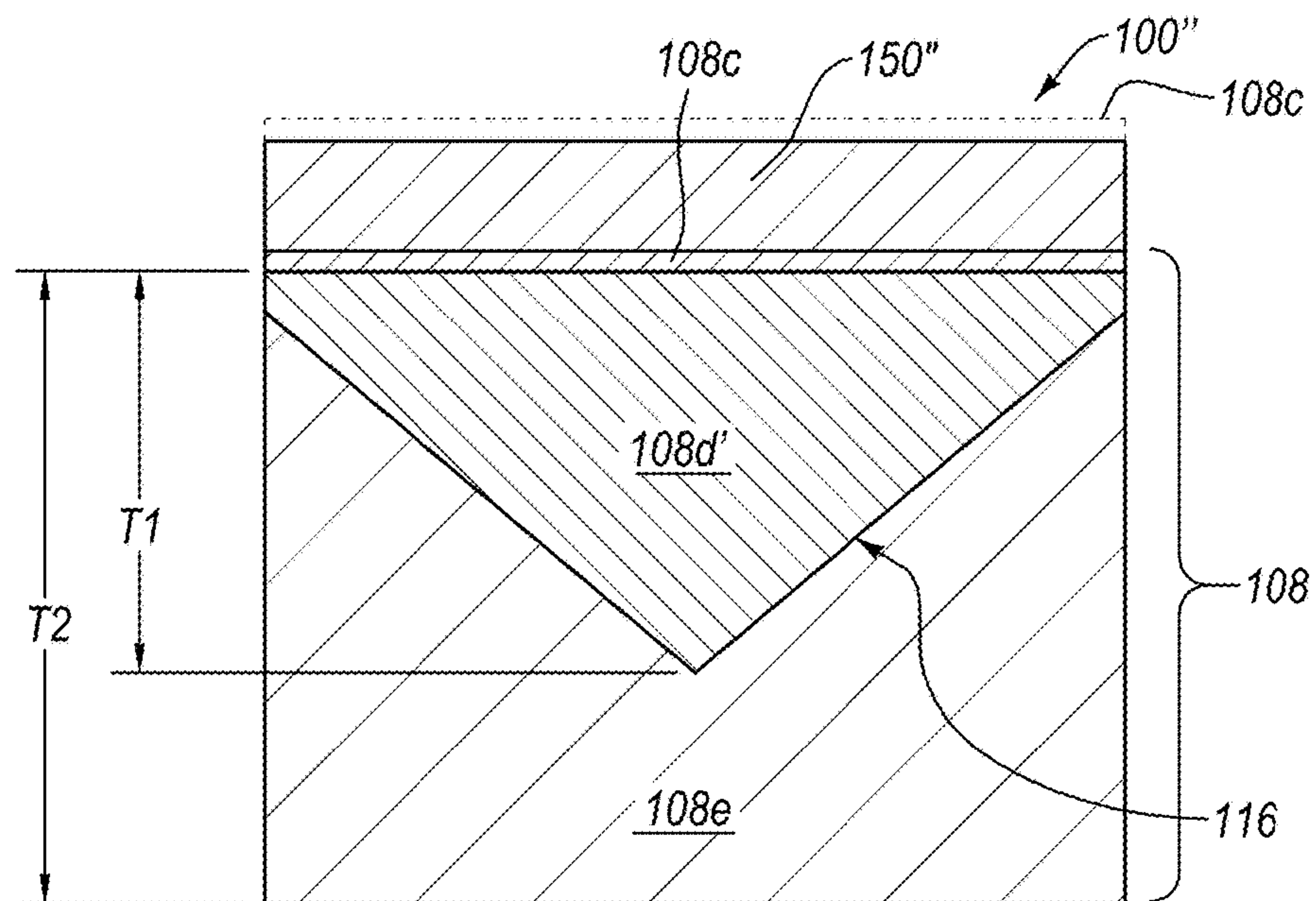
FIG. 3C
