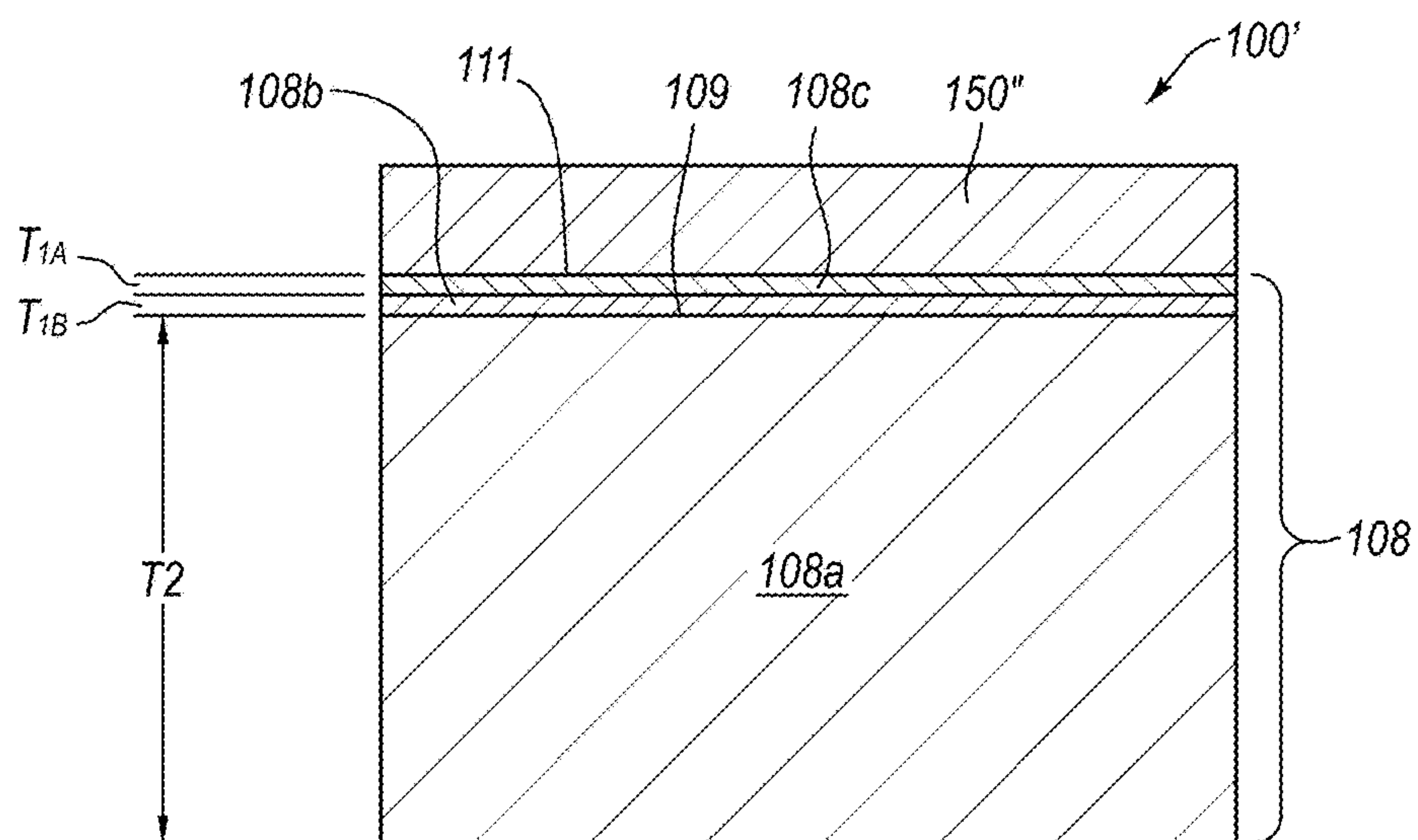
FIG. 3A
