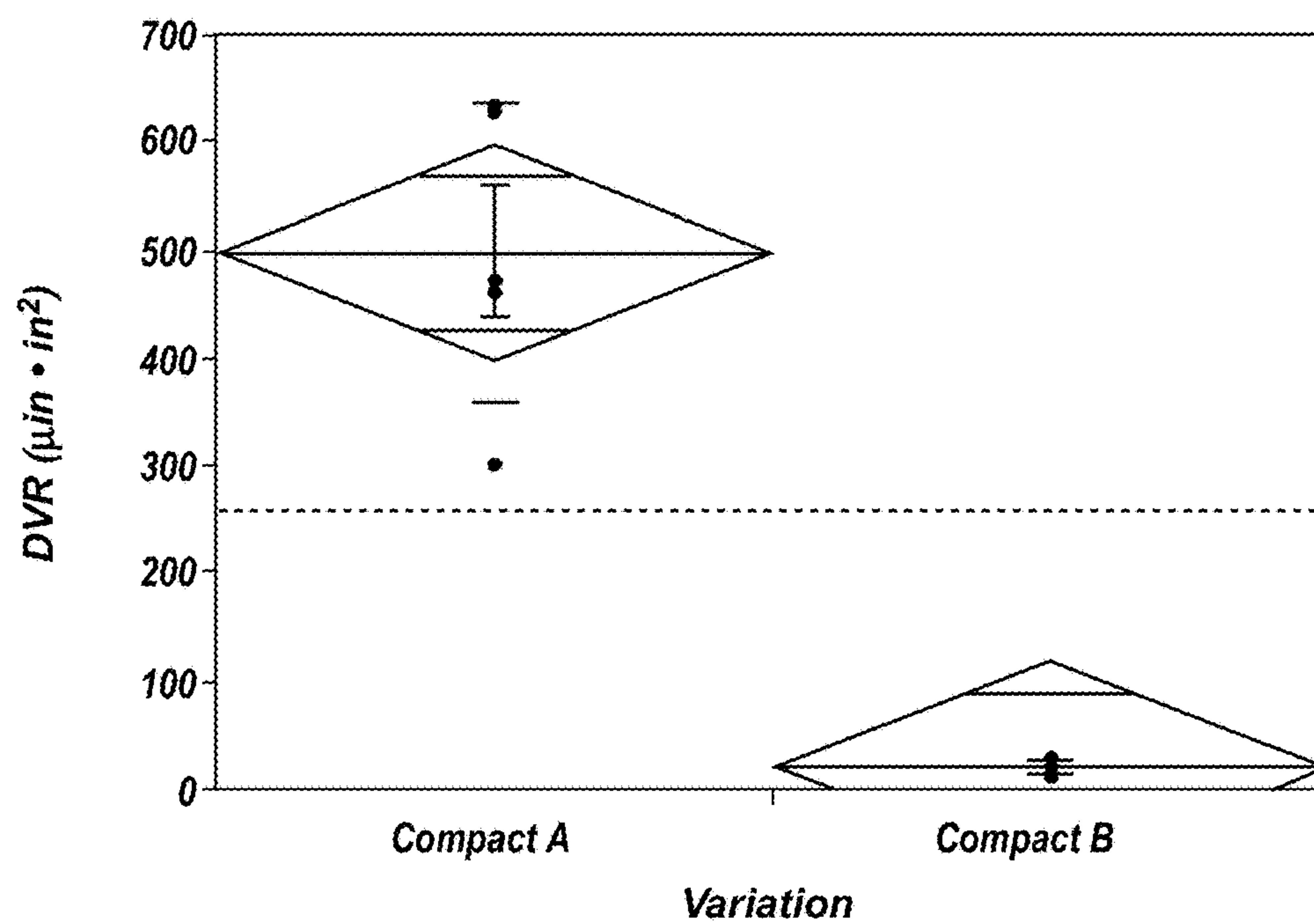
FIG. 5F
