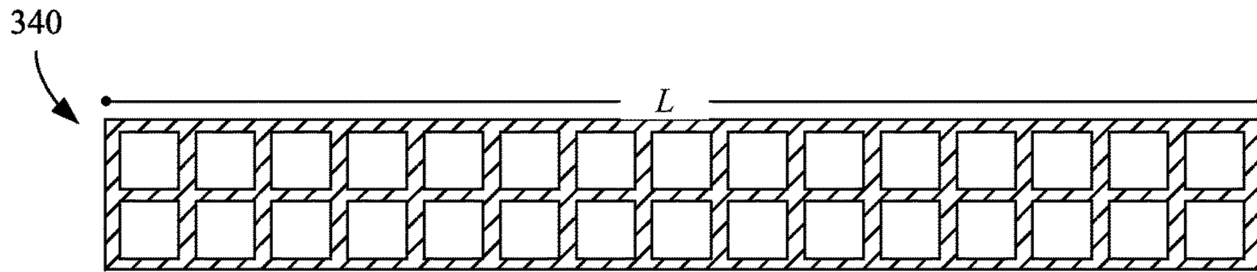
FIG. 3E
