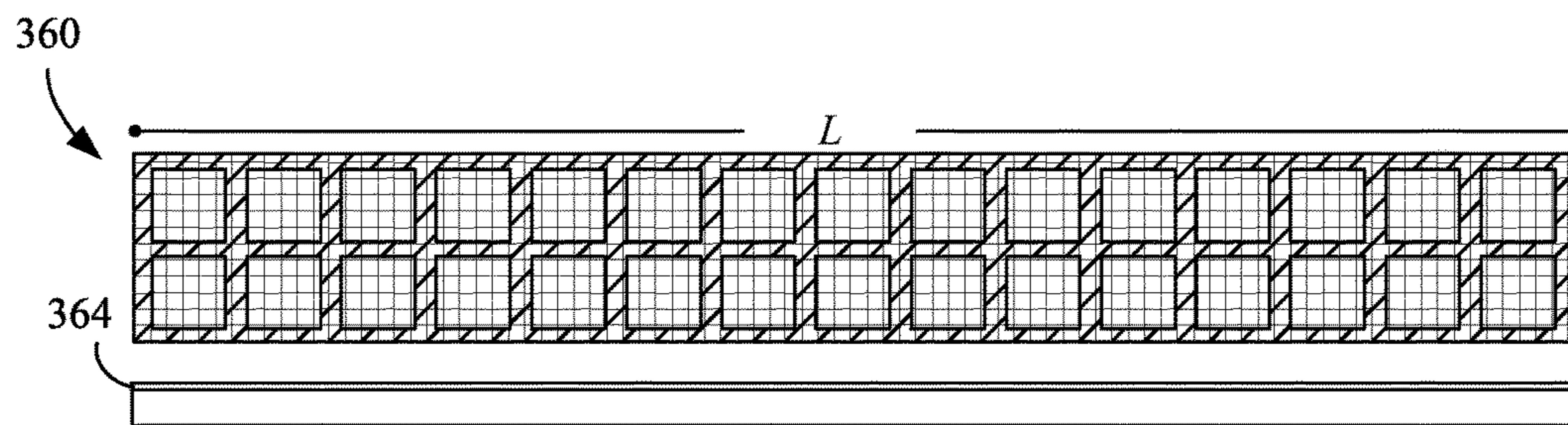
FIG. 3G
