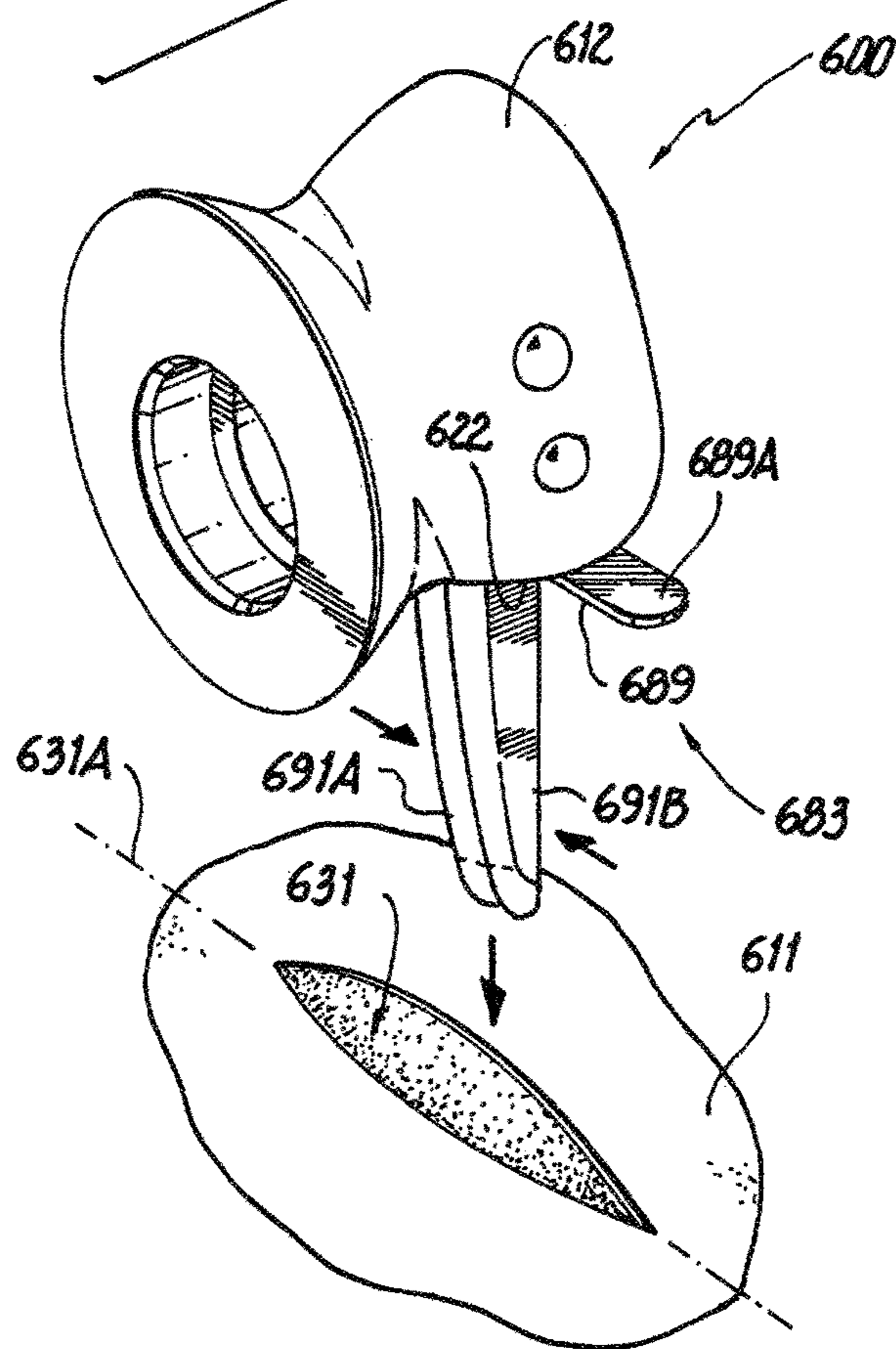
Fig. 12
