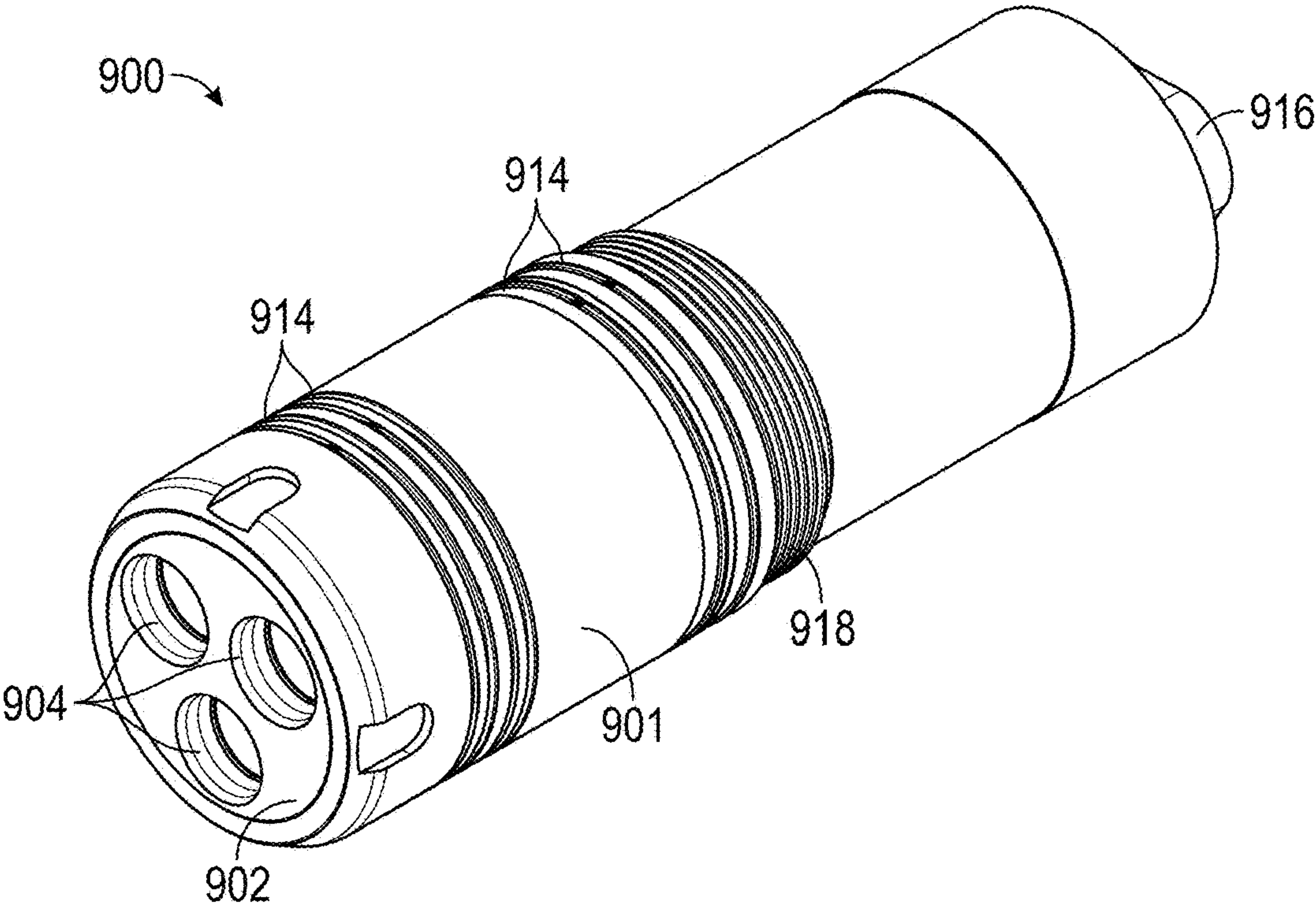
FIG. 9A
