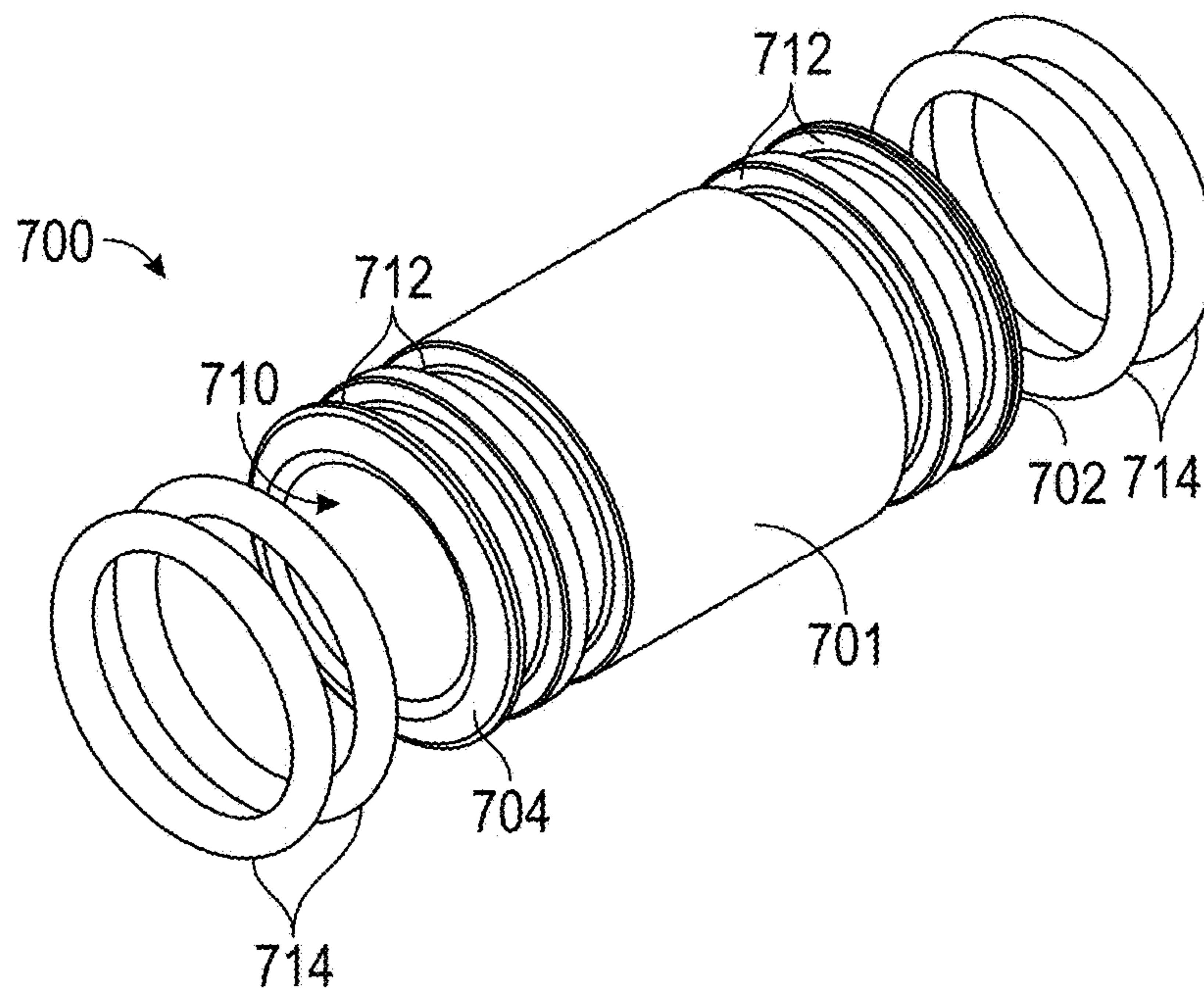
FIG. 7A
