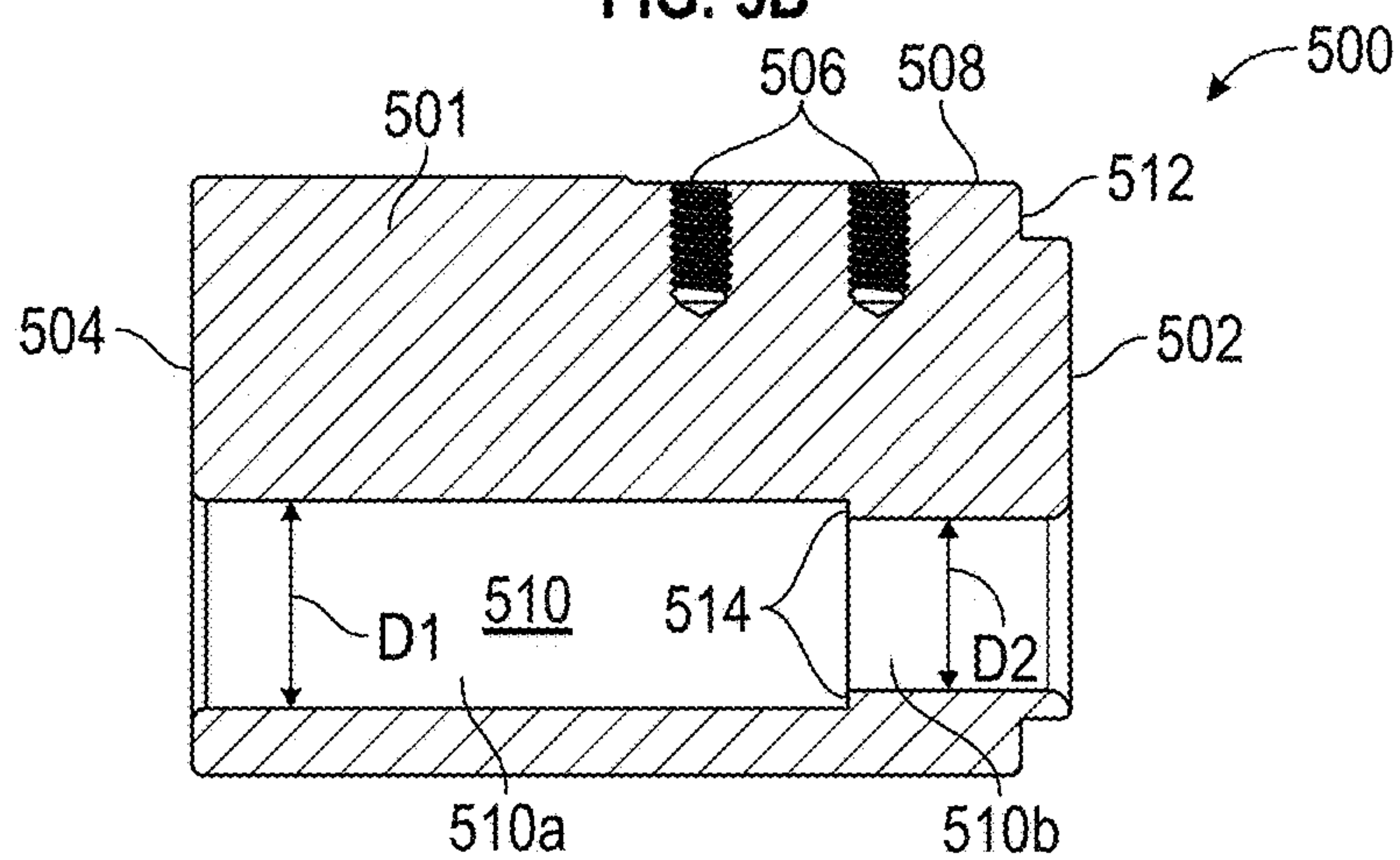
FIG. 5C
