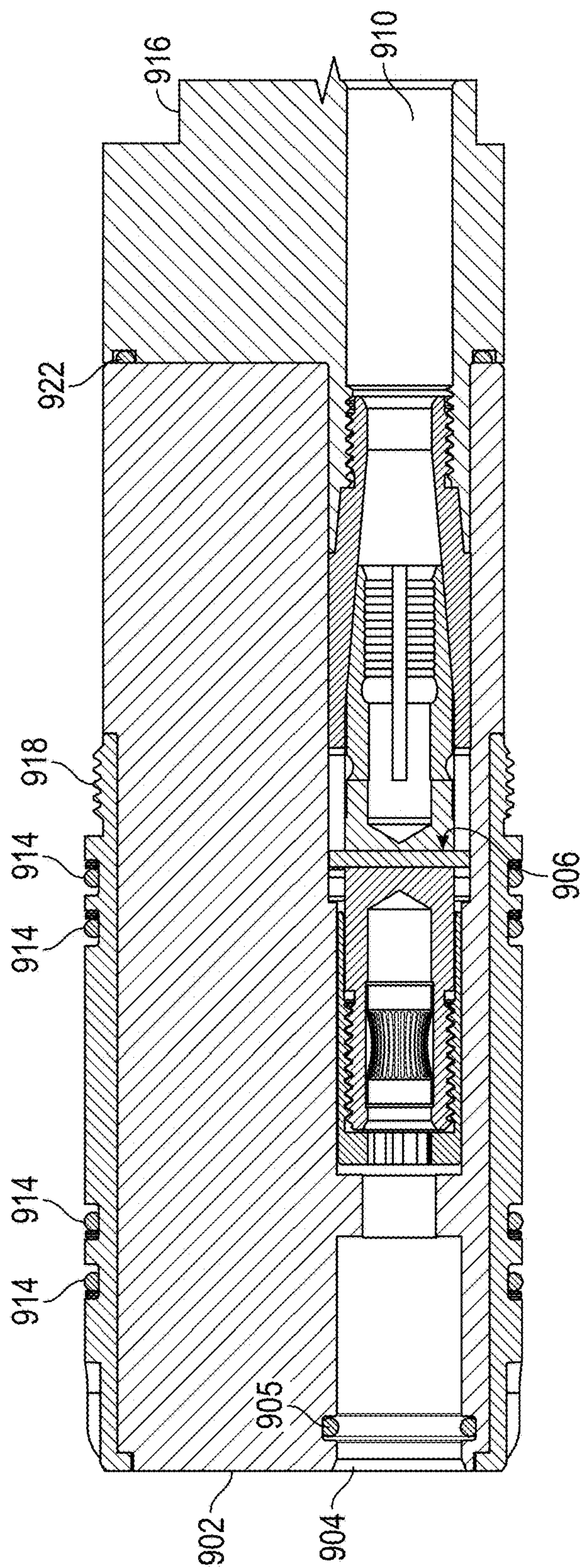
FIG. 9C
