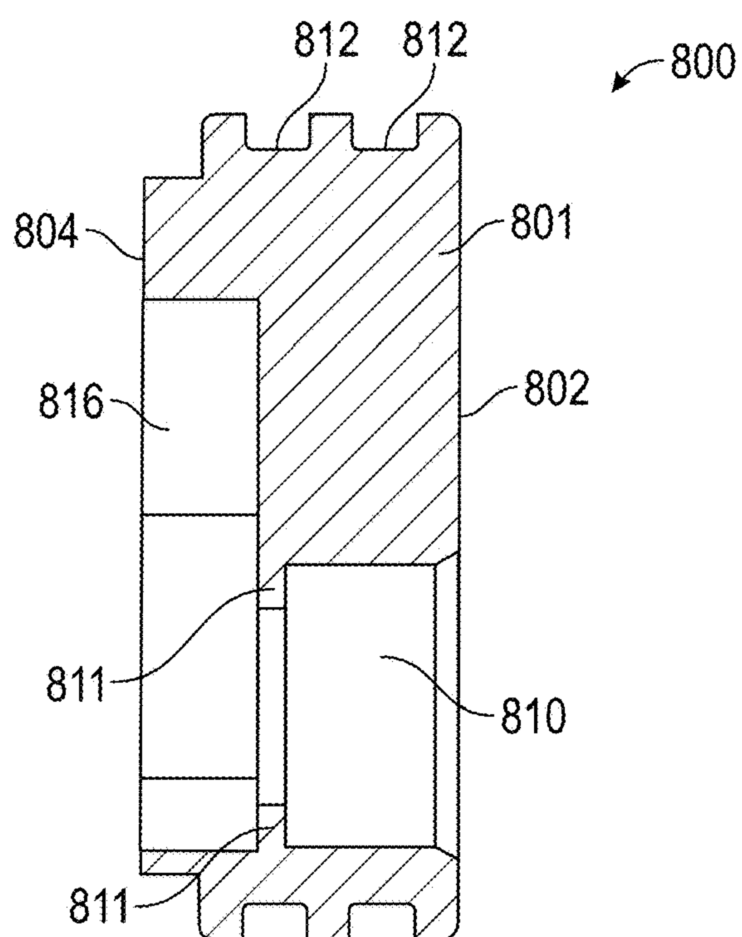
FIG. 8D
