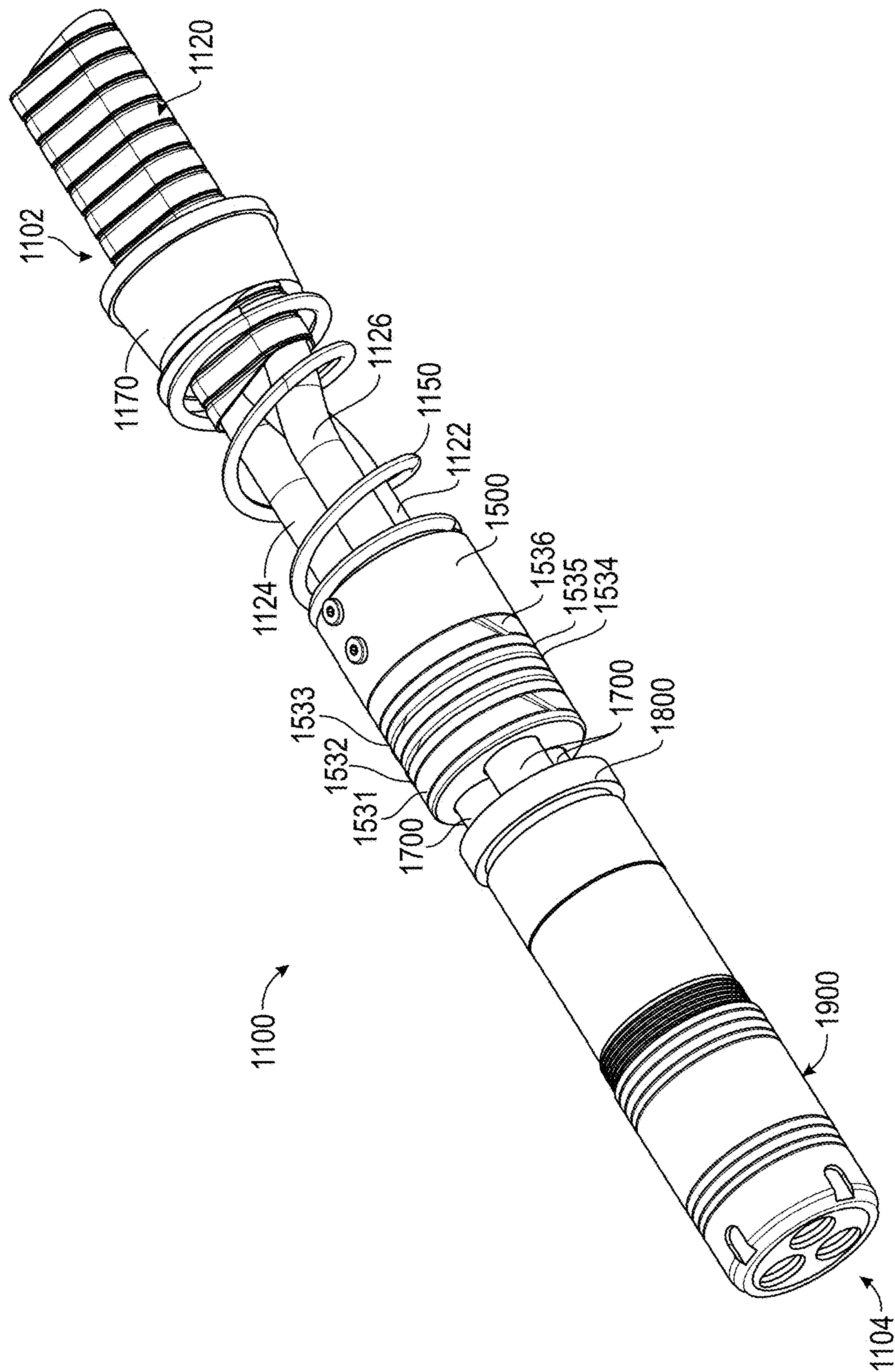
FIG. 11B
