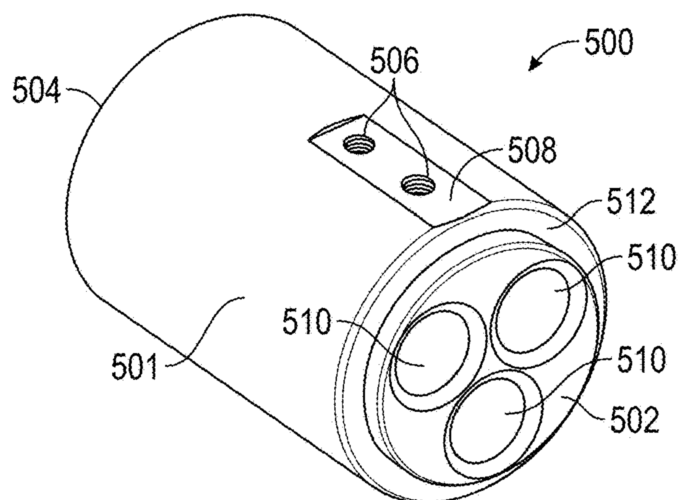
FIG. 5B
