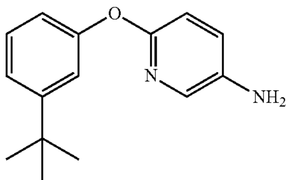
6-(3-(tert-butyl)phenoxy)pyridin-3-amine
