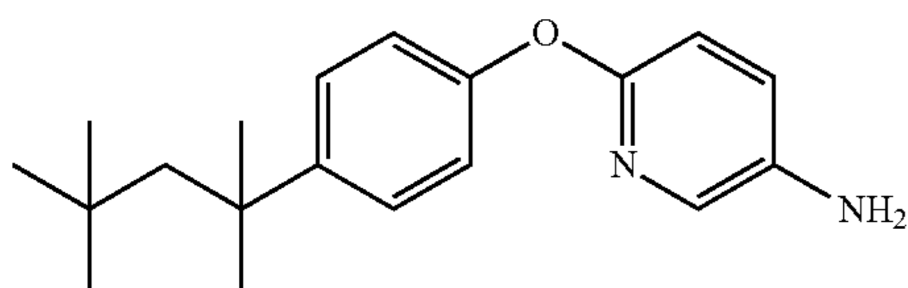
6-(4-(2,4,4-trimethylpentan-2-yl)phenoxy)pyridin-3-amine
