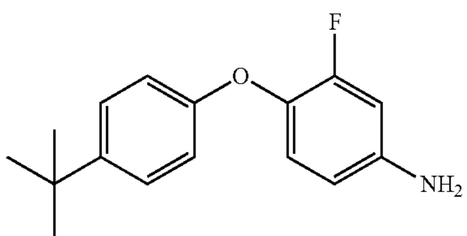
4-(4-(tert-butyl)phenoxy)-3-fluoroaniline
