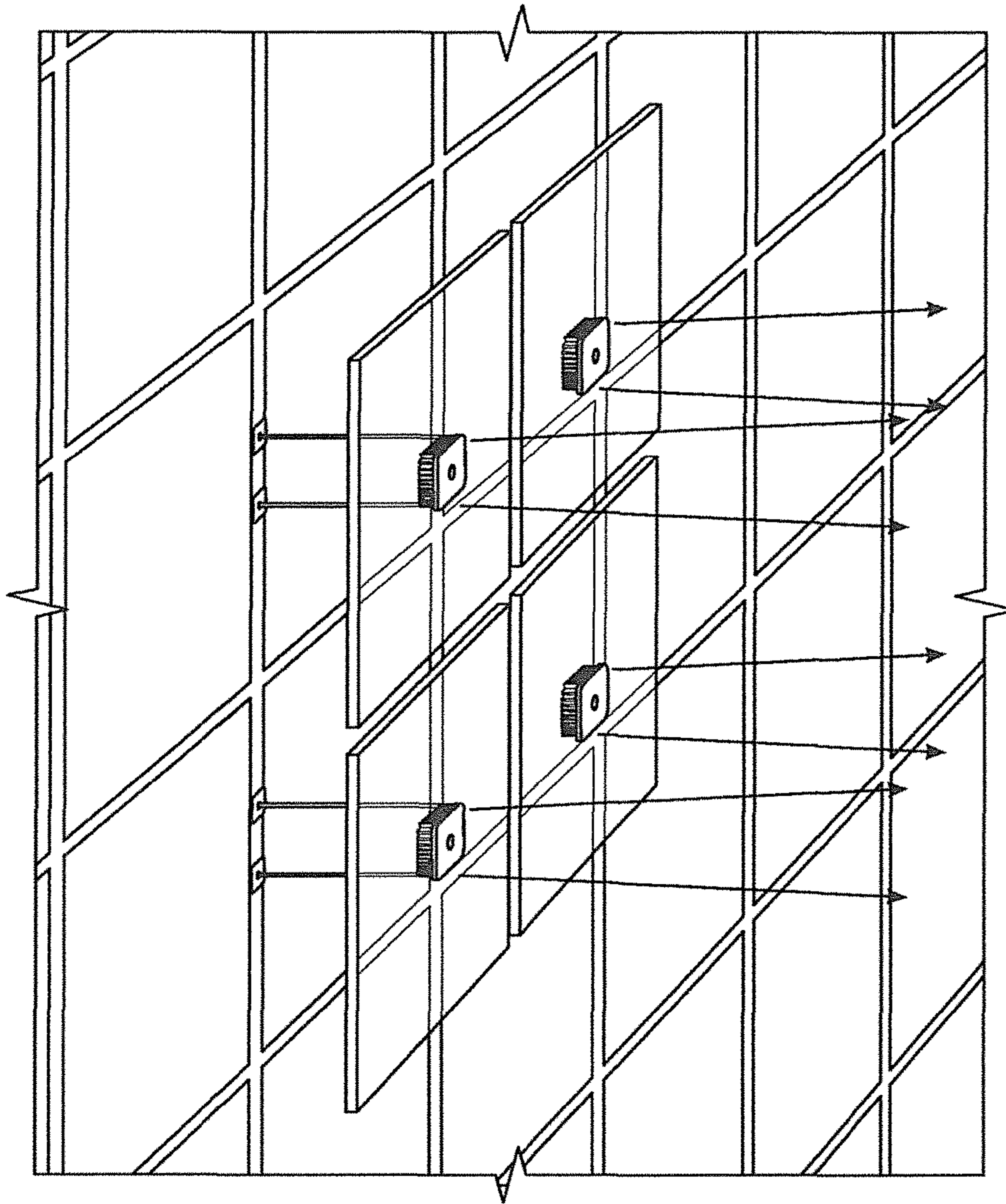
FIG. 6H
