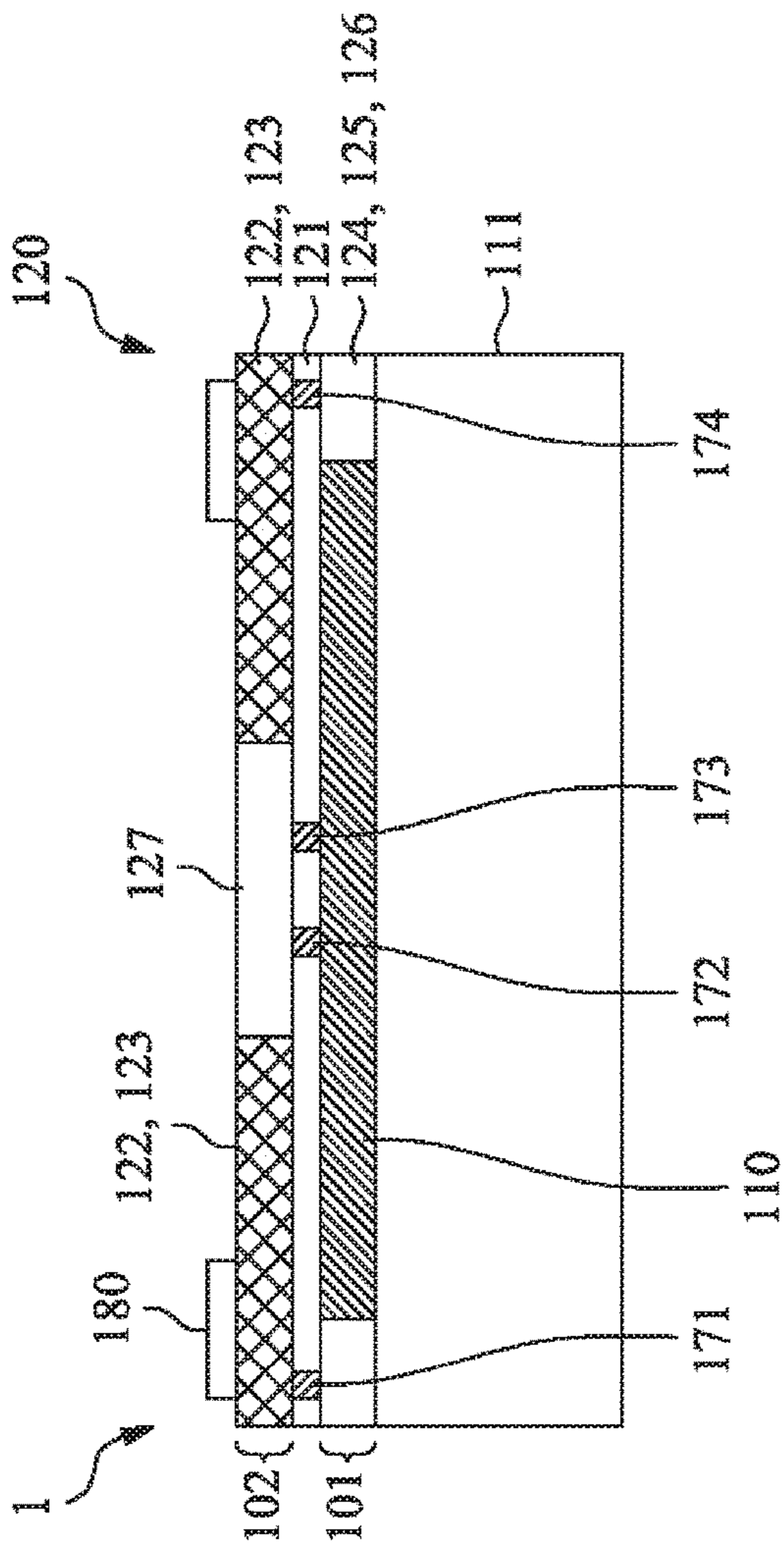
Fig. 1A
