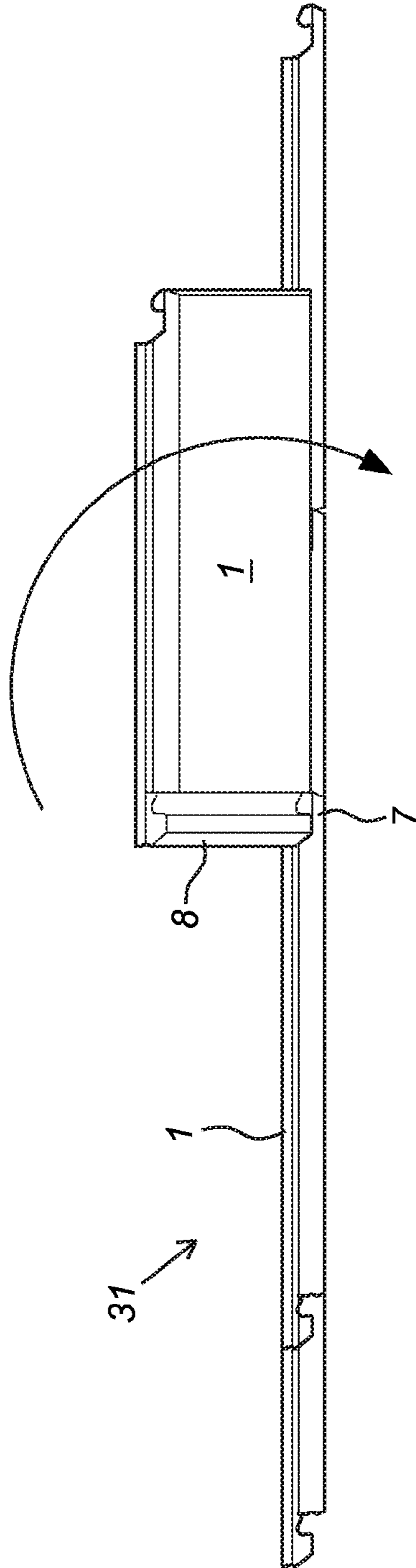
Fig. 4f
