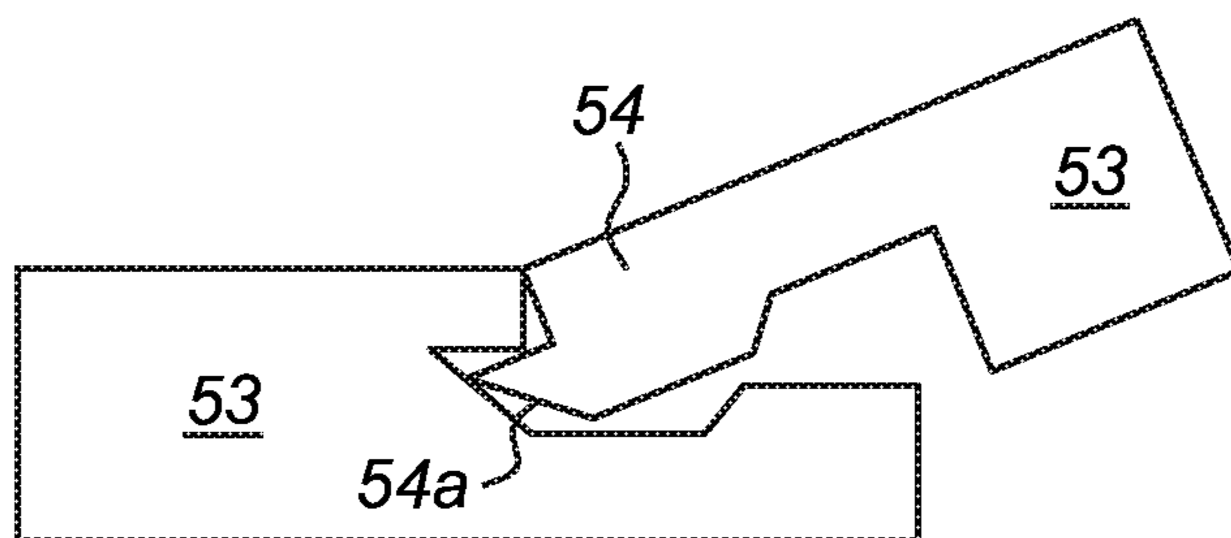
Fig. 5e
