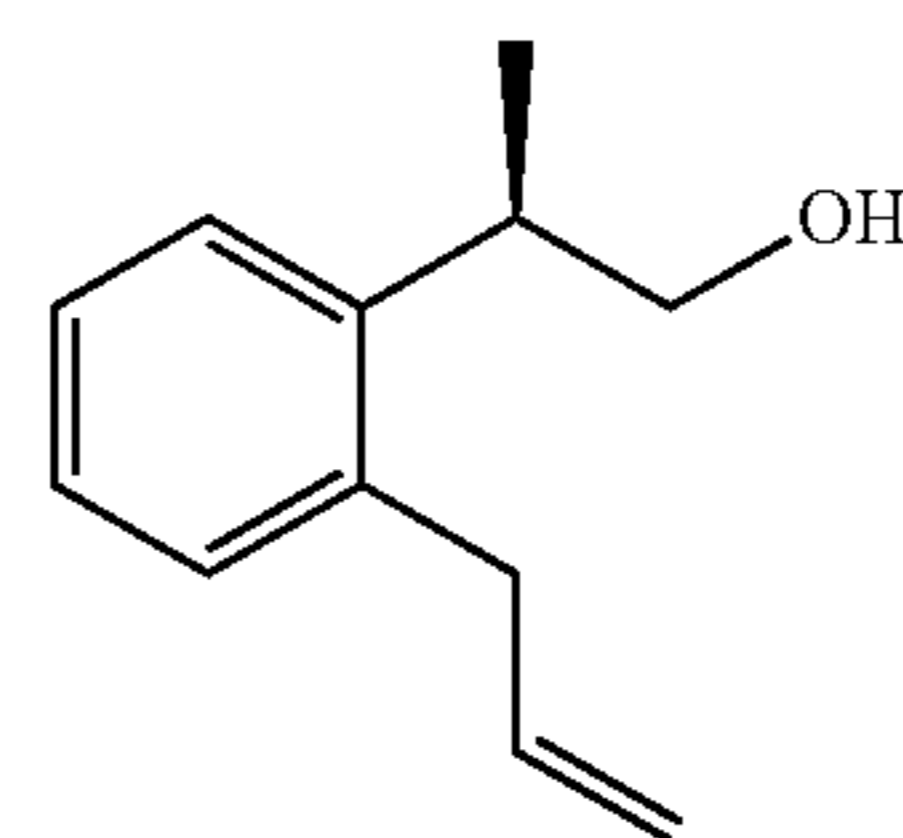
(R)-2-(2-allylphenyl)propan-1-ol (5)
