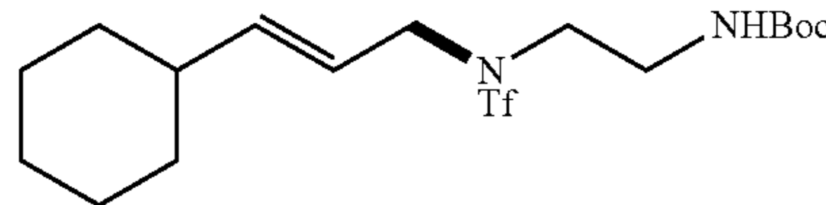
tert-Butyl-(E)-(2-((N-(3-cyclohexylallyl)-1,1,1-trifluoromethyl)sulfonamido)ethyl) carbamate (7)
