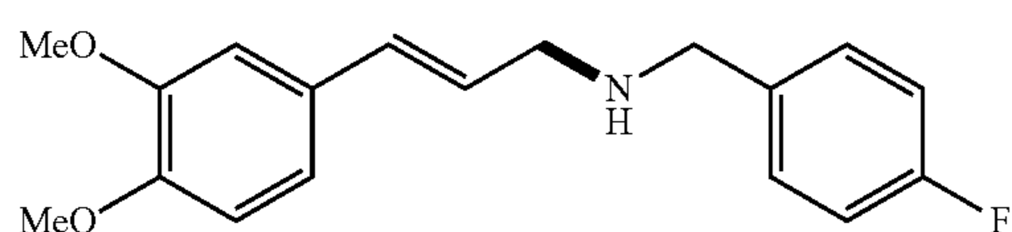
(E)-3-(3,4-dimethoxyphenyl)-N-(4-fluorobenzyl)prop-2-en-1-amine (51)
