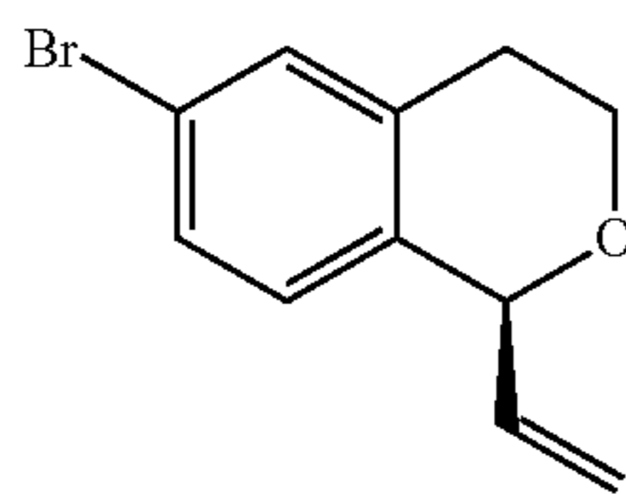
(S)-6-bromo-1-vinylisochromane (2e)
