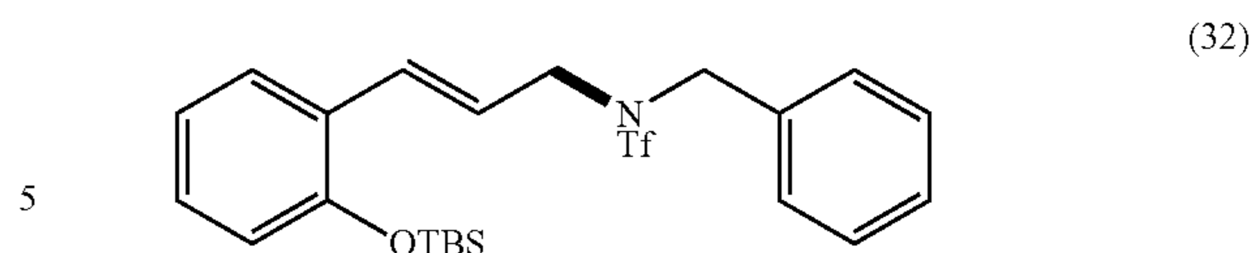
(E)-N-benzyl-N-(3-(2-((tert-butyl)dimethylsilyloxy)phenyl)allyl)-1,1,1-trifluoromethanesulfonamide (32)
