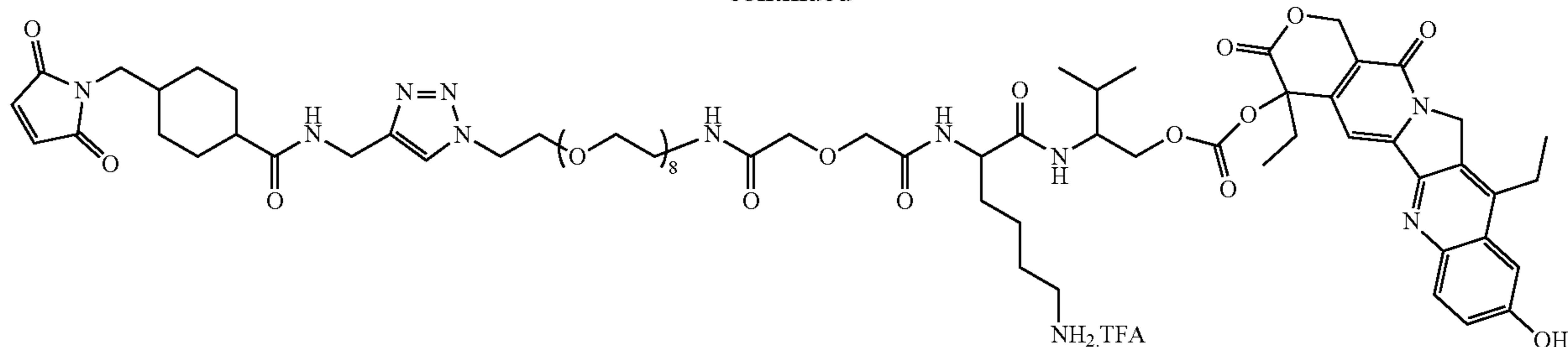
CL7-SN-38
