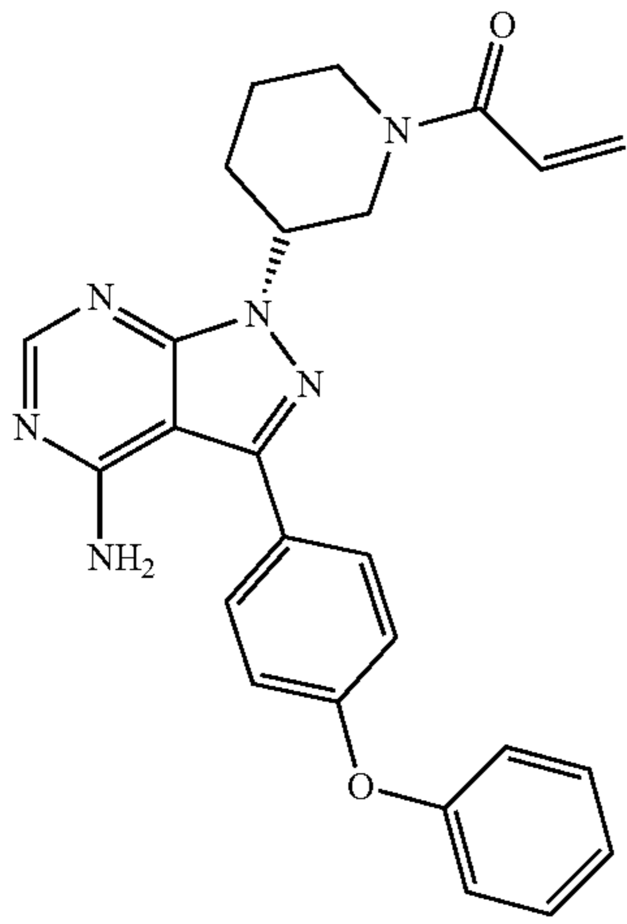
Ibrutinib
