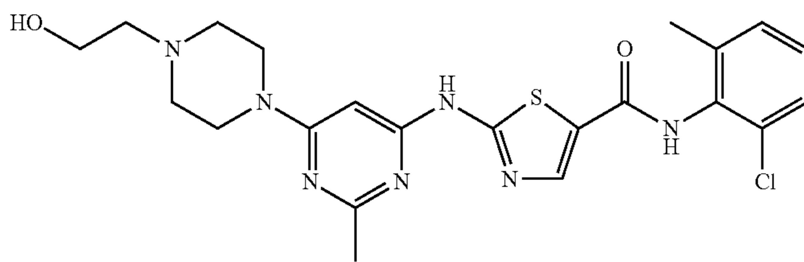
Dasatinib
