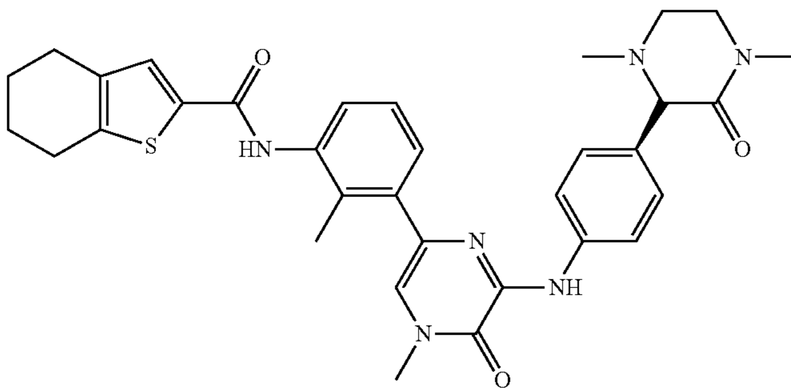
GDC-0834
