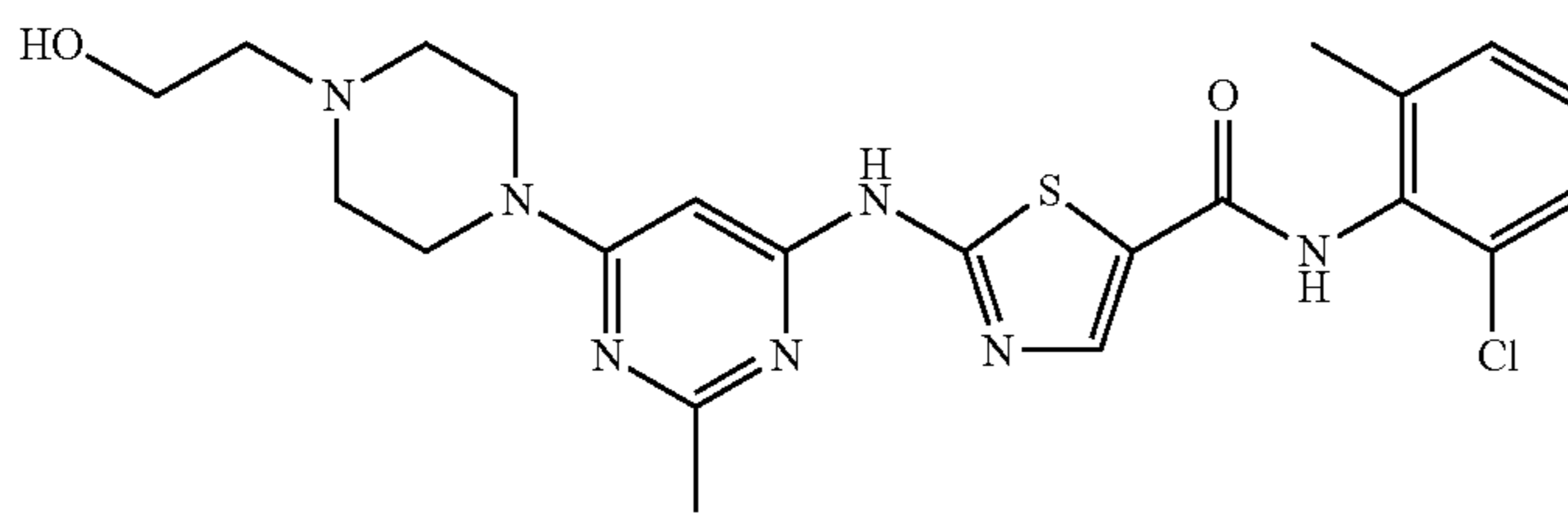
Dasatinib
