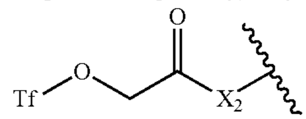
2-(((trifluoromethyl)-sulfonyl)oxy)acetyl
