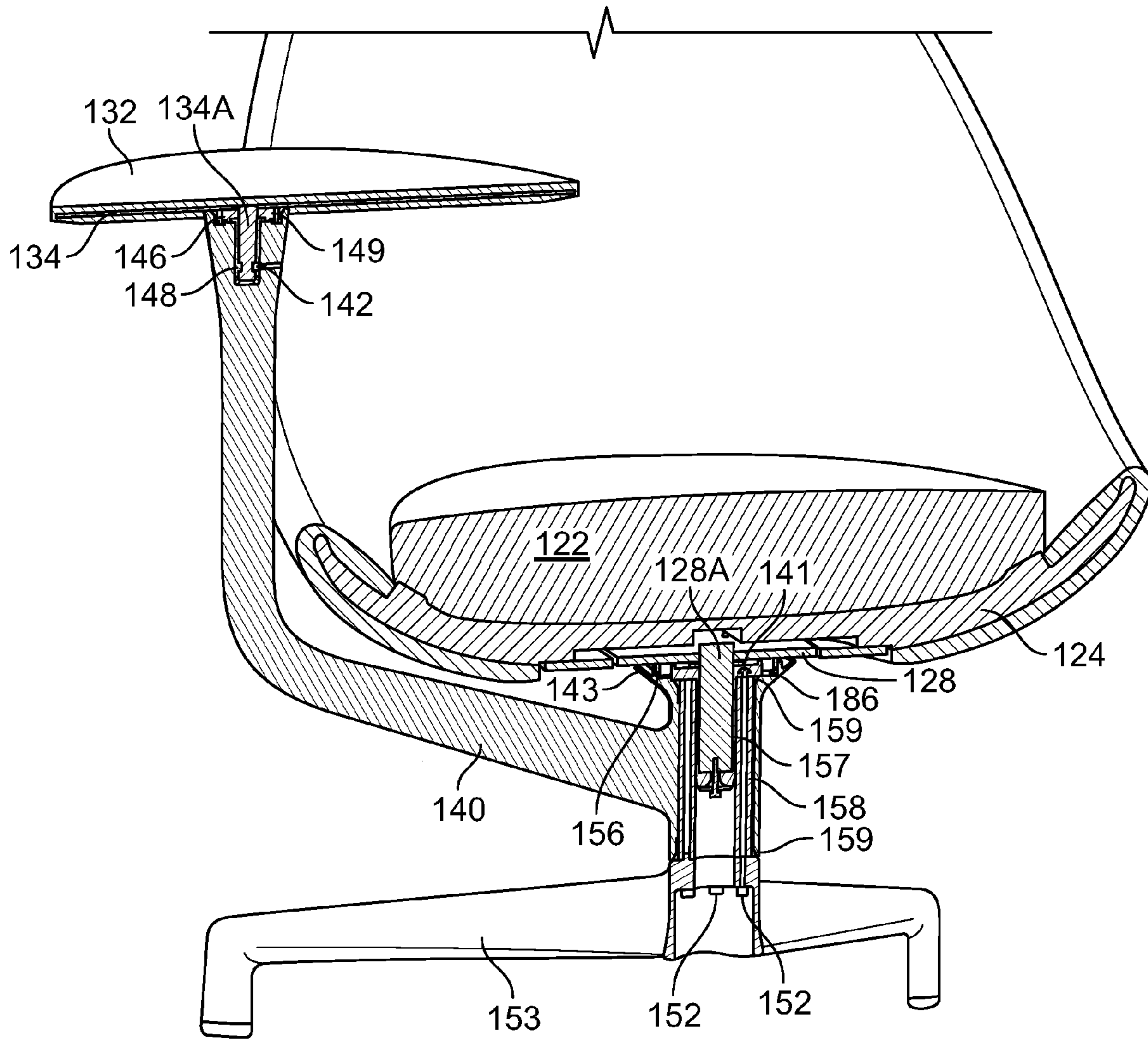
FIG. 10
