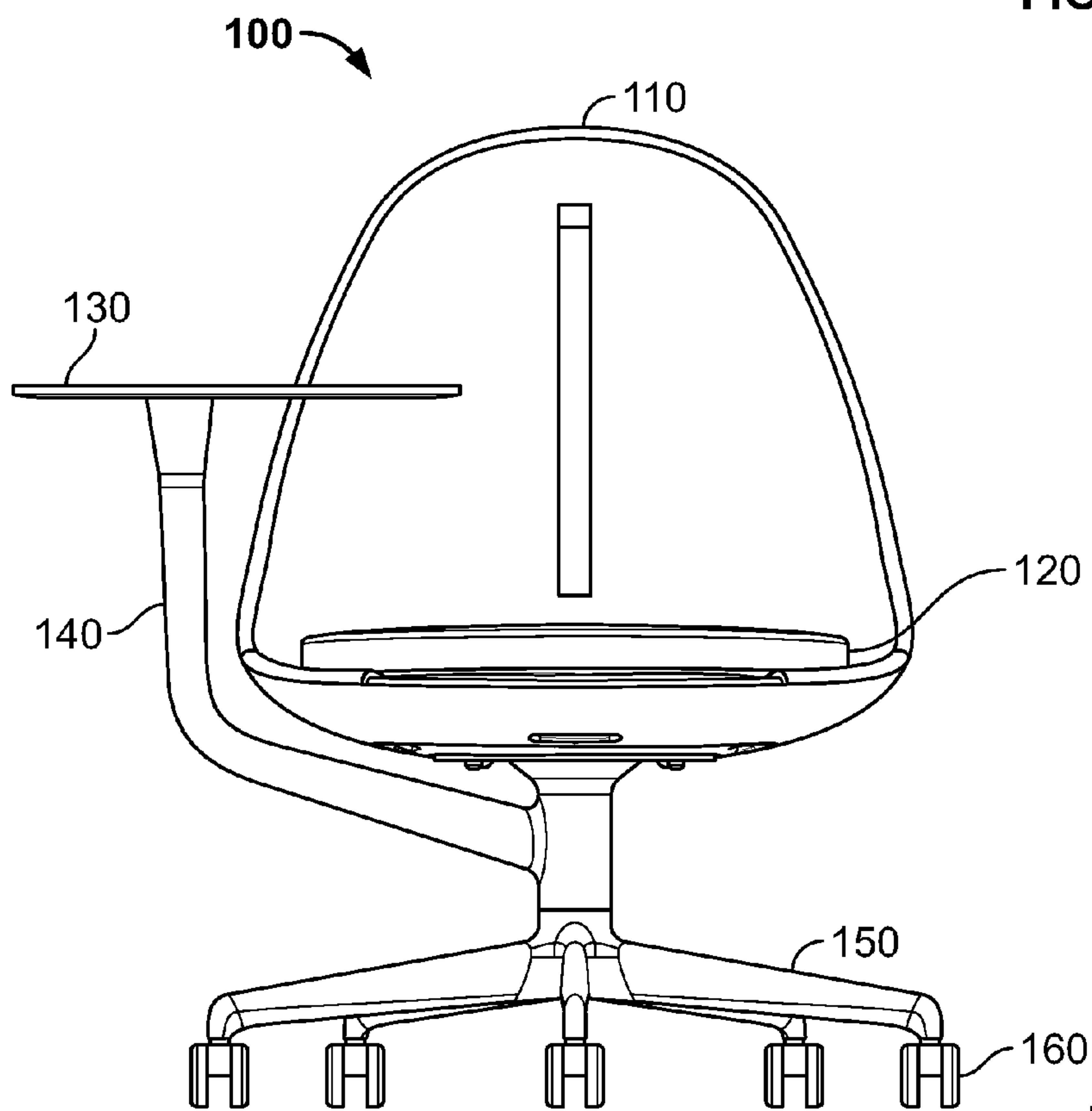
FIG. 1A
