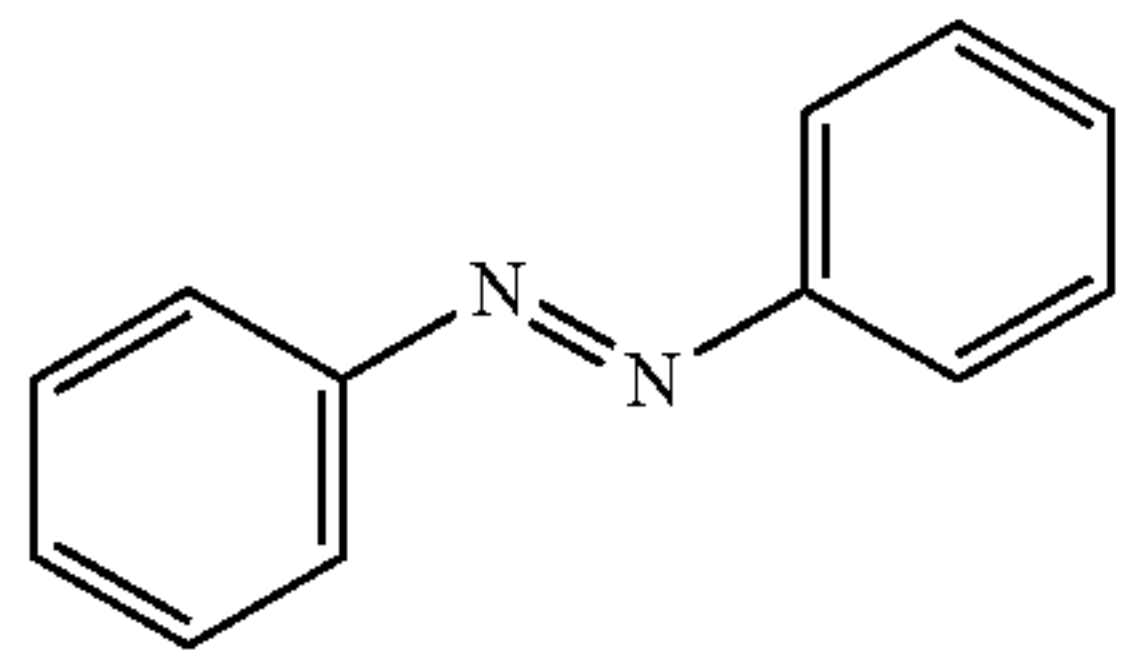
(E)-diphenyldiazene, (E)-Azobenzene
