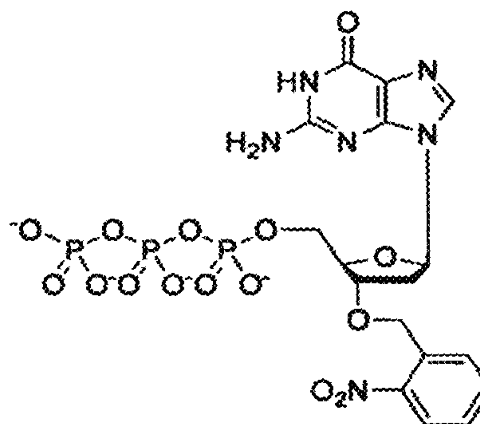
3'-O-(2-Nitrobenzyl)-dGTP
