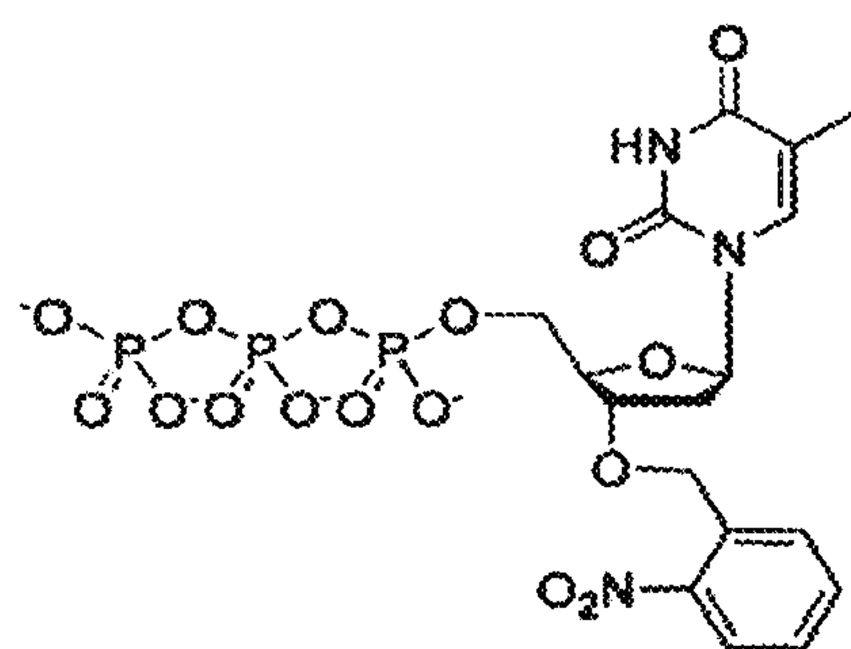
3'-O-(2-Nitrobenzyl)-dTTP
