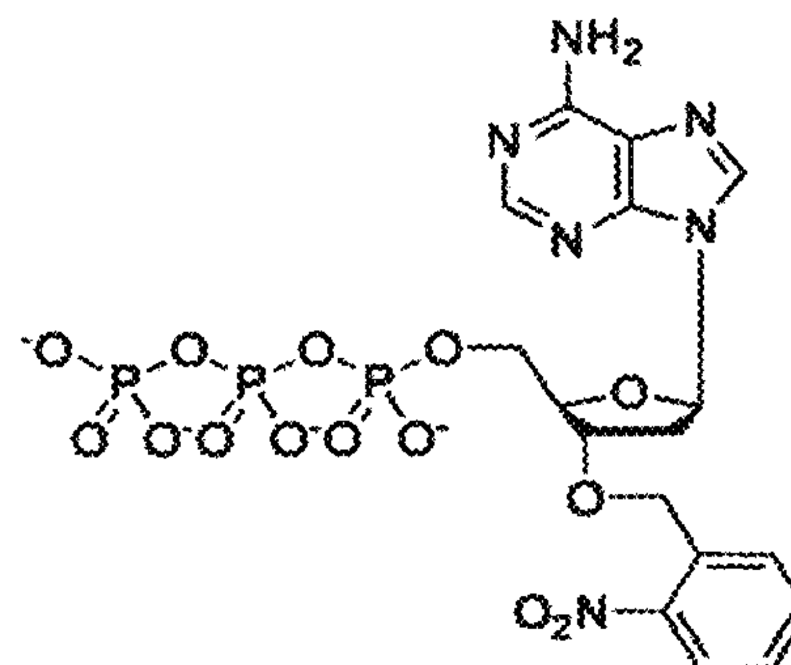
3'-O-(2-Nitrobenzyl)-dATP
