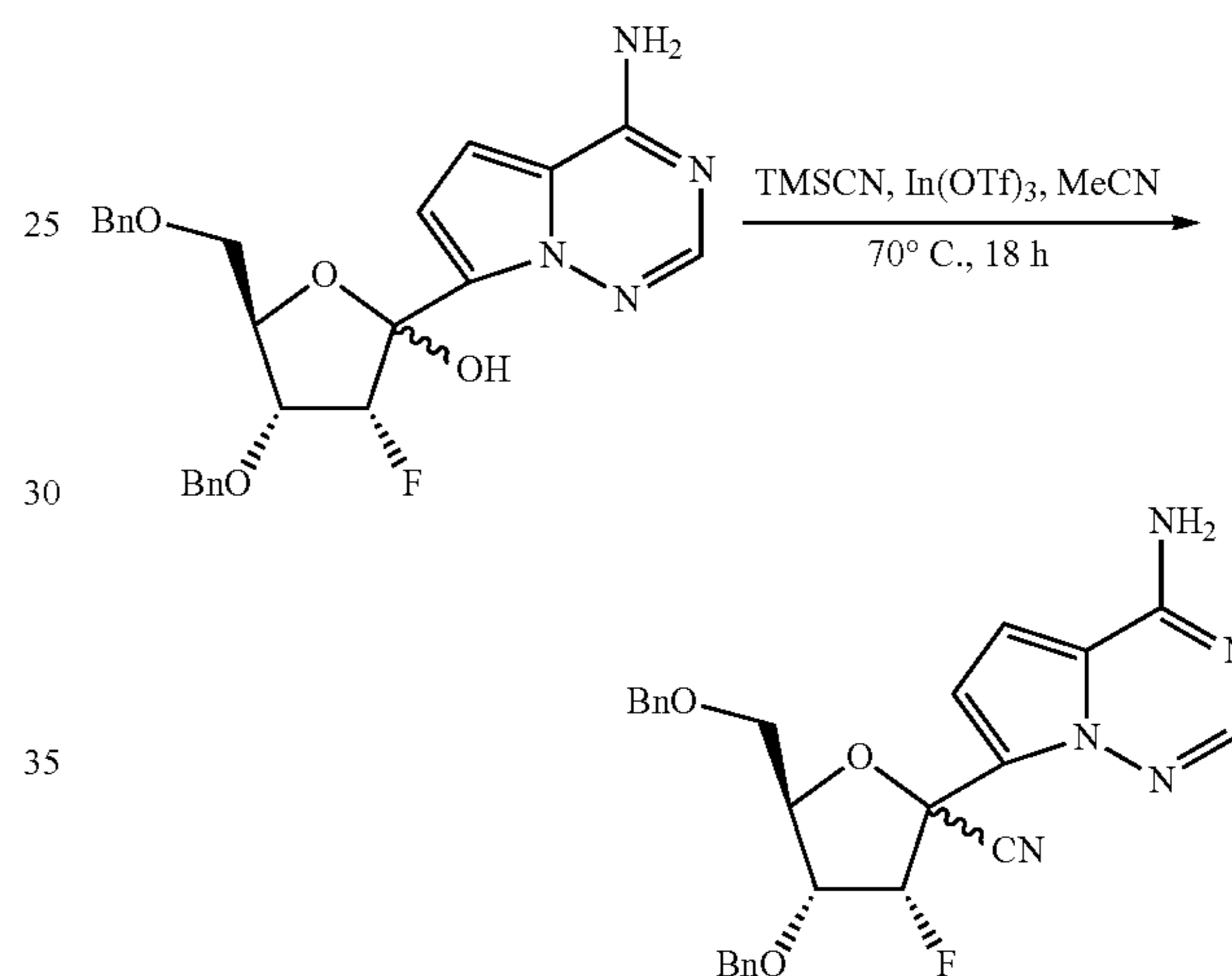
(3R,4R,5R)-2-(4-aminopyrrolo[1,2-f][1,2,4]triazin-7-yl)-4-(benzyloxy)-5-(benzyloxymethyl)-3-fluorotetrahydrofuran-2-carbonitrile
