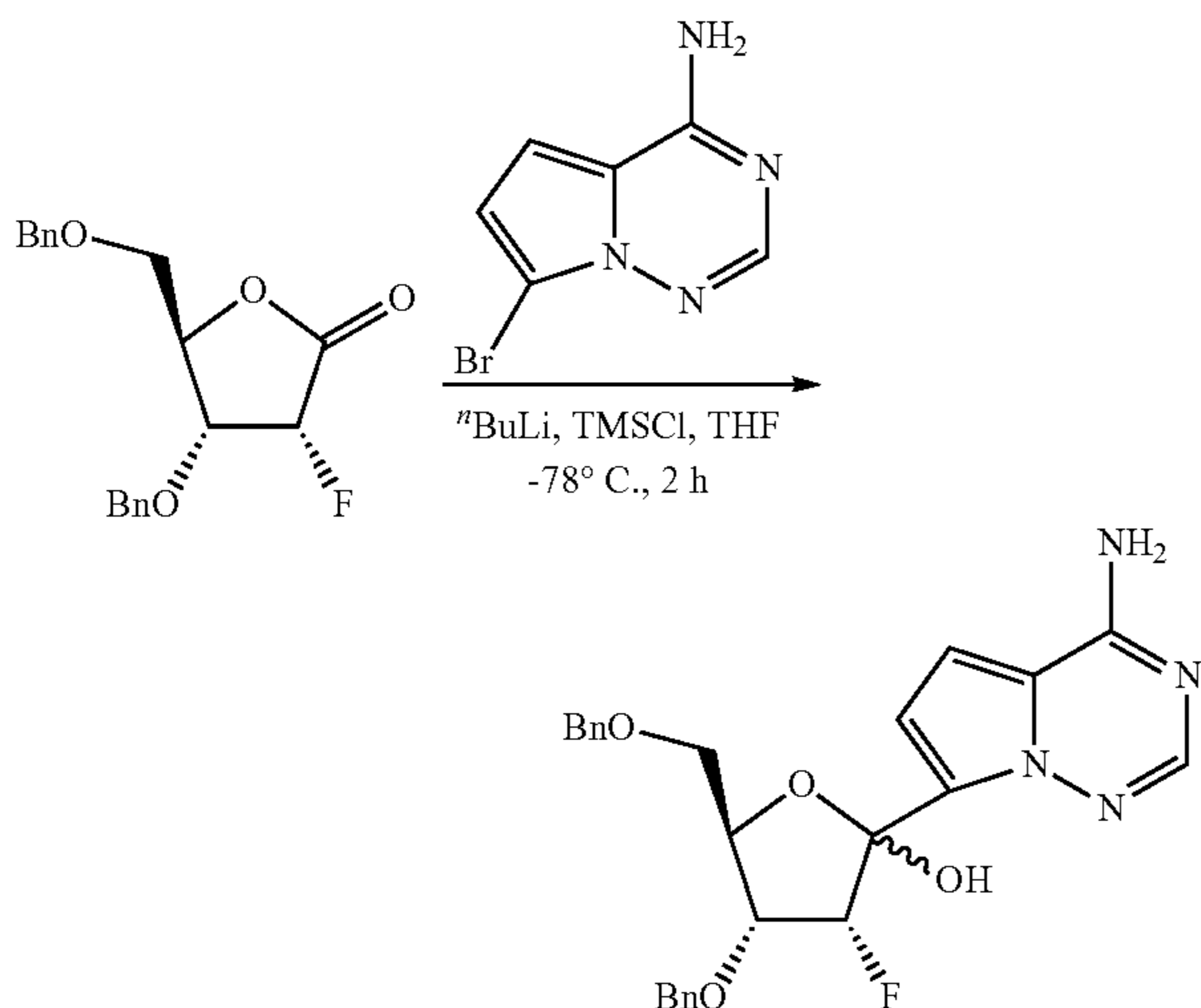
(3R,4R,5R)-2-(4-aminopyrrolo[1,2-f][1,2,4]triazin-7-yl)-4-(benzyloxy)-5-(benzyloxymethyl)-3-fluorotetrahydrofuran-2-ol
