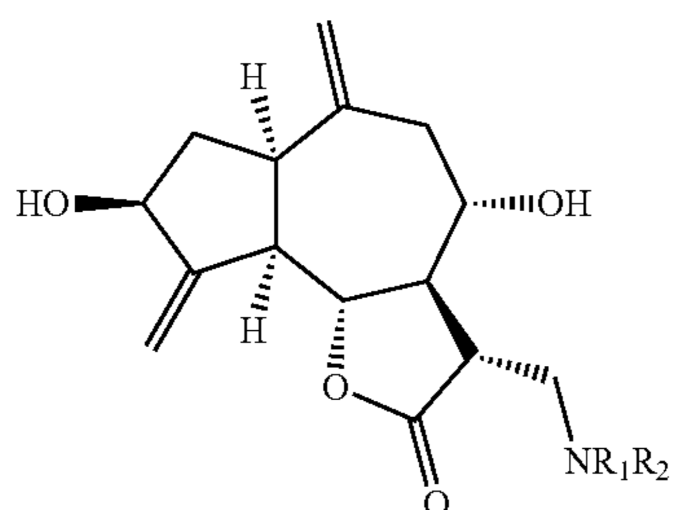
Aminodesacylcynarpicrins
