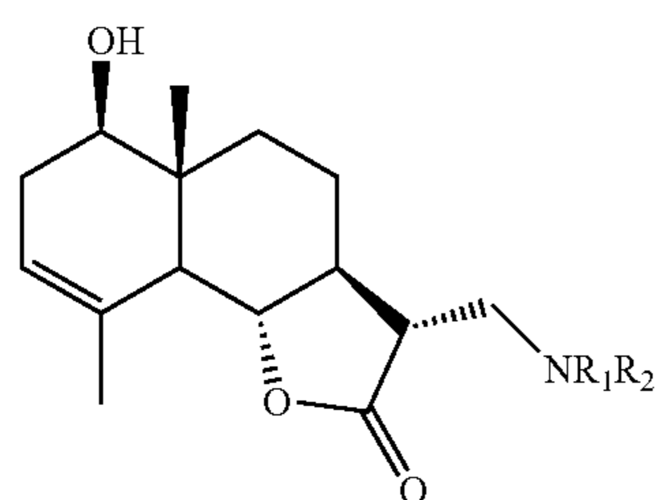
Aminosantamarins
