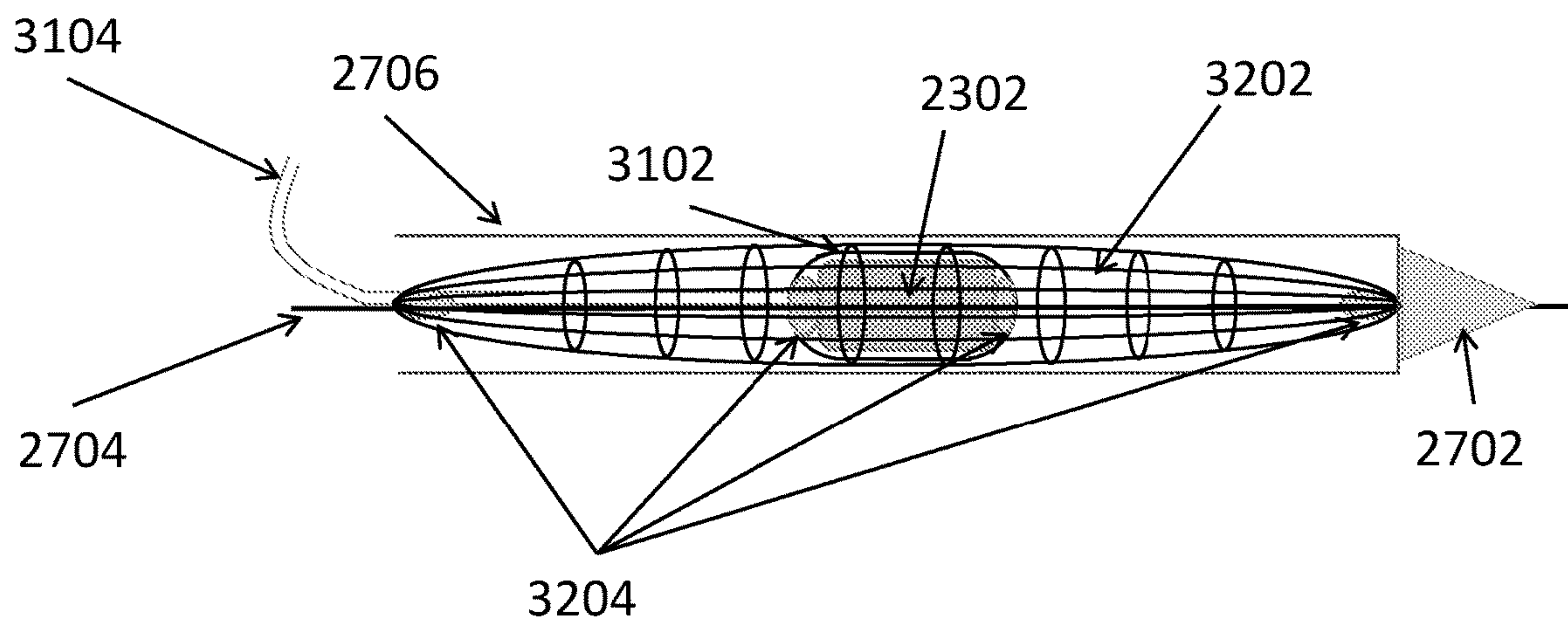
FIG. 32
