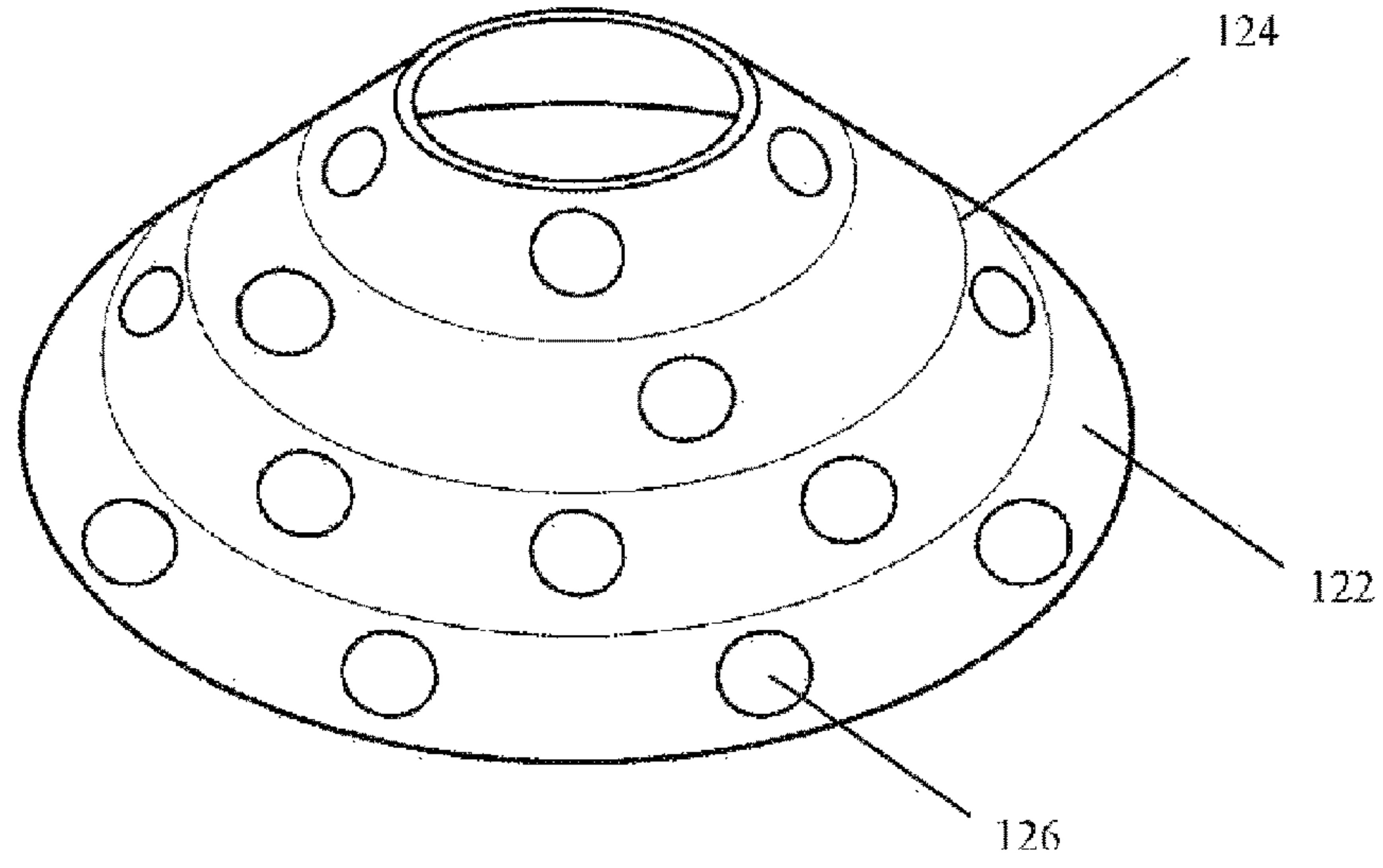
FIG. 11A
