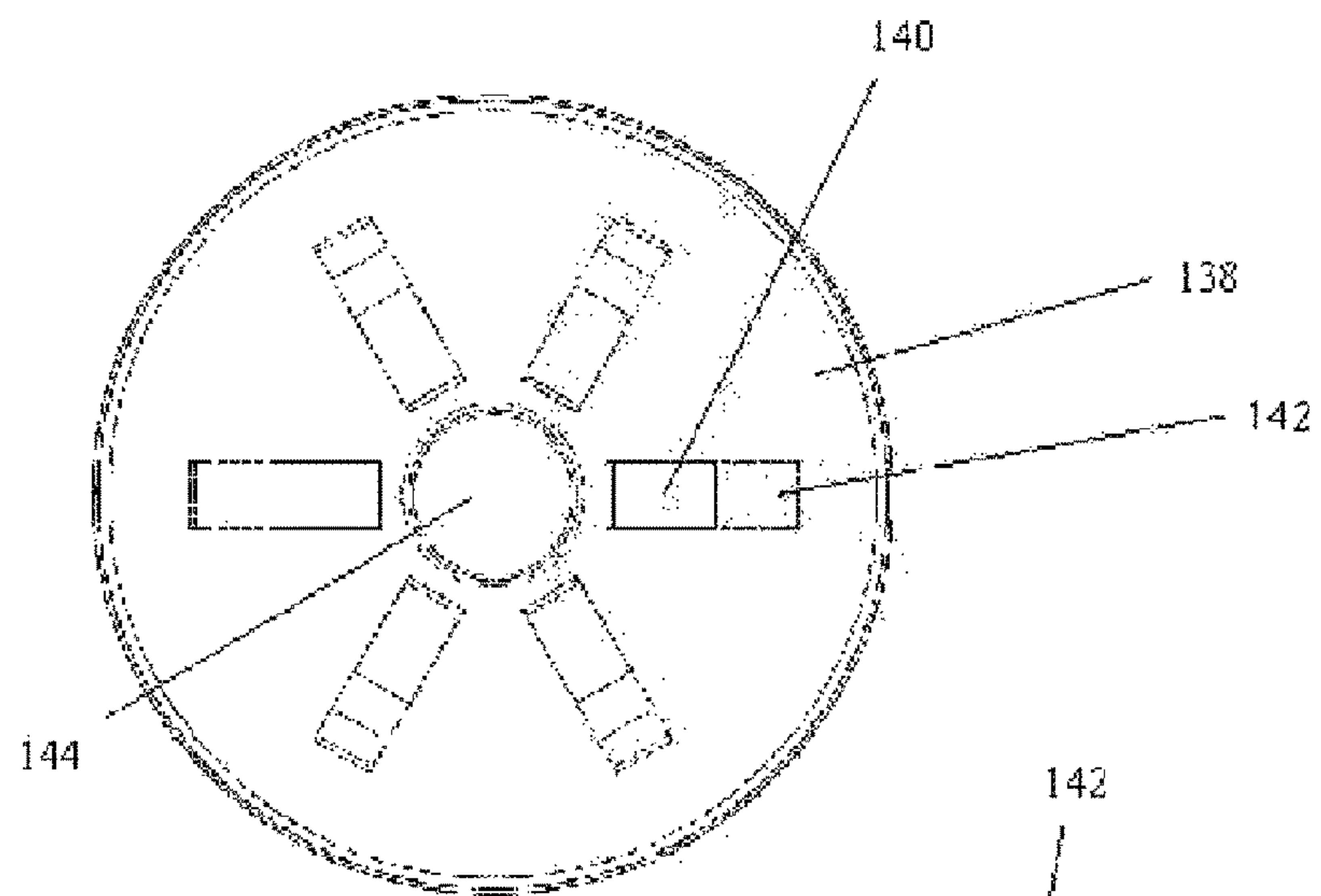
FIG. 15B
