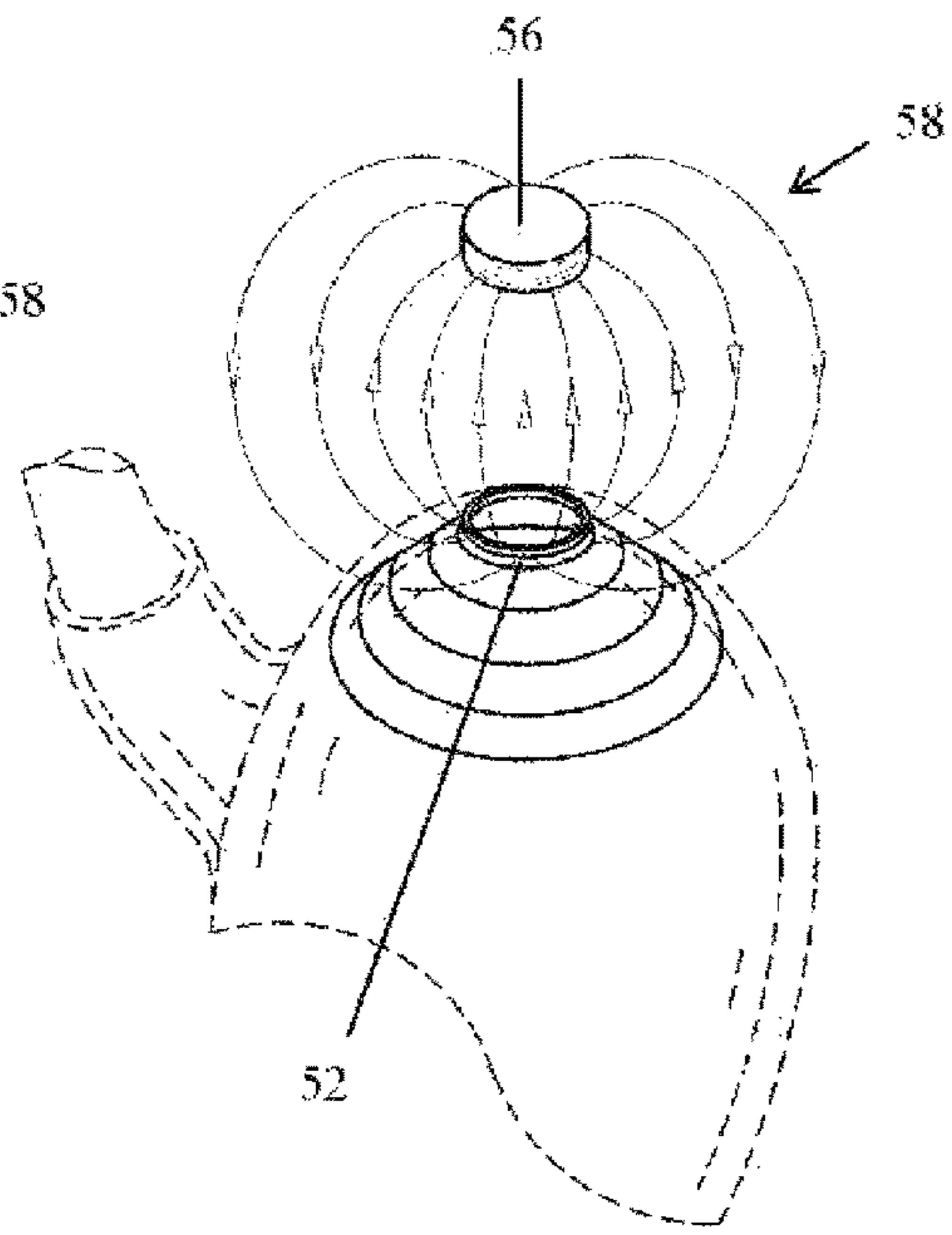
FIG. 2C
