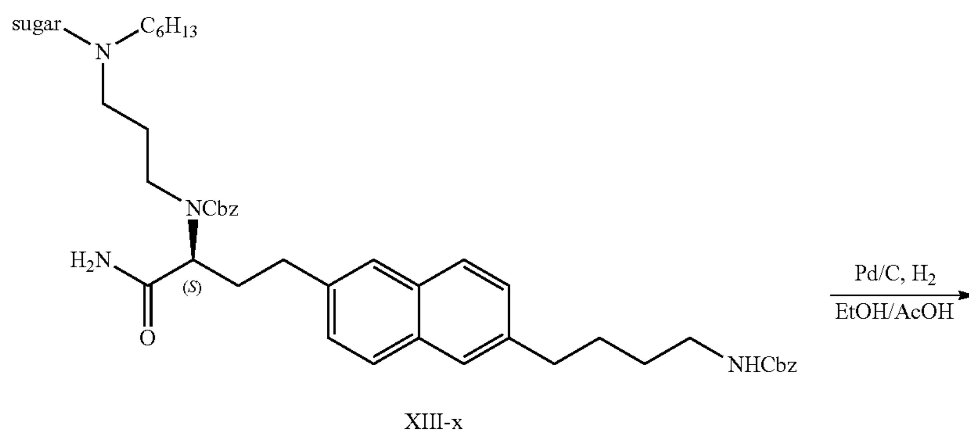
Scheme XIV 3,5-diamino-N-(N-(4-(6-((S)-4-amino-3-(3-hexyl((2S,3R,4R,5R)-2,3,4,5,6-pentahydroxyhexyl)amino)propylamino)-4-oxobutyl)naphthalen-2-yl)butyl)carbamide)-6-chloropyrazine-2-carboxamide
