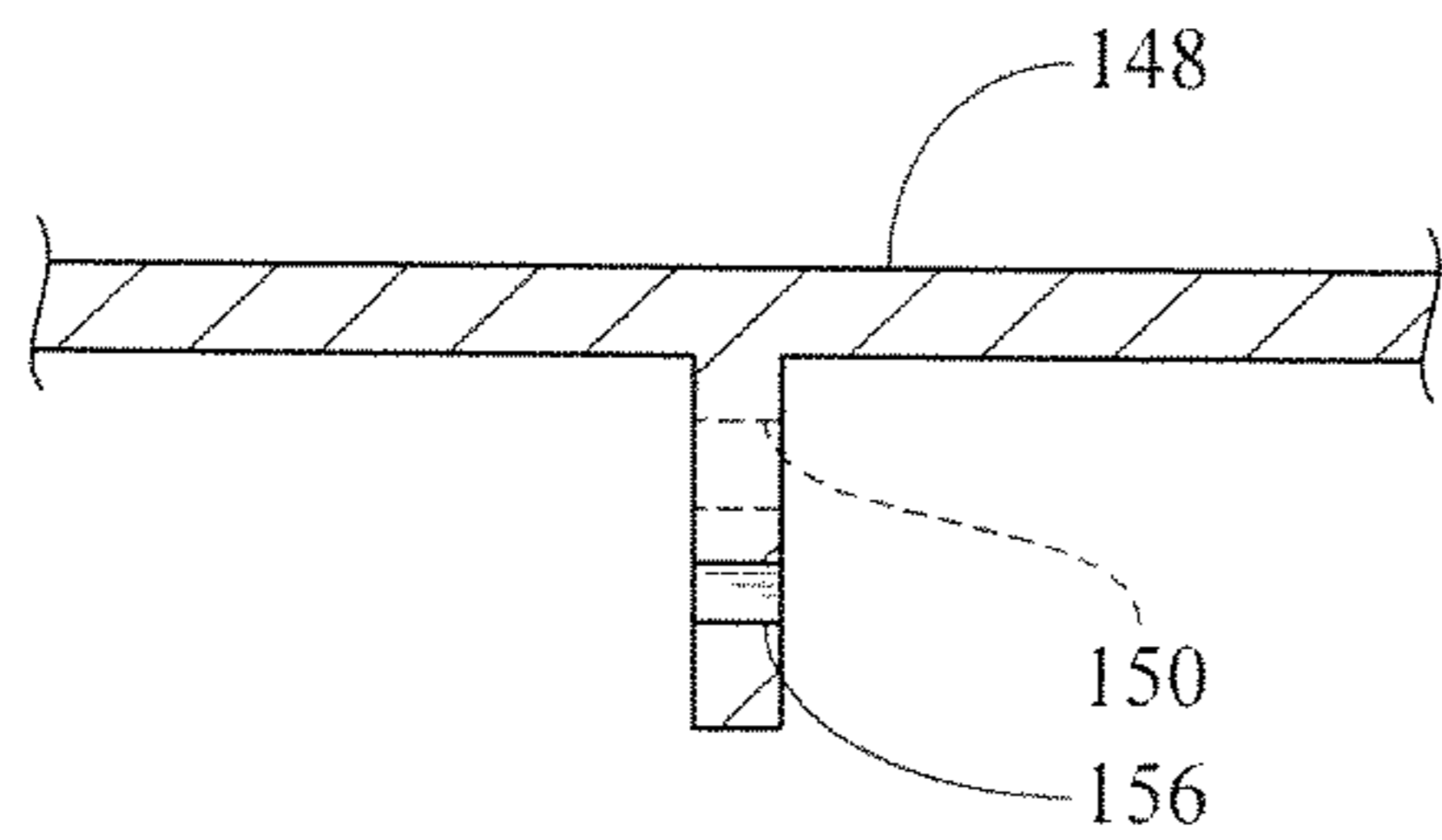
FIG. 6 (SECT. A-A)
