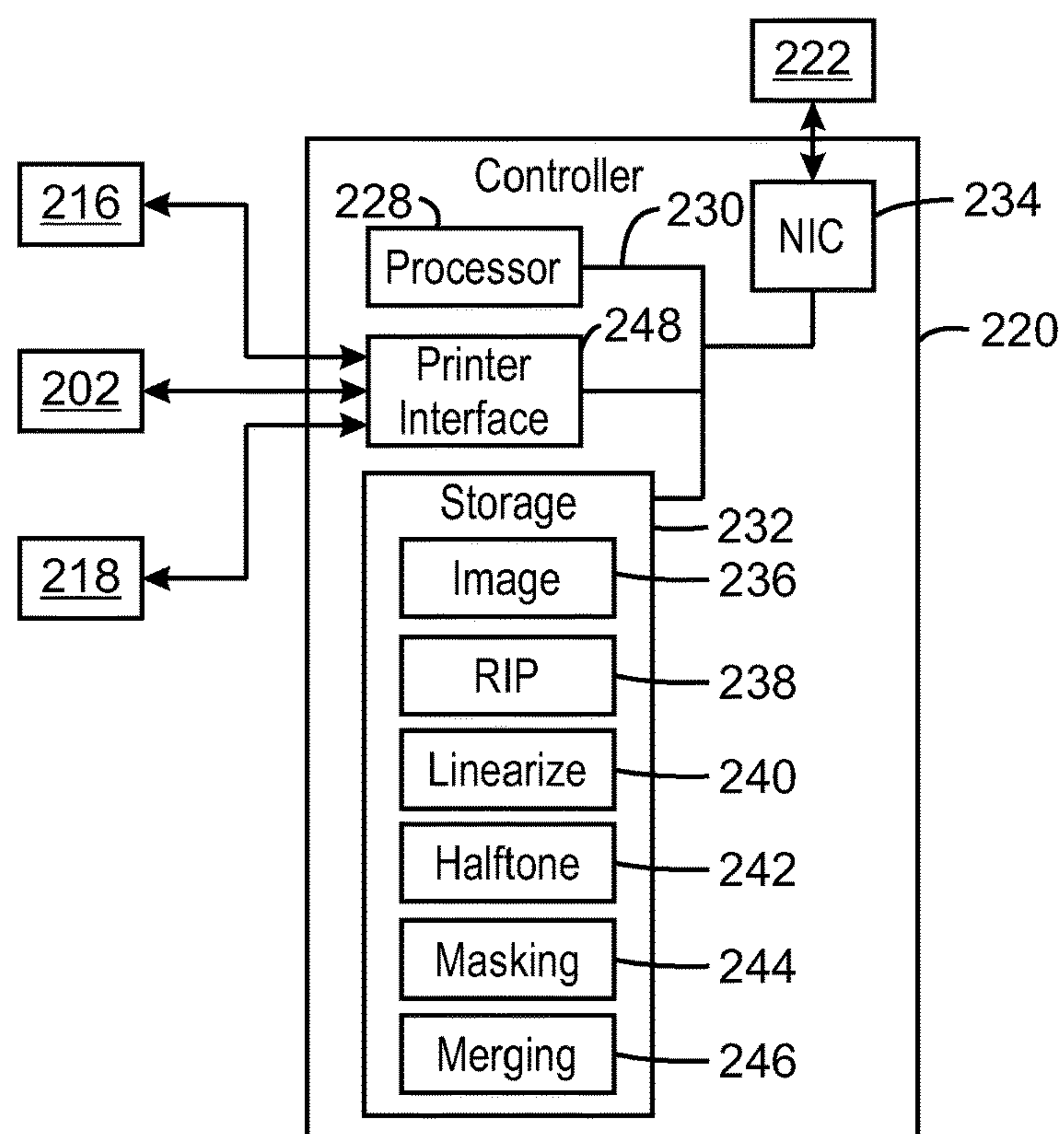
200 FIG. 2A
