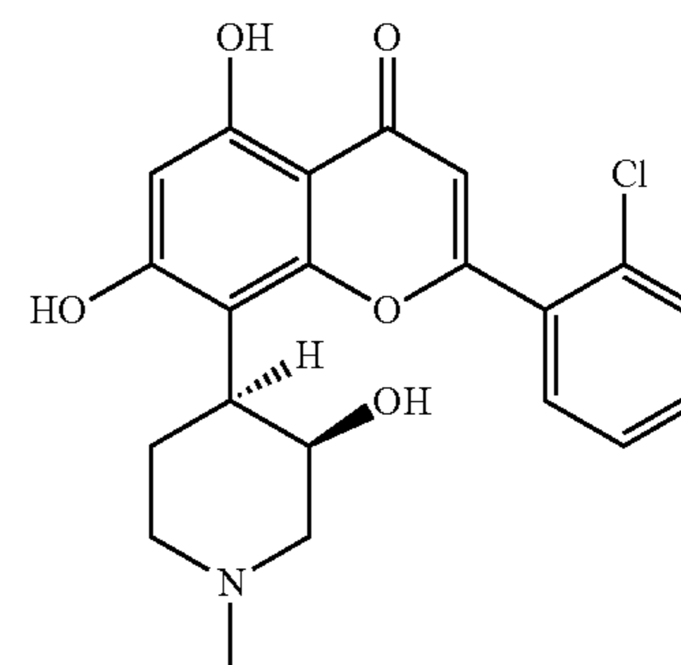
flavopiridol
