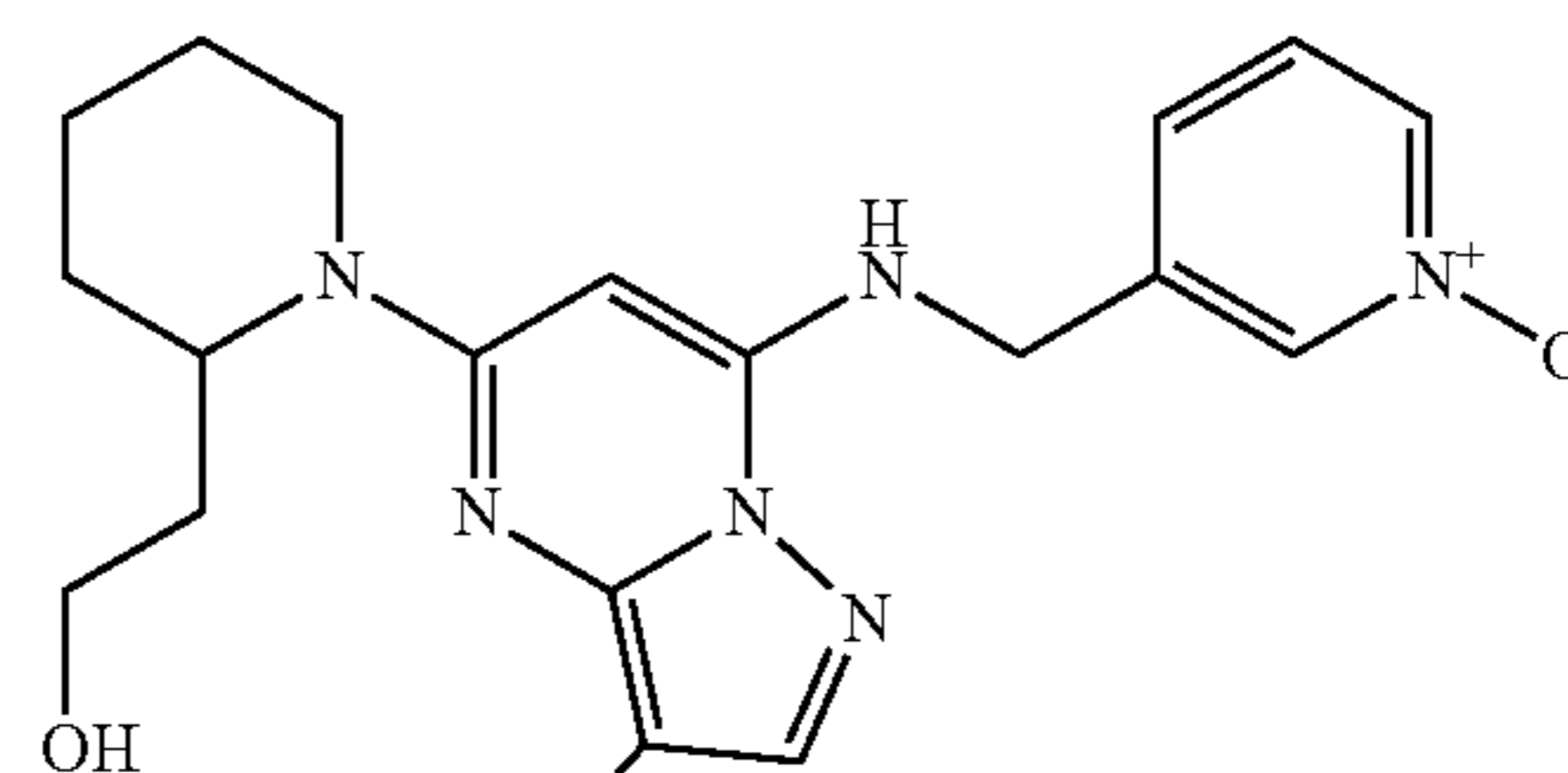
dinaciclib
