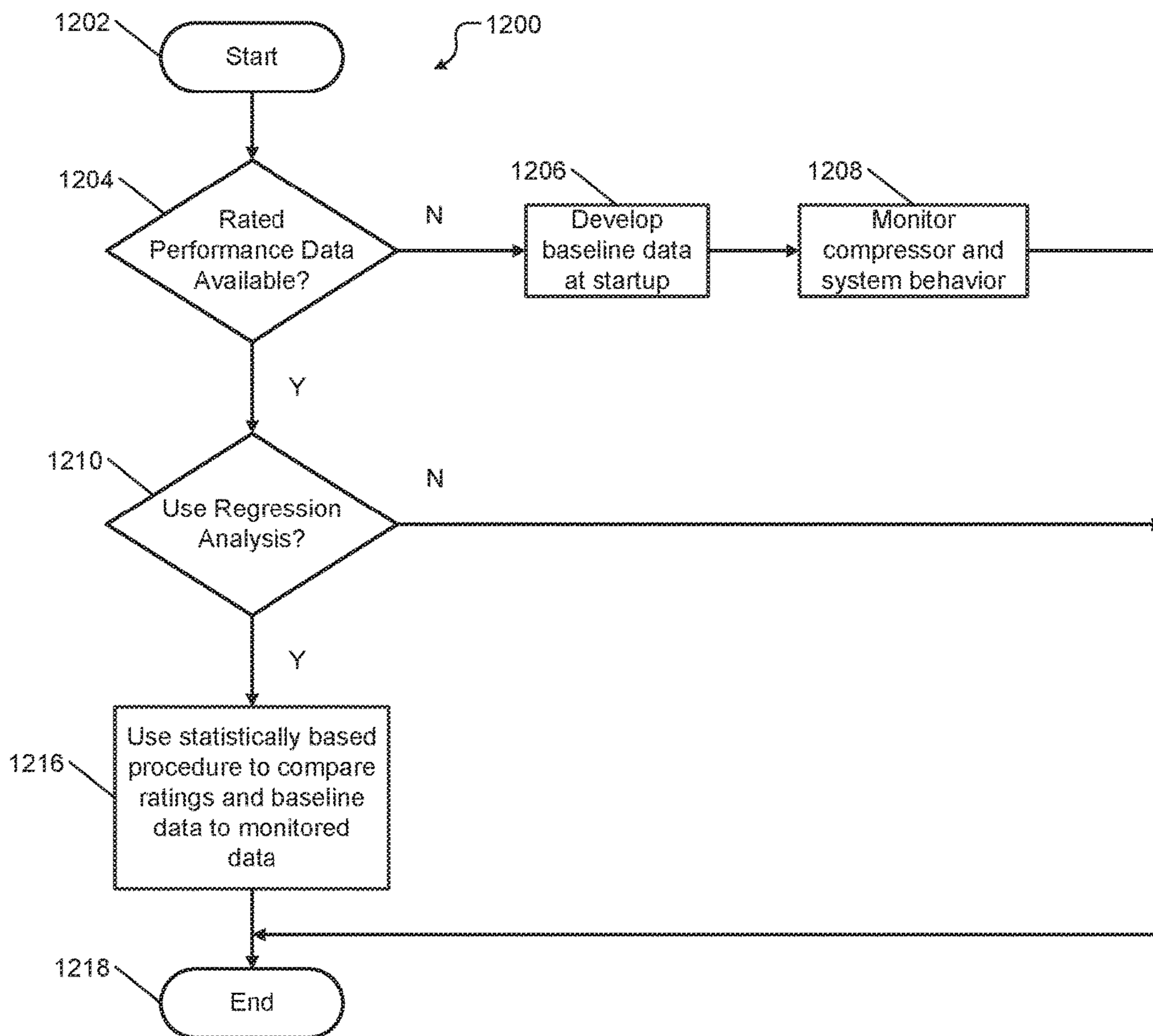
FIG. 12
