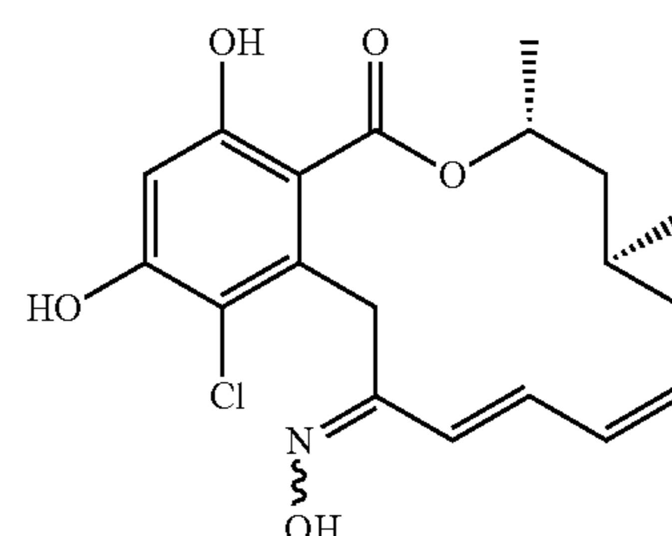
Cycloproparadicicol
