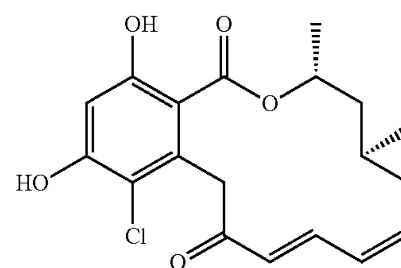
Cycloproparadicicol
