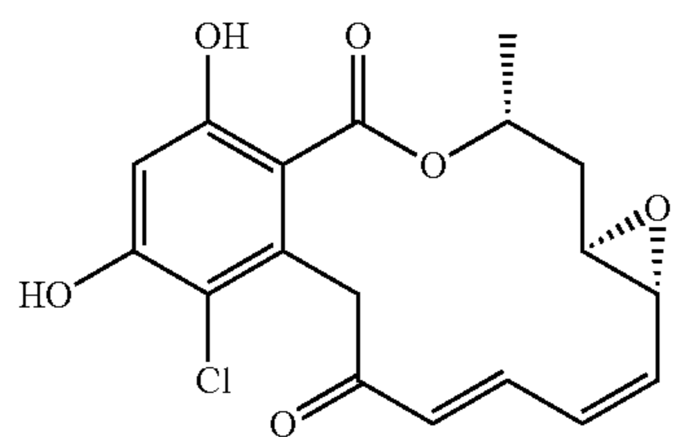
Radicol
