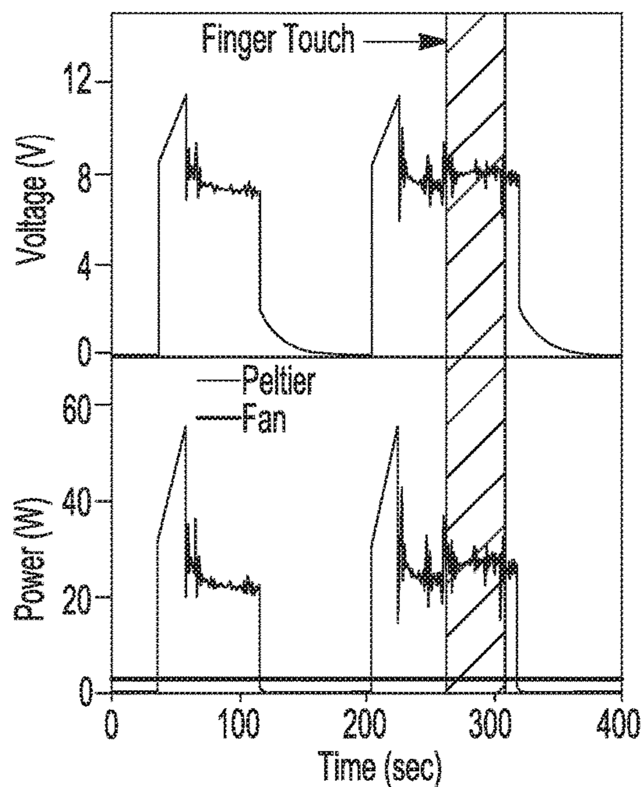
Fig-5B
