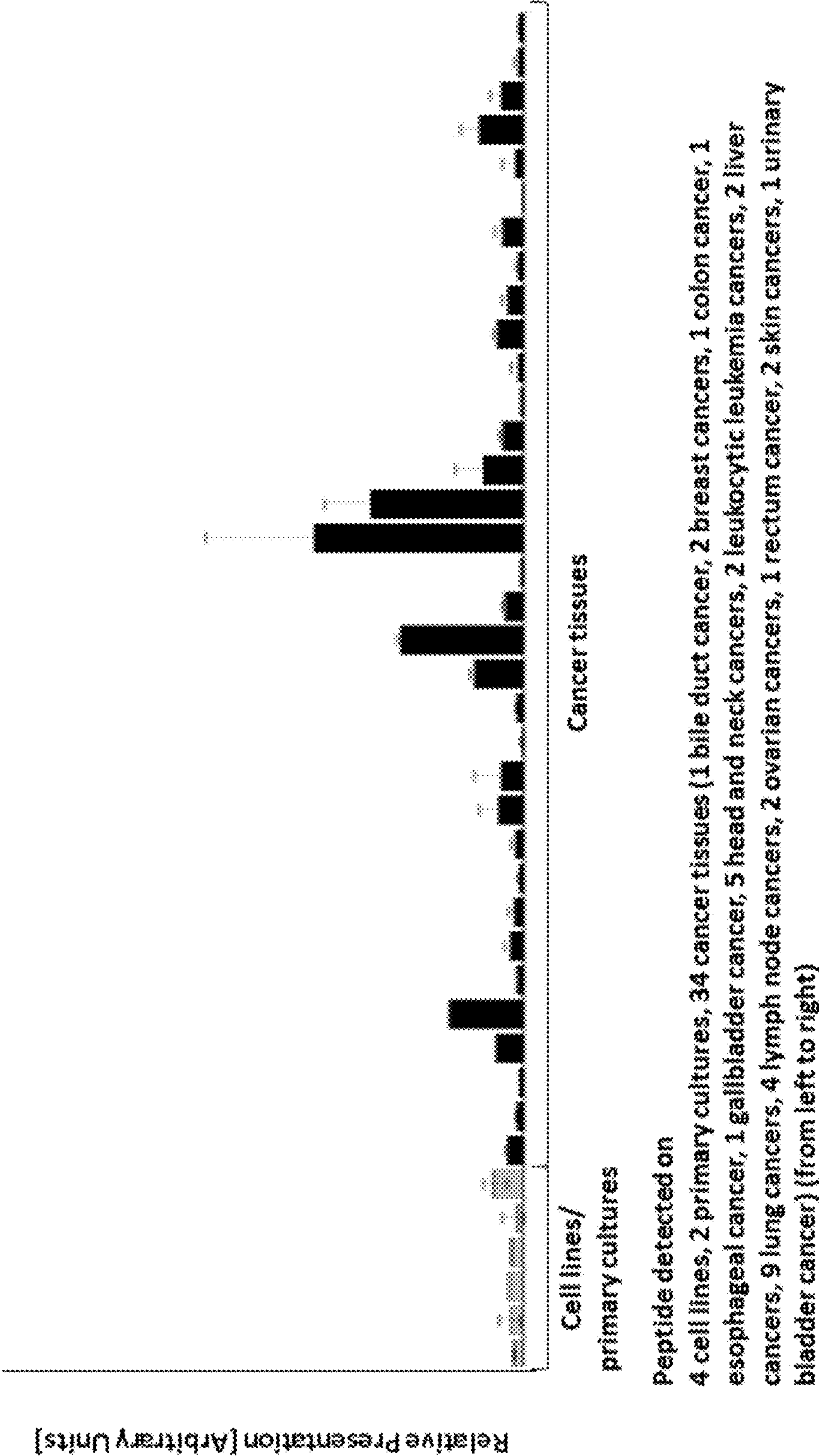
Figure 1R Peptide: YMFEFVPIVI(A*02) SEQ ID NO: 200
