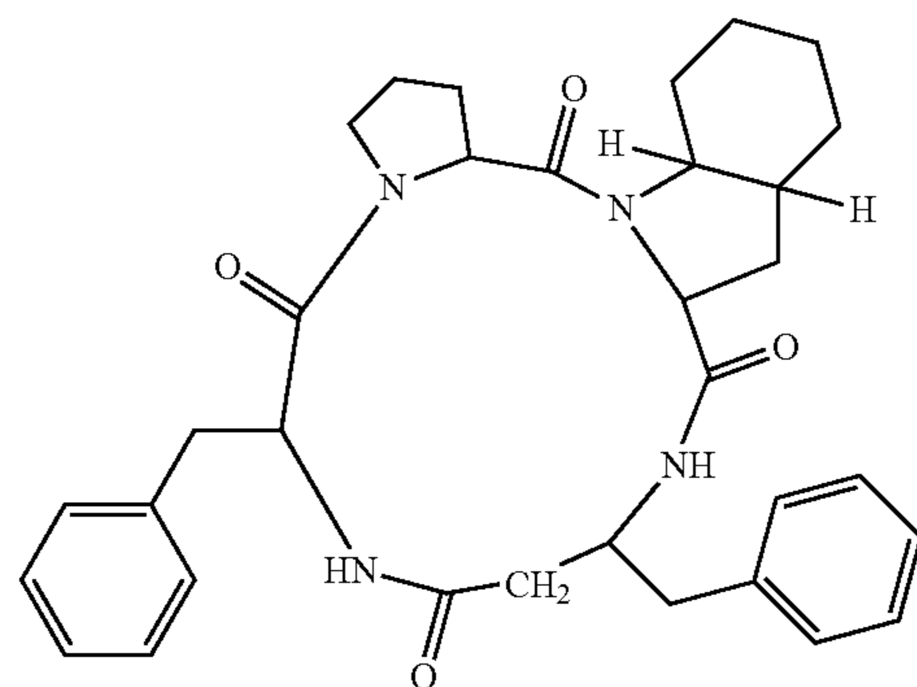
(cyclo(-Pro-Oic-β 3 hoPhe-Phe))
