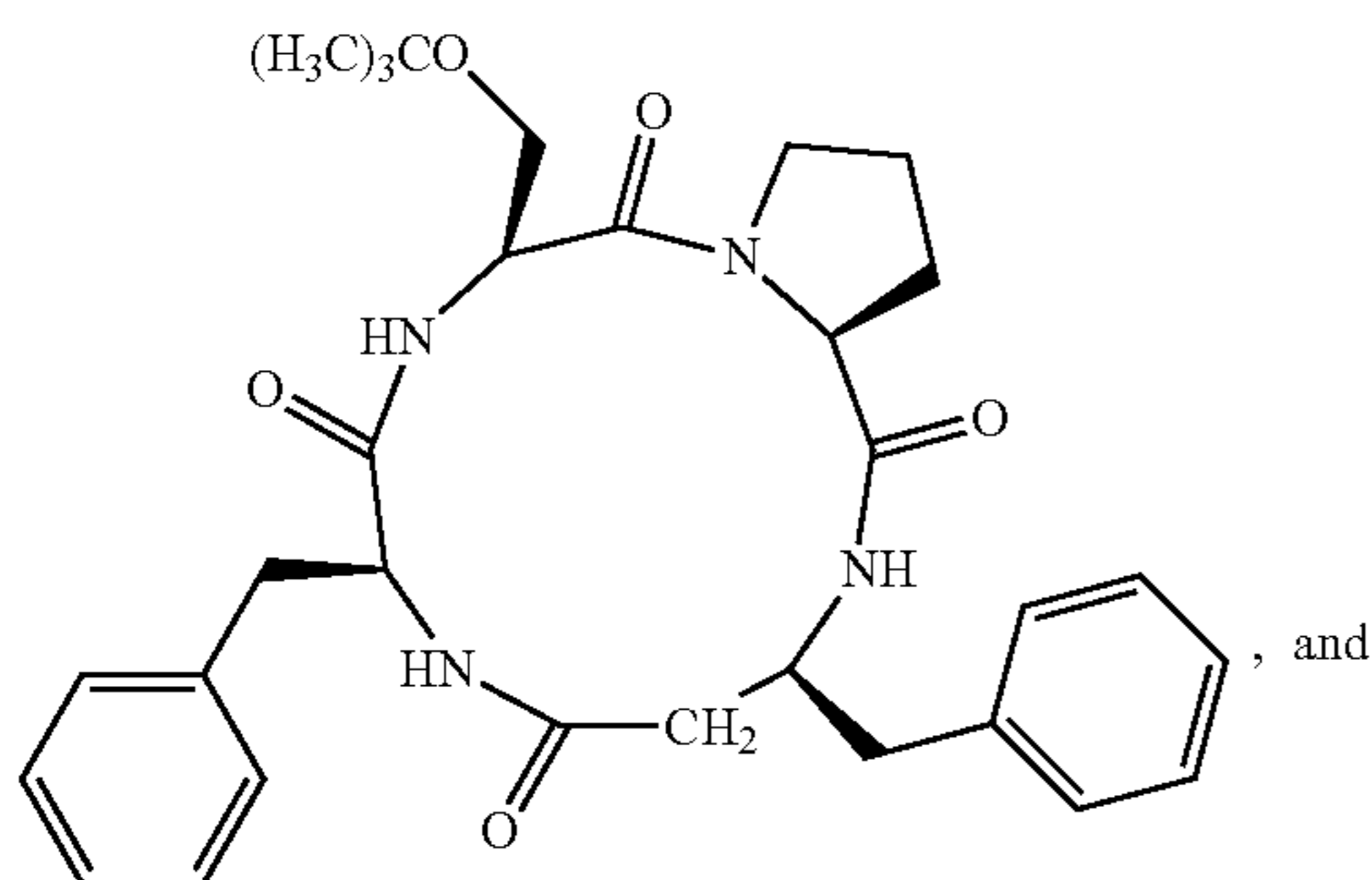
(cyclo(-L-Ser(tBu)-L-Pro-L-β 3 hoPhe-L-Phe))
