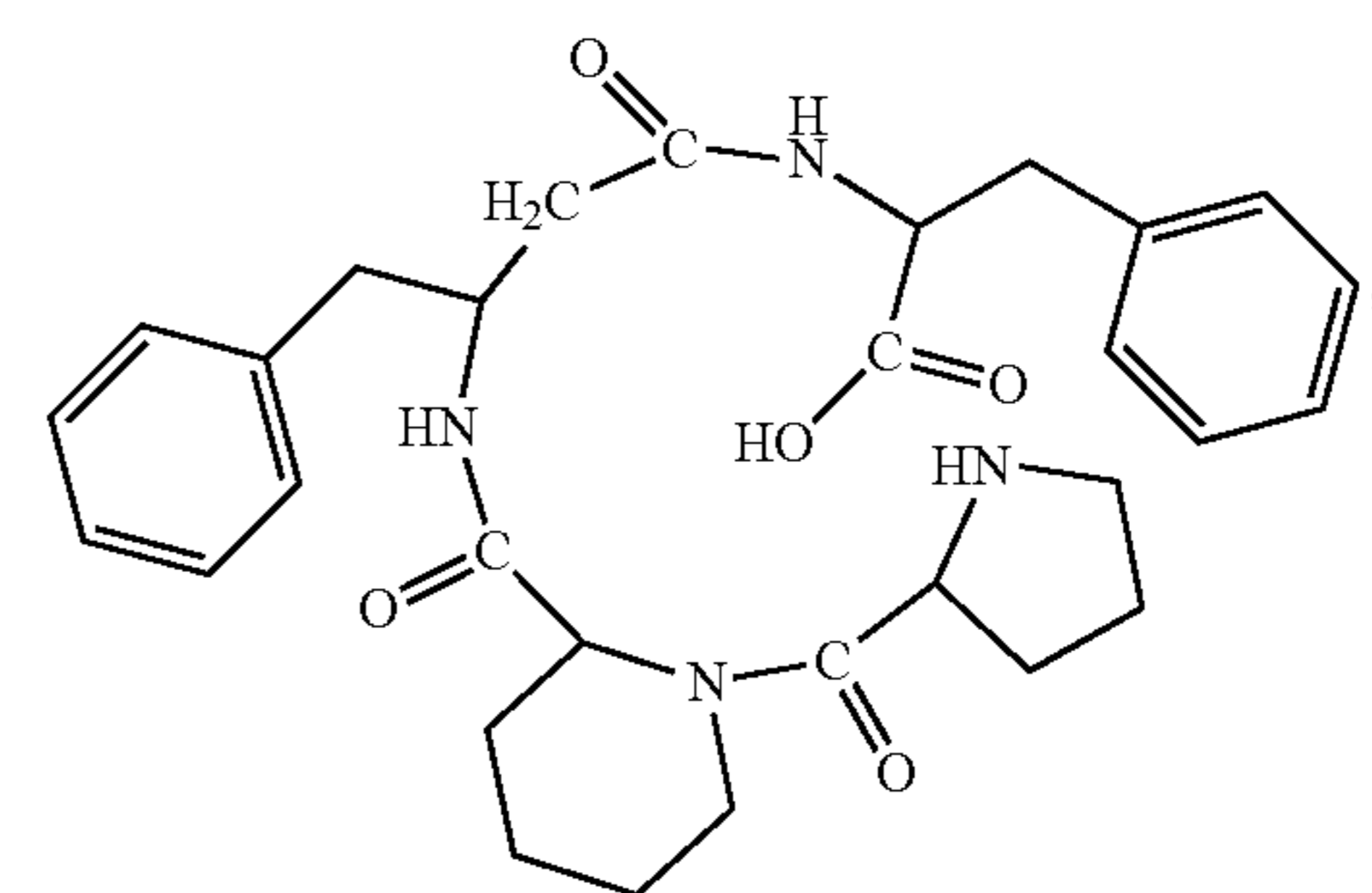
(H-Pro-Pip-β 3 hoPhe-Phe-OH)
