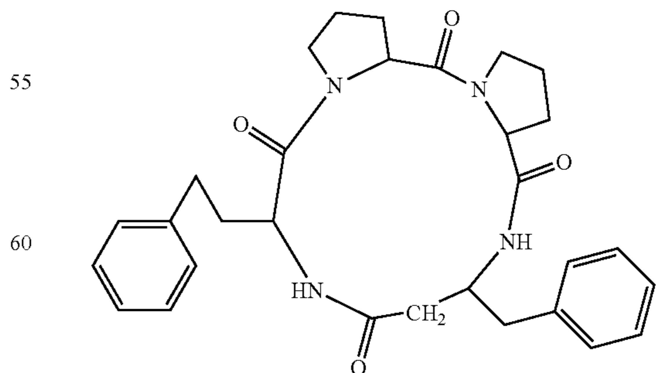
(cyclo(-Pro-Pro-β³hoPhe-hoPhe))
