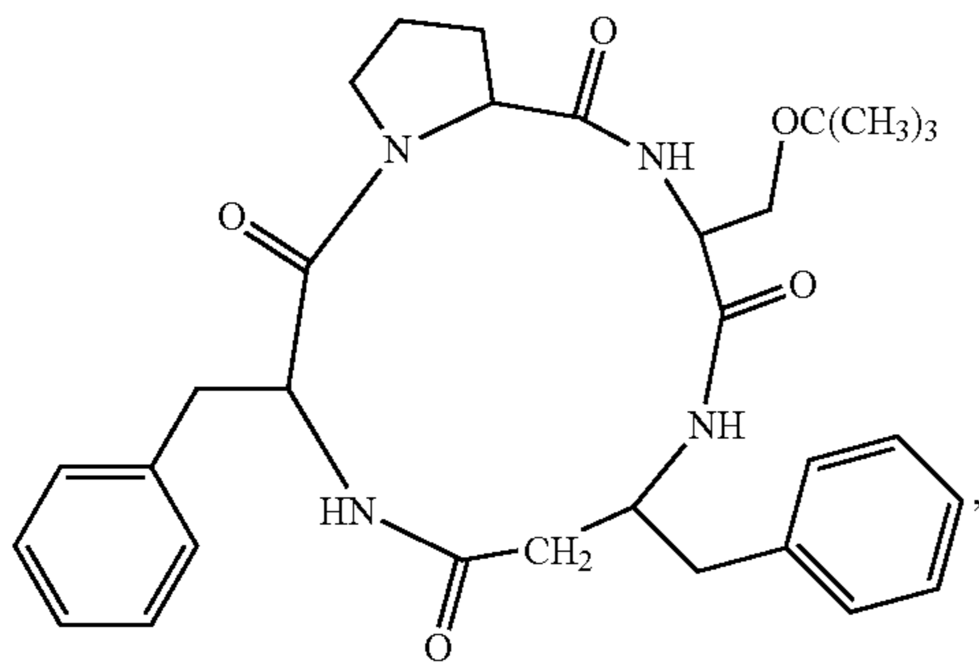
(cyclo(-Pro-Ser(tBu)-β³hoPhe-Phe))
