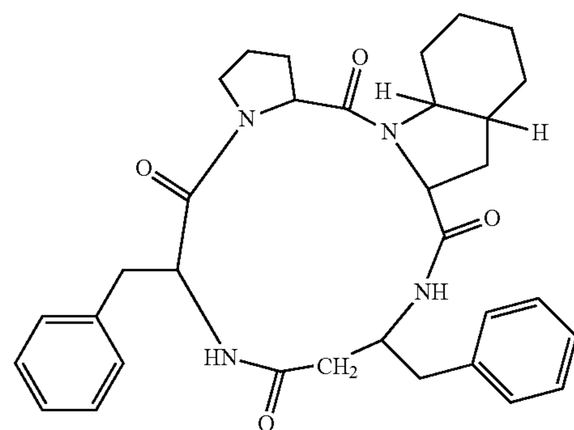
(cyclo(-Pro-Oic-β³hoPhe-Phe))
