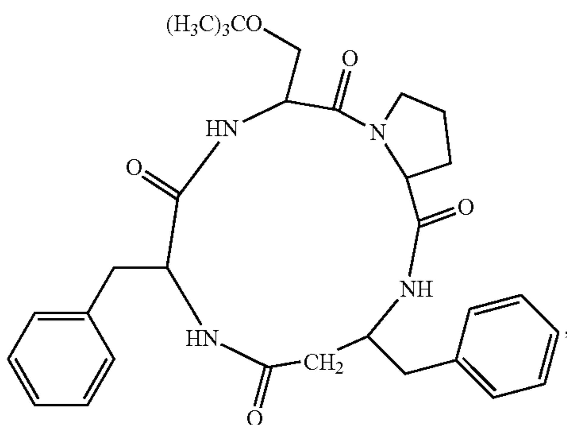
(cyclo(-Ser(tBu)-Pro-β 3 hoPhe-Phe))
