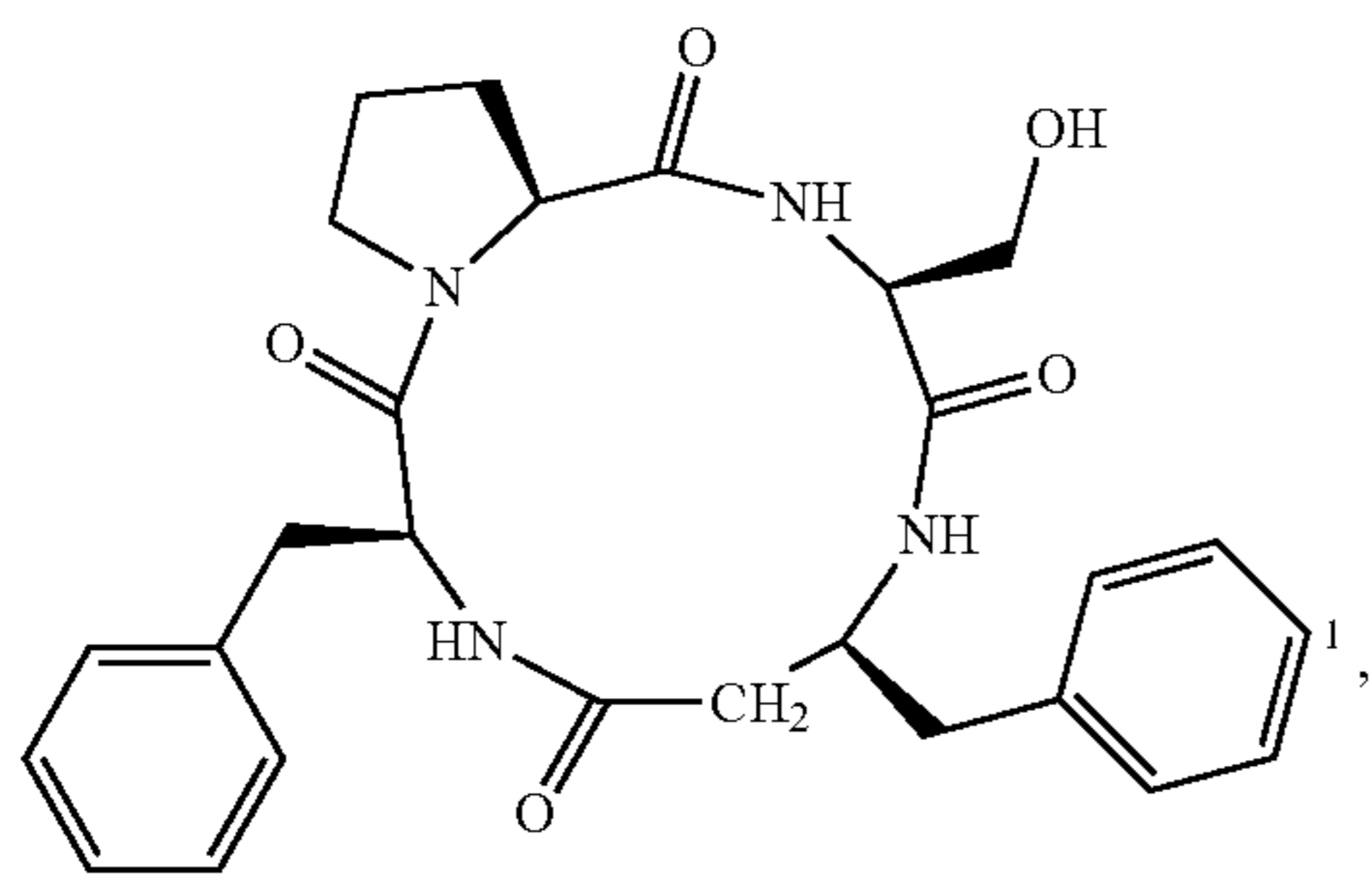
(cyclo(-L-Pro-L-Ser-L-β 3 hoPhe-L-Phe))
