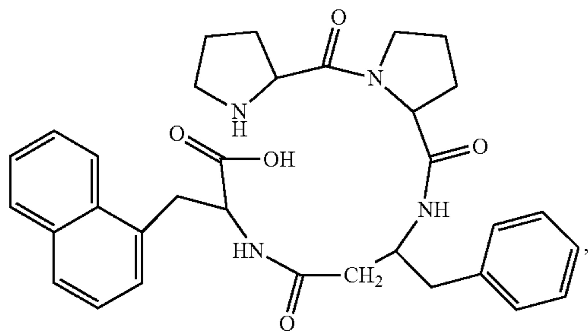
(H-Pro-Pro-β 3 hoPhe-1Nal-OH)
