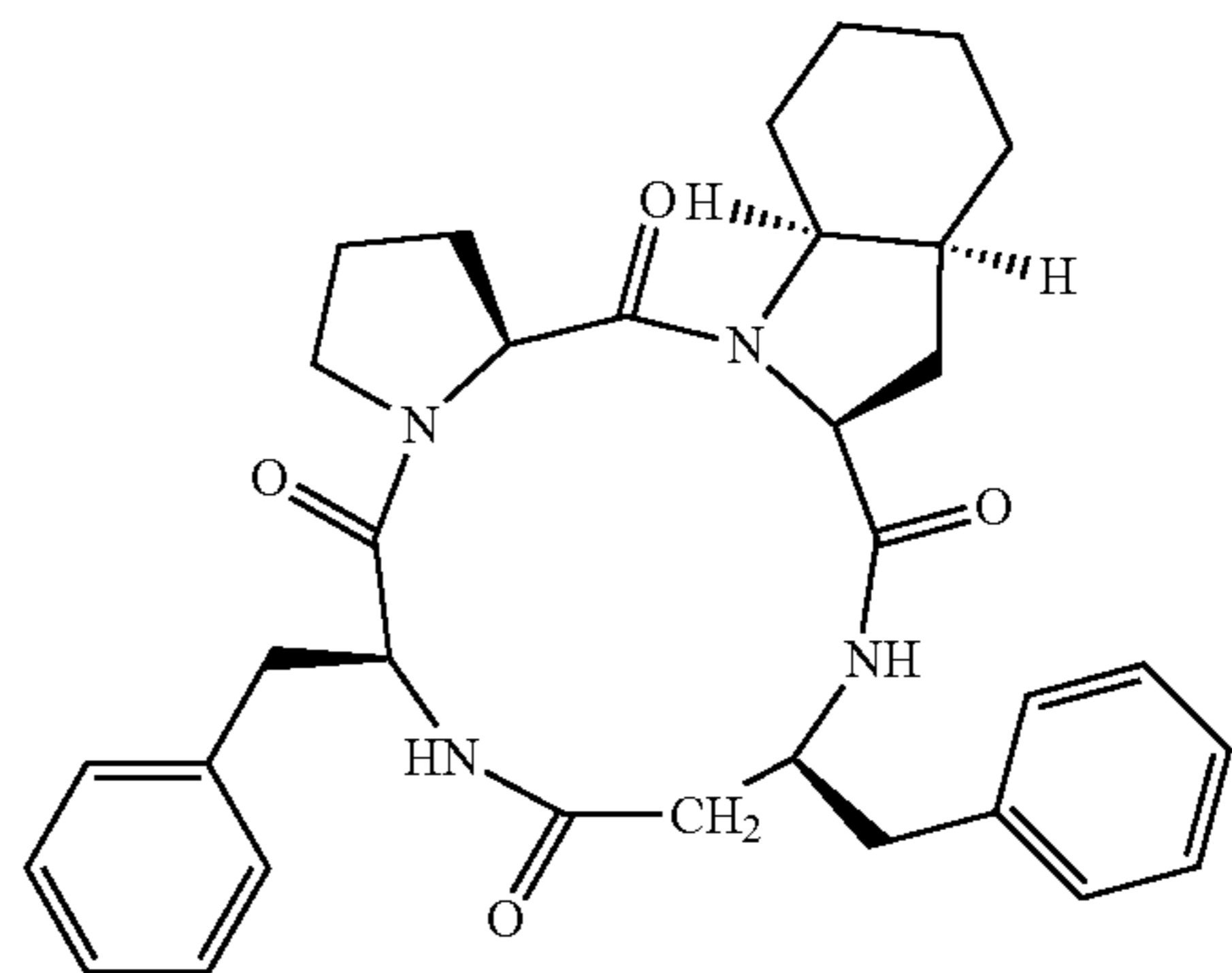
cyclo(-L-Pro-L-Oic-L-β³hoPhe-L-Phe))
