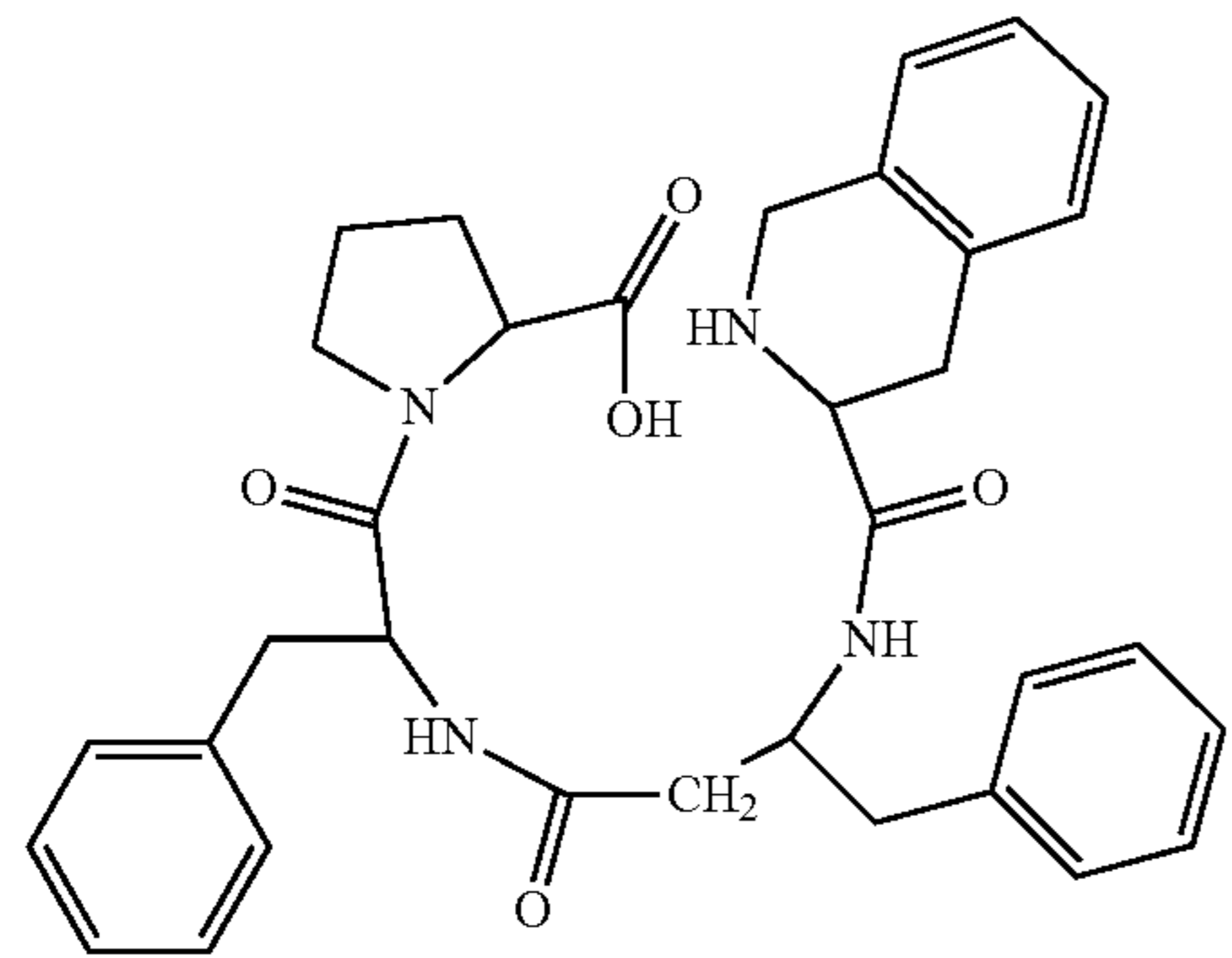
(H-Tic-β 3 hoPhe-Phe-Pro-OH)
