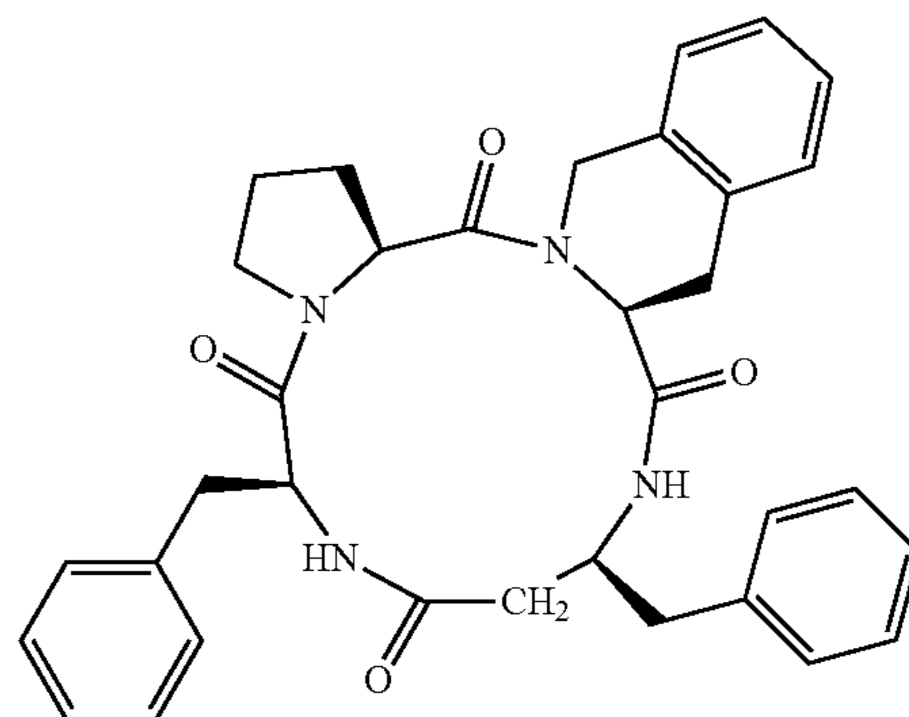
(cyclo(-L-Pro-L-Tic-L-β³hoPhe-L-Phe))
