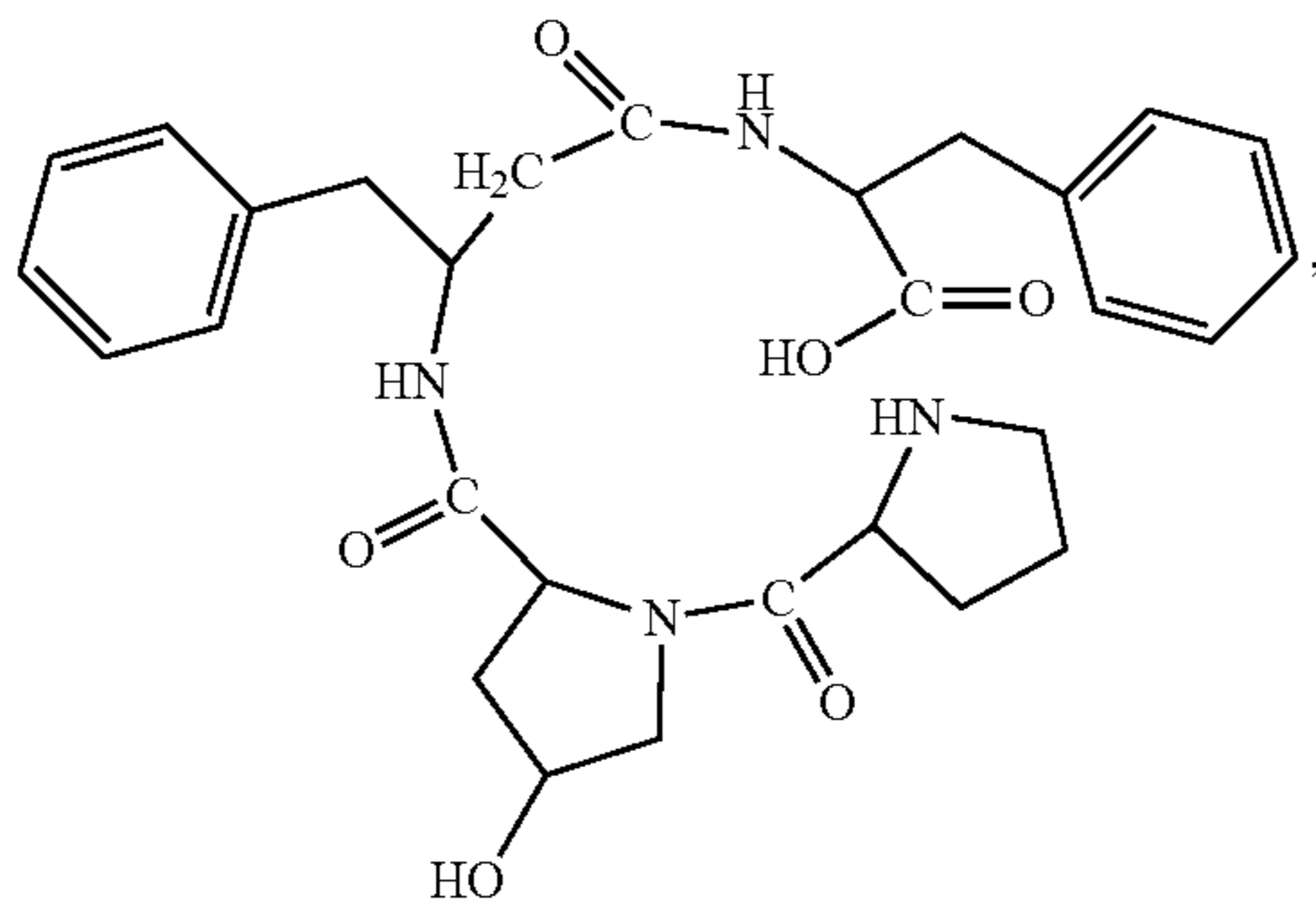
(H-Pro-Hyp-β 3 hoPhe-Phe-OH)
