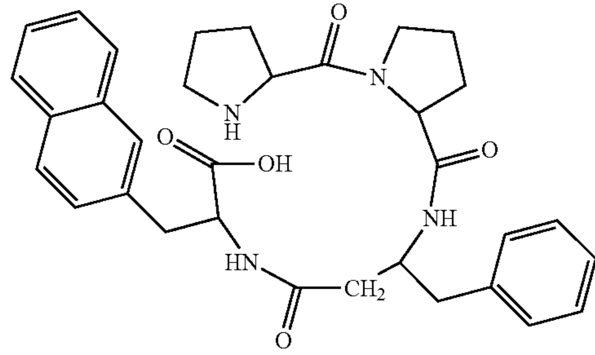
(H-Pro-Pro-β 3 hoPhe-2Nal-OH)
