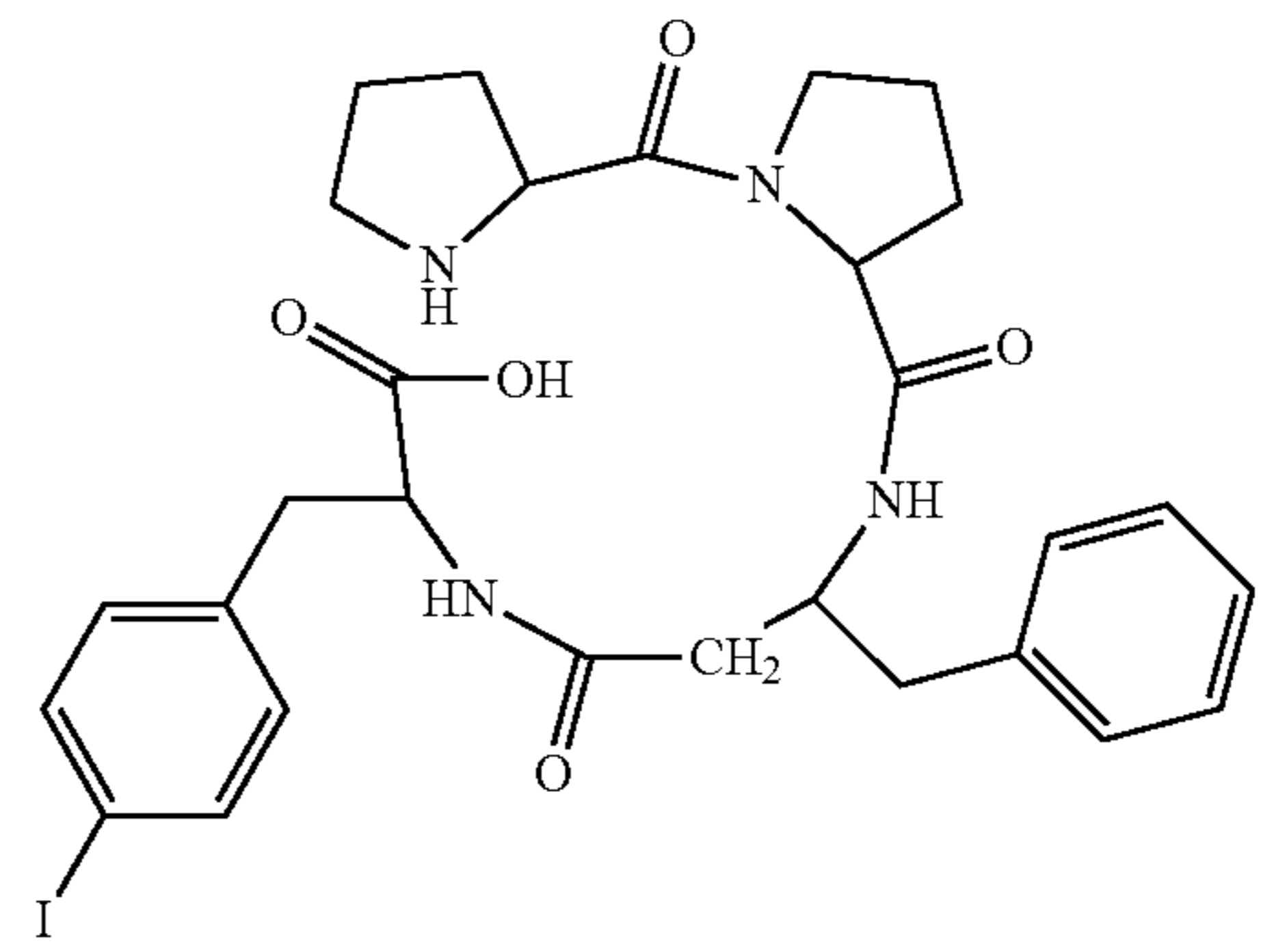
(H-Pro-Pro-β 3 hoPhe-Phe(4I)-OH)
