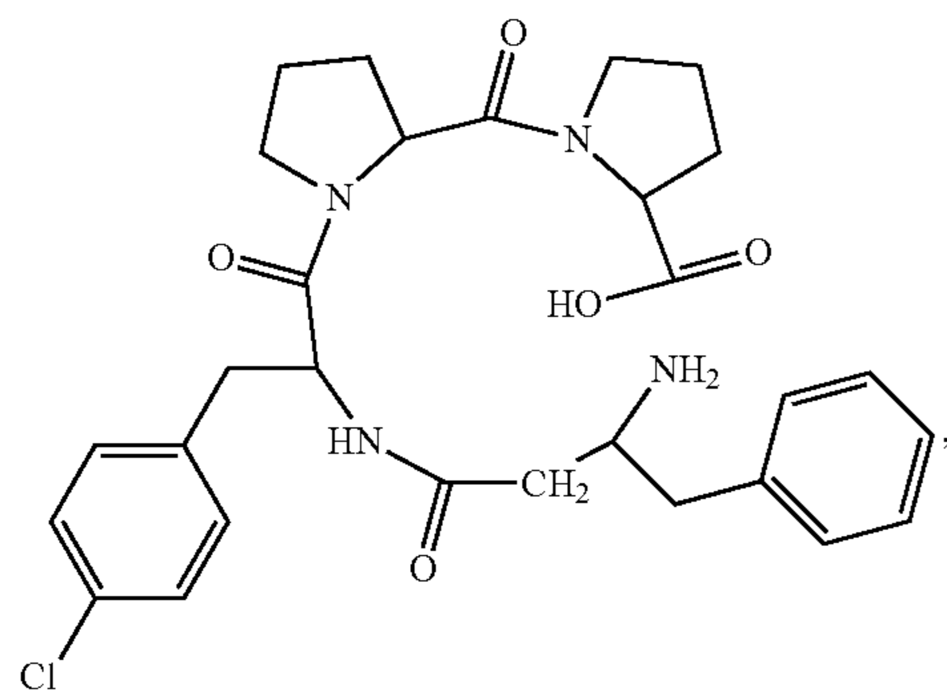
(H-β 3 hoPhe-Phe(4Cl)-Pro-Pro-OH)
