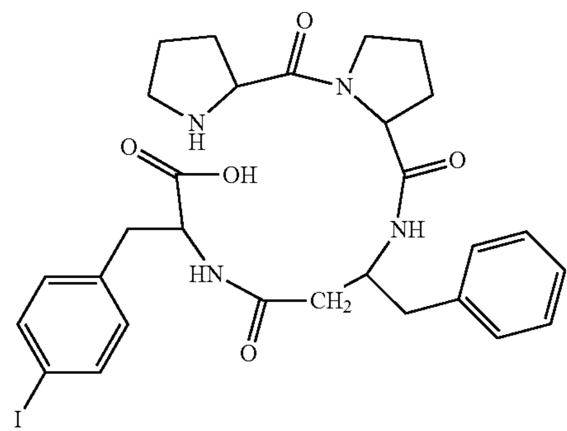
(H-Pro-Pro-β 3 hoPhe-Phe(4I)-OH)
