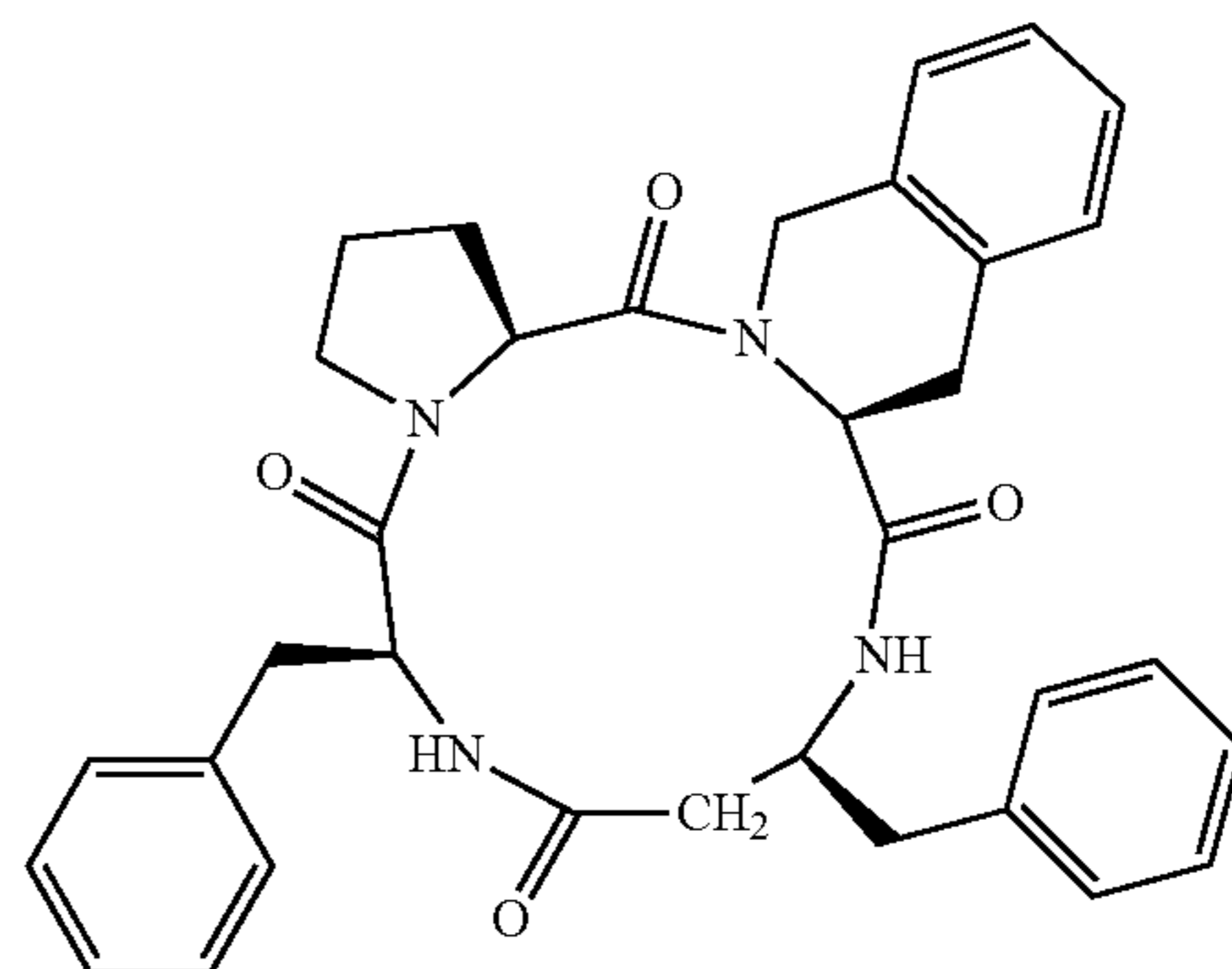
(cyclo(-L-Pro-L-Tic-L-β³hoPhe-L-Phe))
