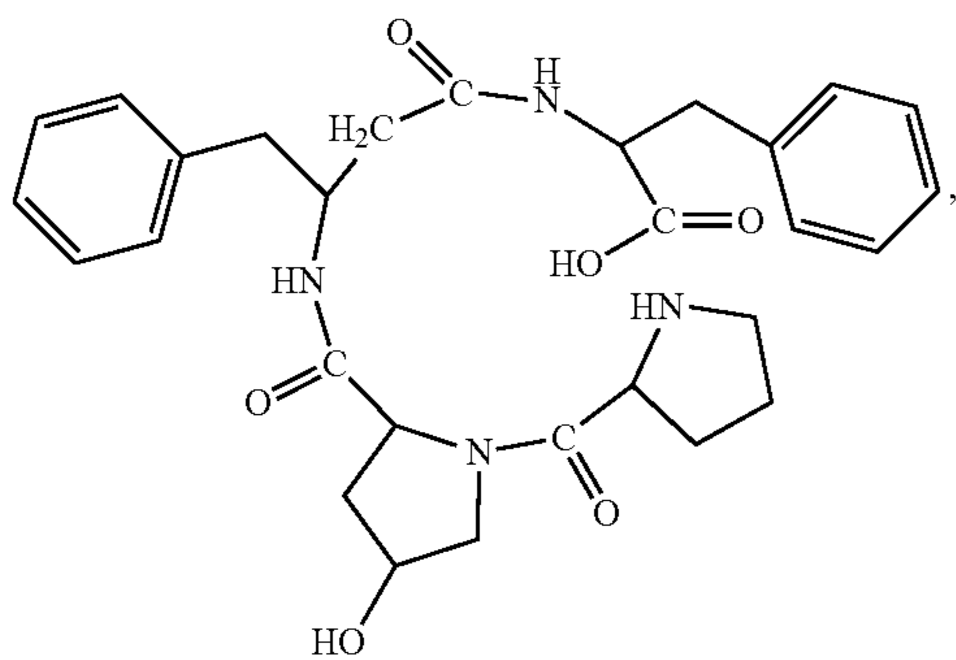
(H-Pro-Hyp-β 3 hoPhe-Phe-OH)
