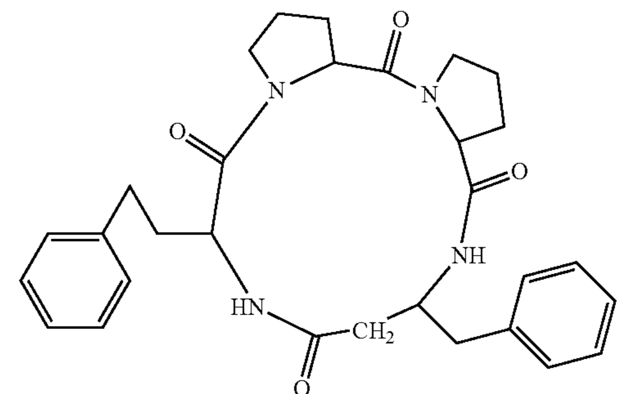
(cyclo(-Pro-Pro-β³hoPhe-hoPhe))
