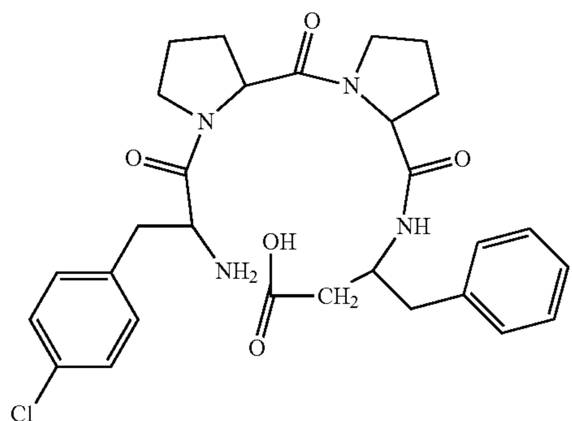
(H-Phe(4Cl)-Pro-Pro-β 3 hoPhe-OH)
