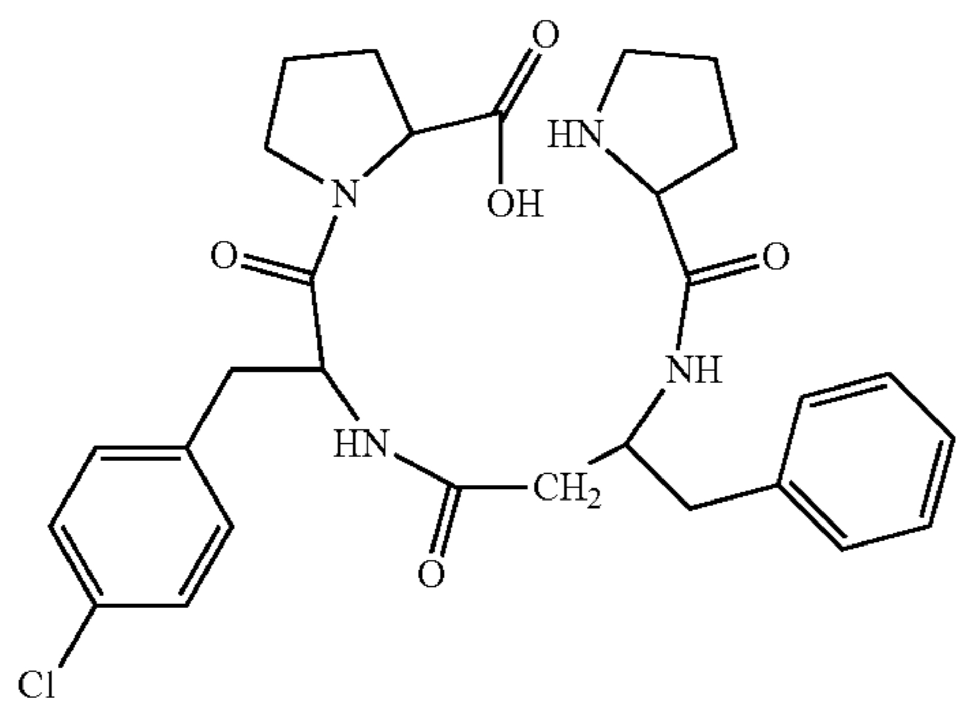
(H-Pro-β 3 hoPhe-Phe(4Cl)-Pro-OH)
