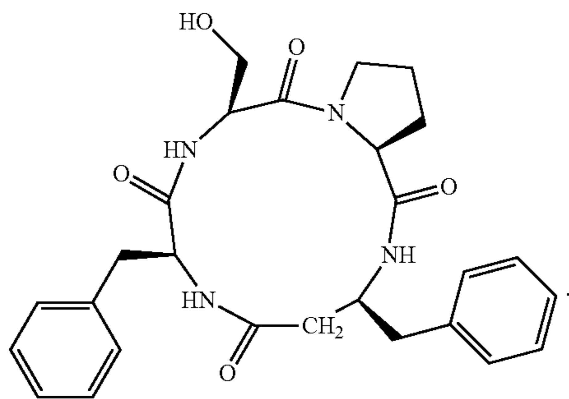
(cyclo(-L-Ser-L-Pro-L-β 3 hoPhe-L-Phe))
