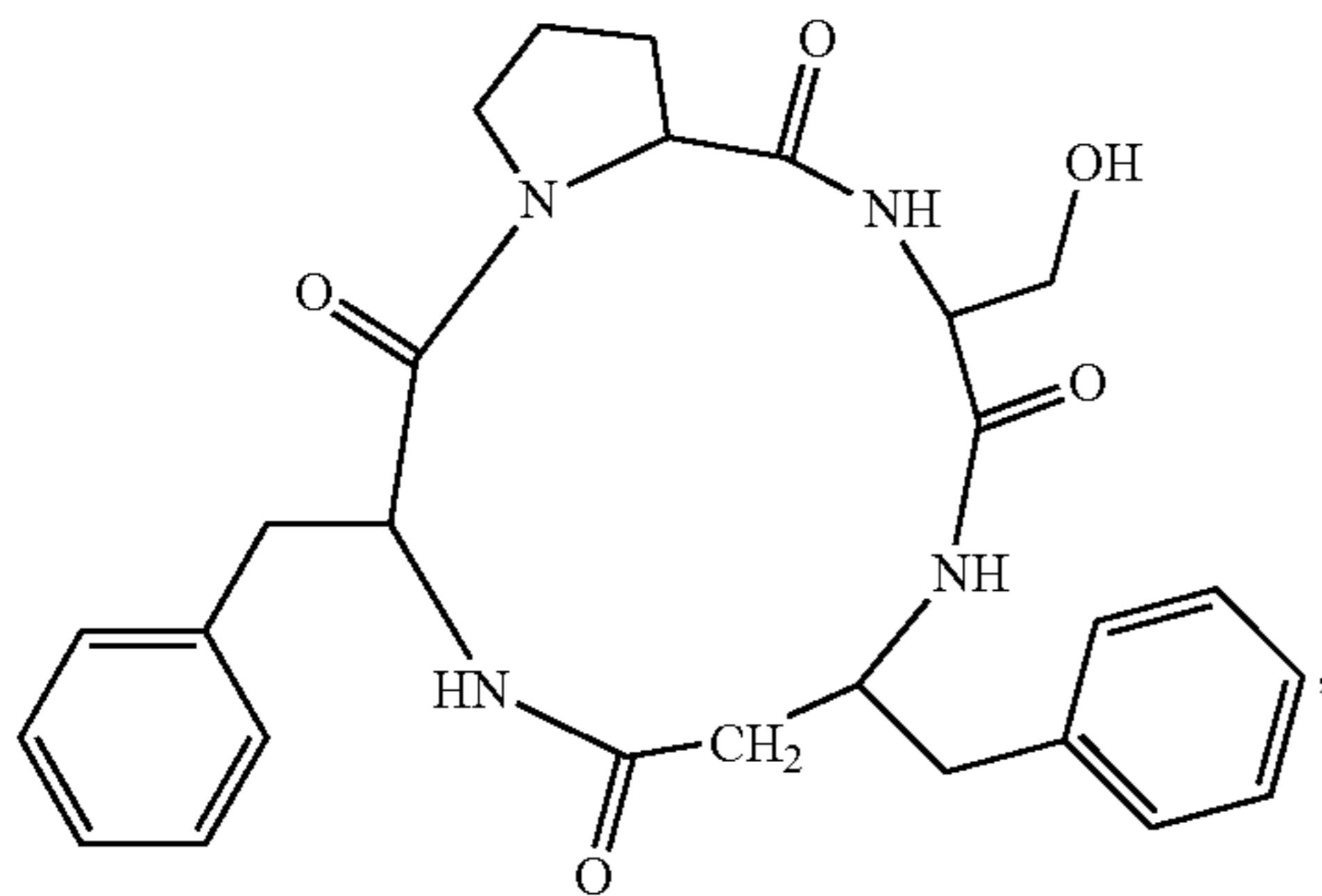
(cyclo(-Pro-Ser-β 3 hoPhe-Phe))
