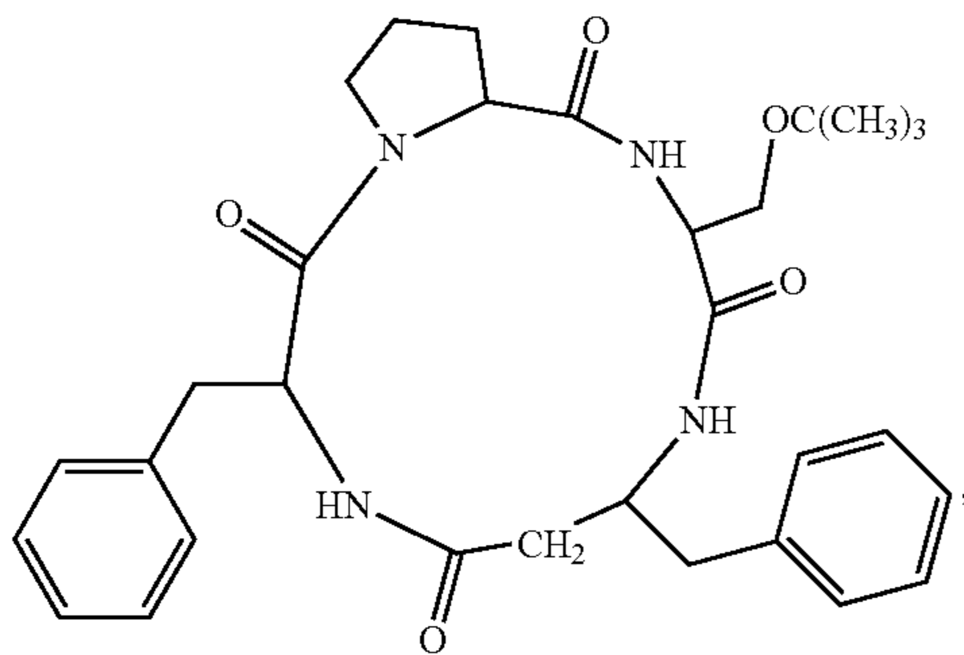
(cyclo(-Pro-Ser(tBu)-β 3 hoPhe-Phe))
