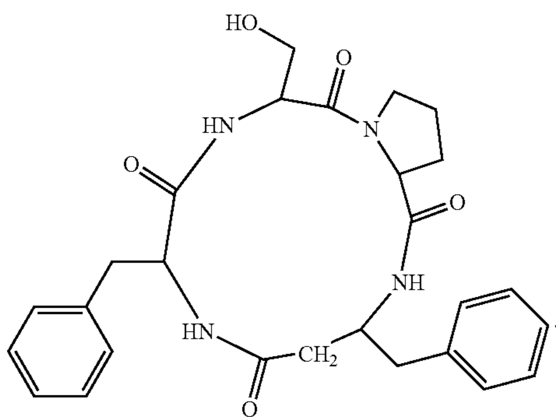
(cyclo(-Ser-Pro-β 3 hoPhe-Phe))
