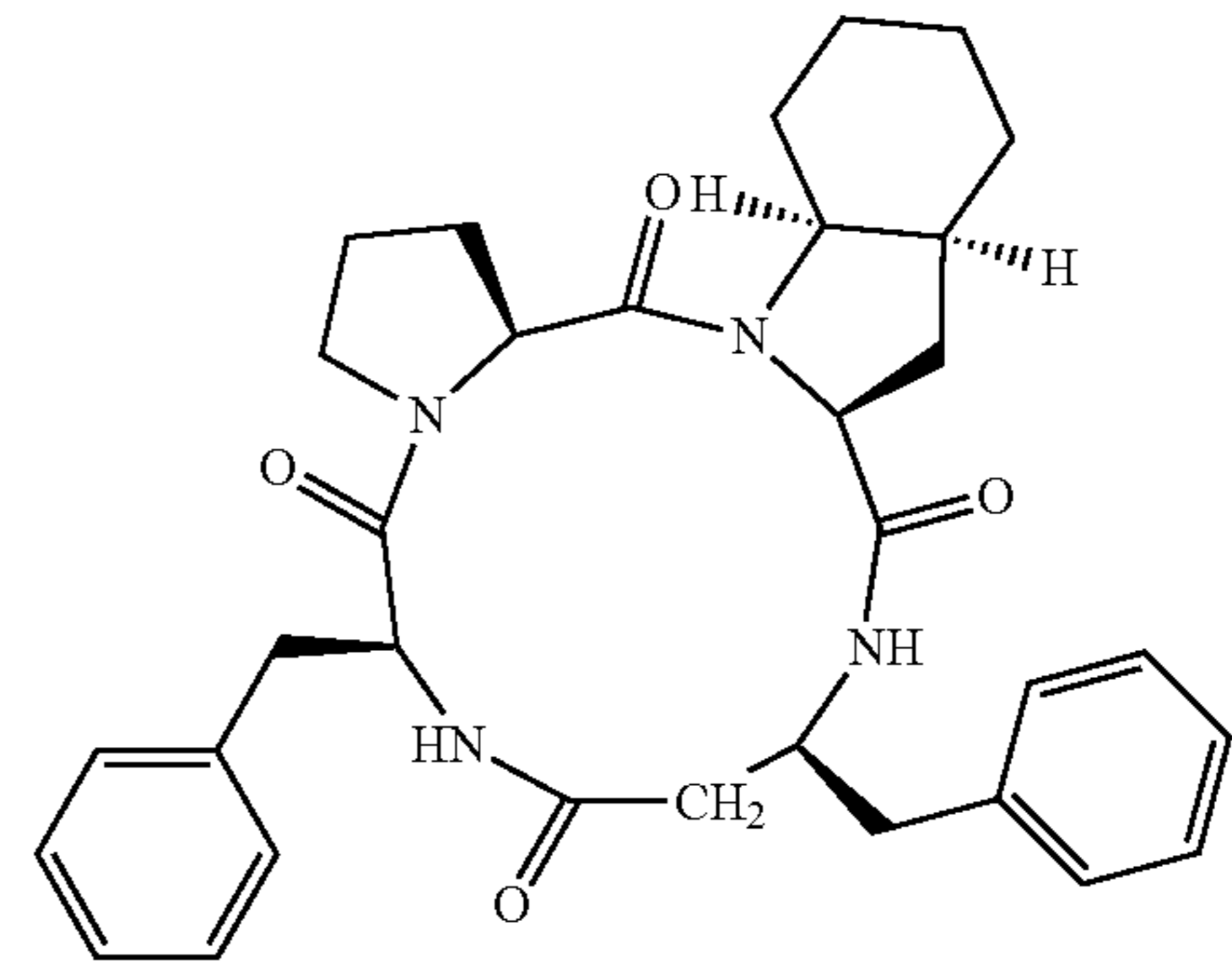
cyclo(-L-Pro-L-Oic-L-β³hoPhe-L-Phe))
