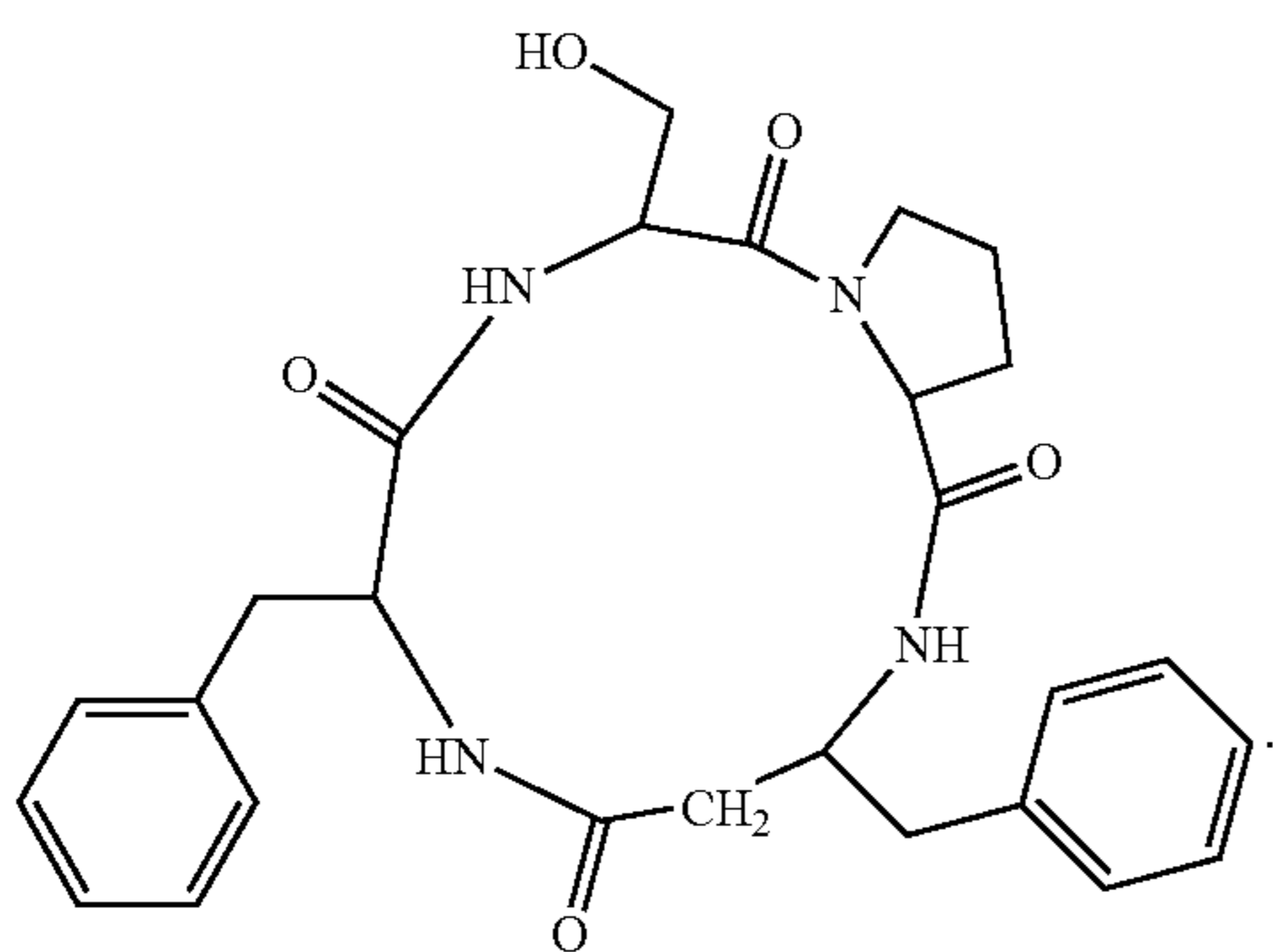
(cyclo(-Ser-Pro-β³hoPhe-Phe))
