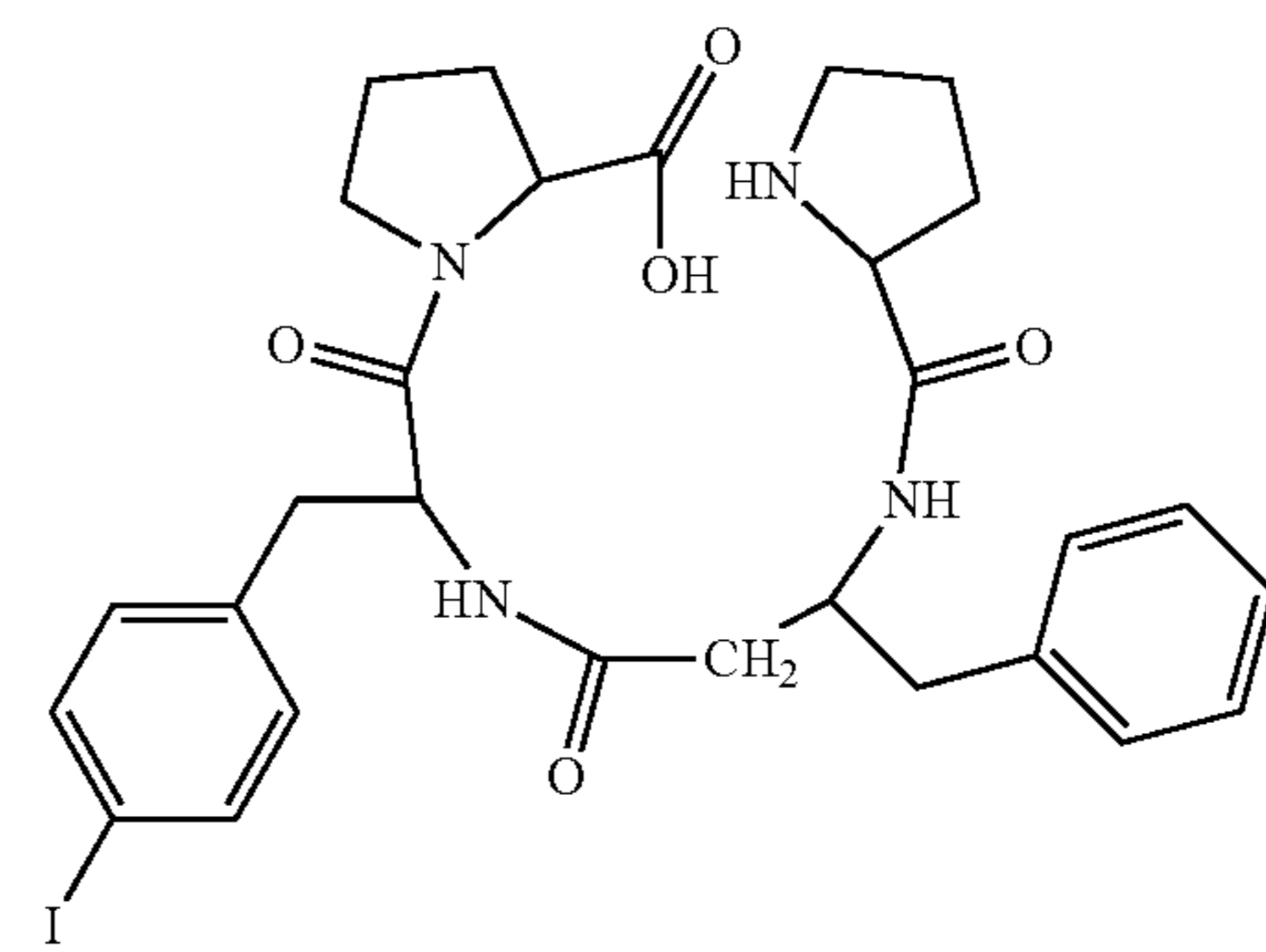
(H-Pro-β 3 hoPhe-Phe(4I)-Pro-OH)
