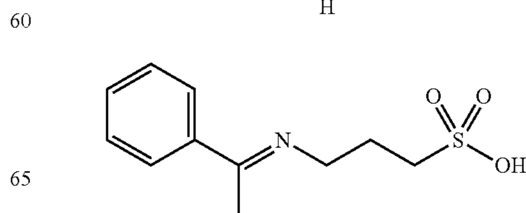
Compound D10
