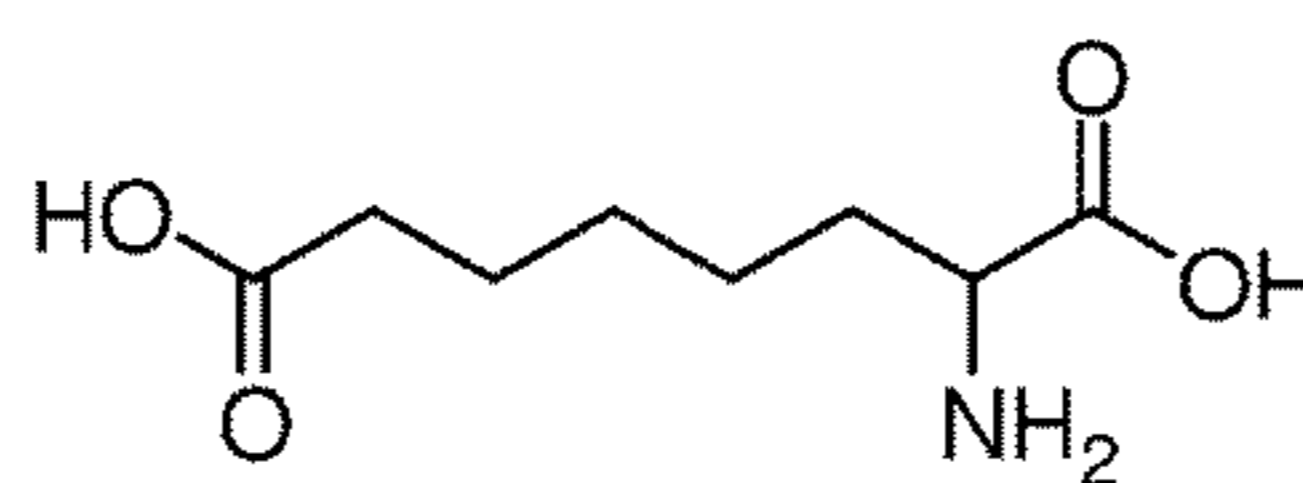
2-Amino-octanedioic acid
