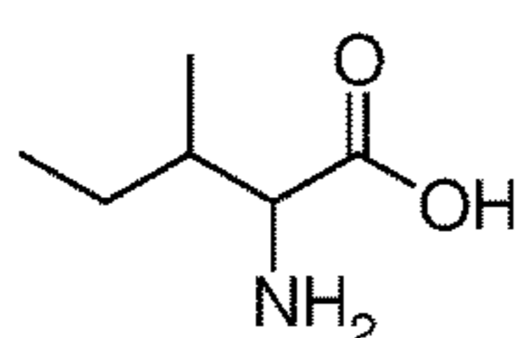
Allo-isoleucine
