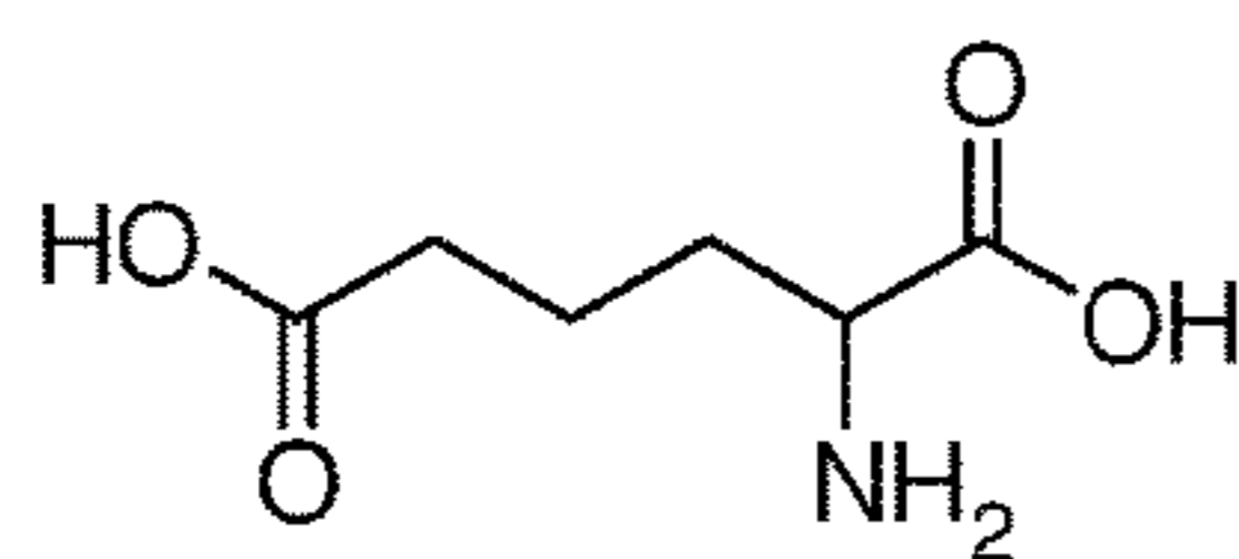
2-Aminoadipic acid
