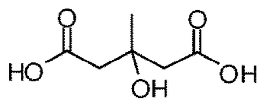
Meglutol
