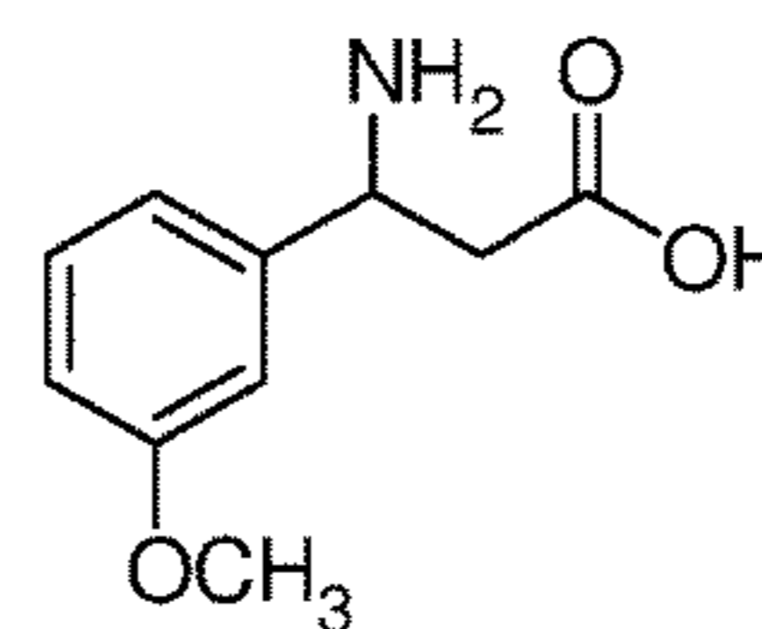
3-Amino-3-(3-methoxyphenyl) propionic acid
