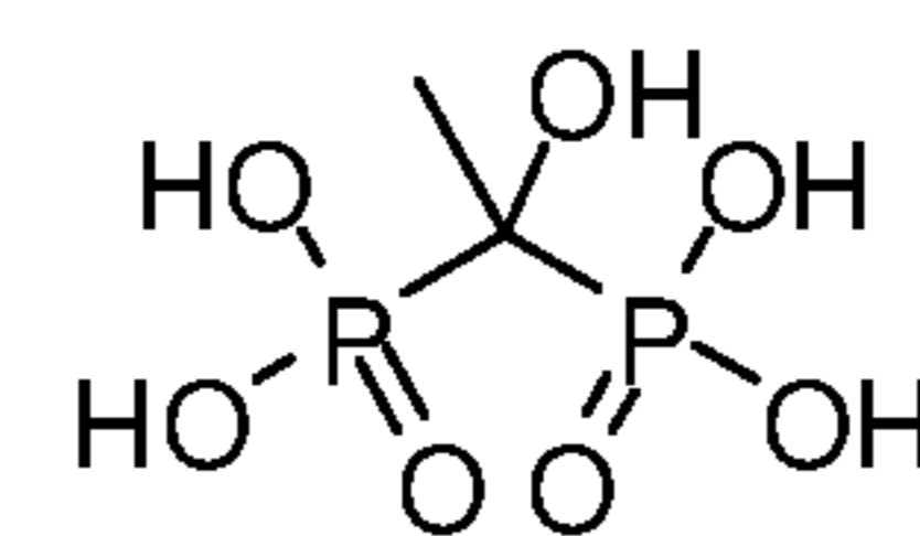
Etidronate
