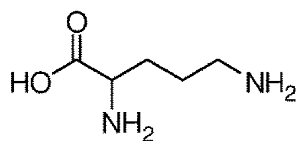
Ornithine
