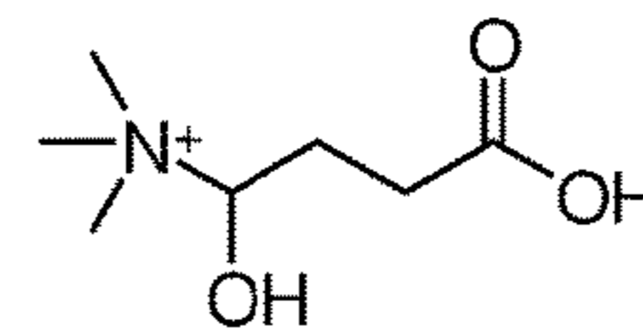
Carnitine
