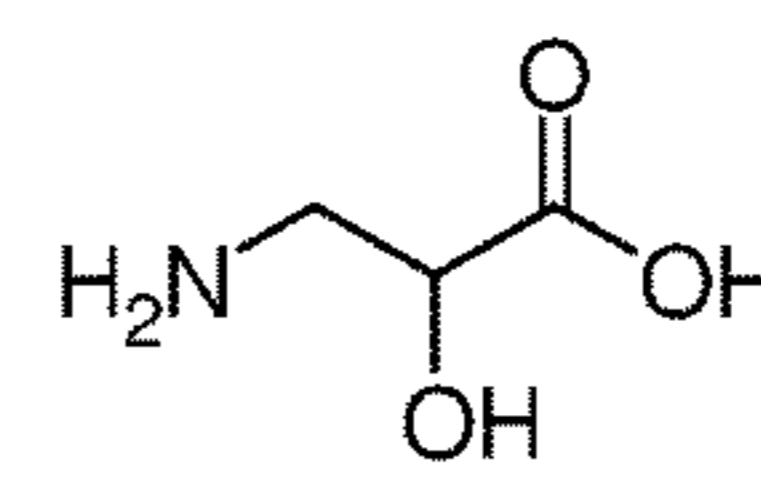
Isoserine
