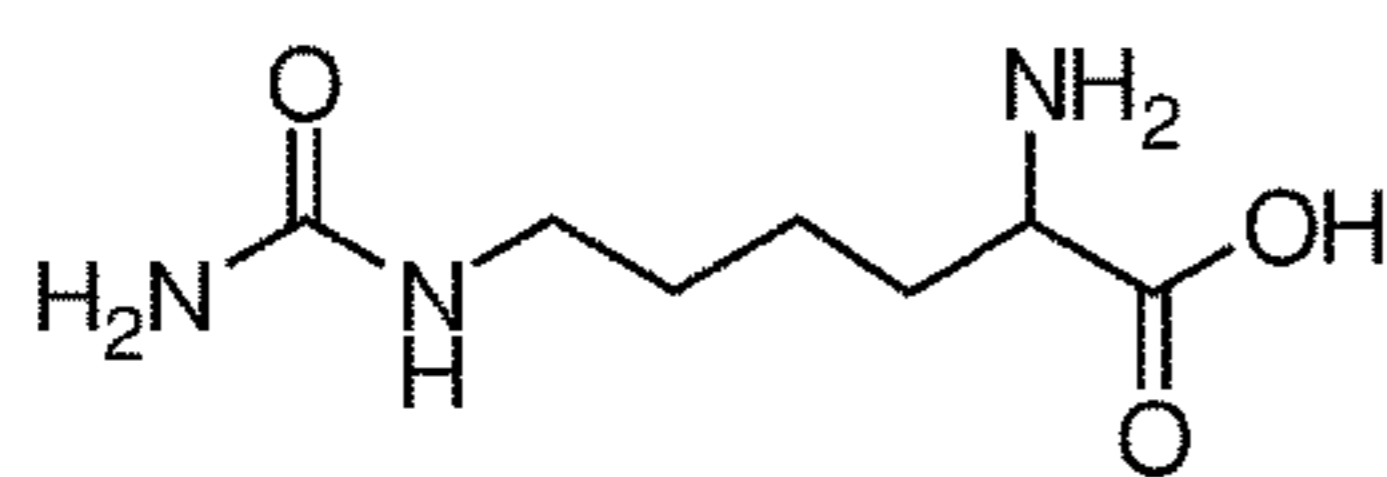
Homocitrulline
