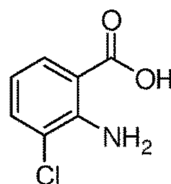
2-Amino-3-chlorobenzoic acid
