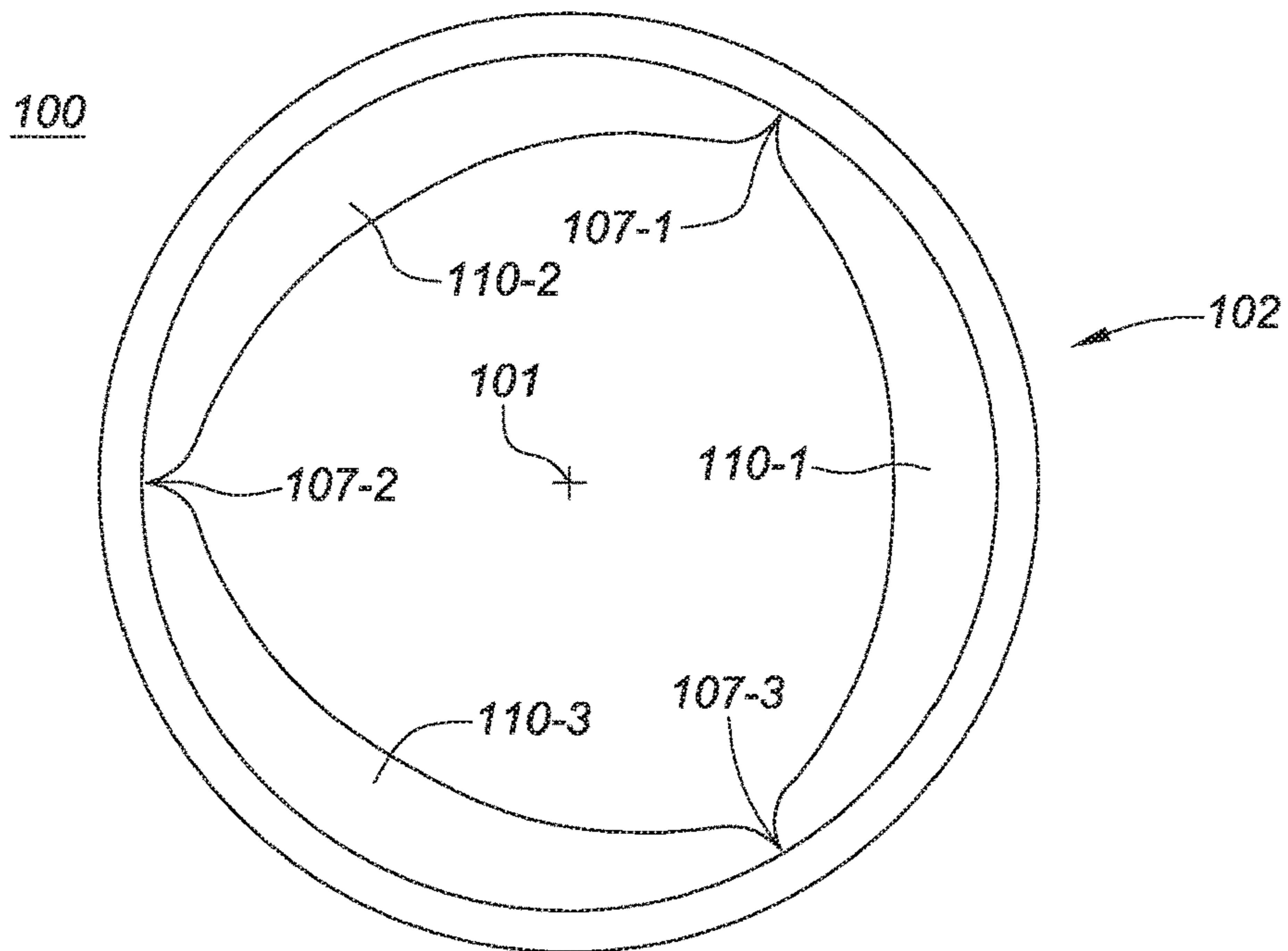
FIG. 2A
