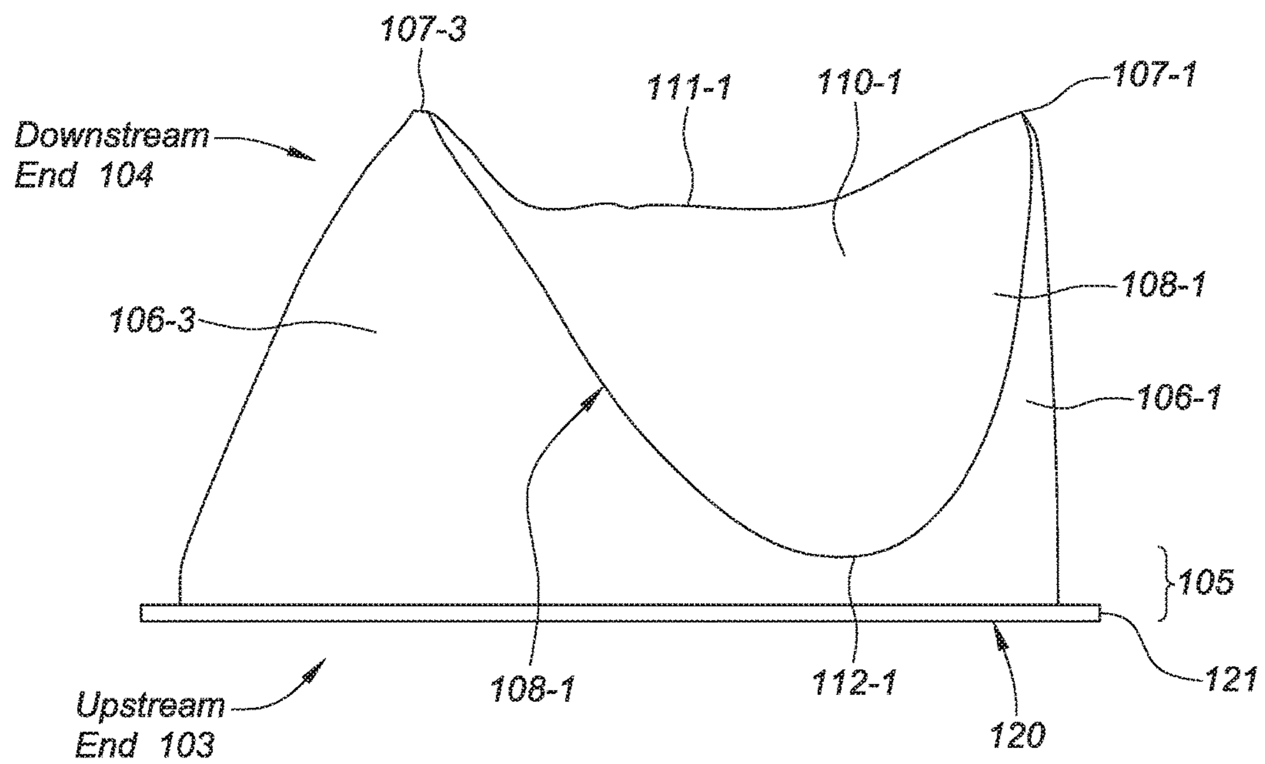
FIG. 3C
