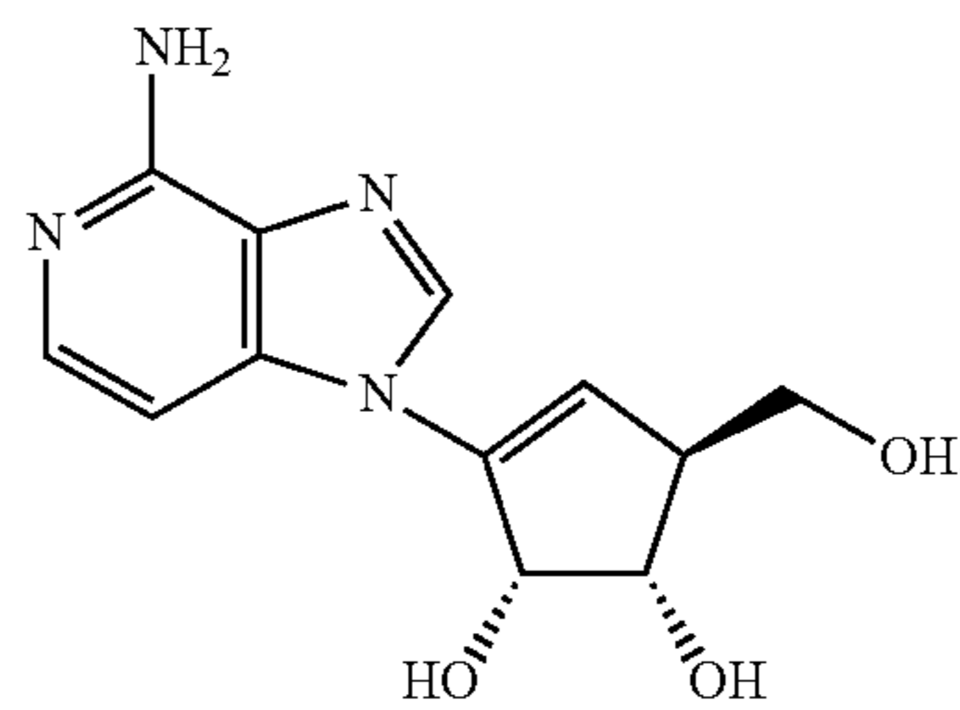
L-3-bromo-3-deazaisoneplanocin
