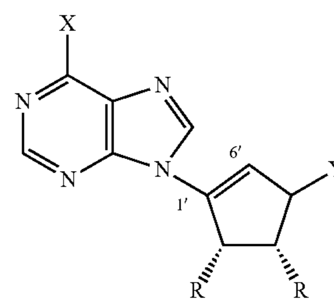
L-isoneplanocin analogue
