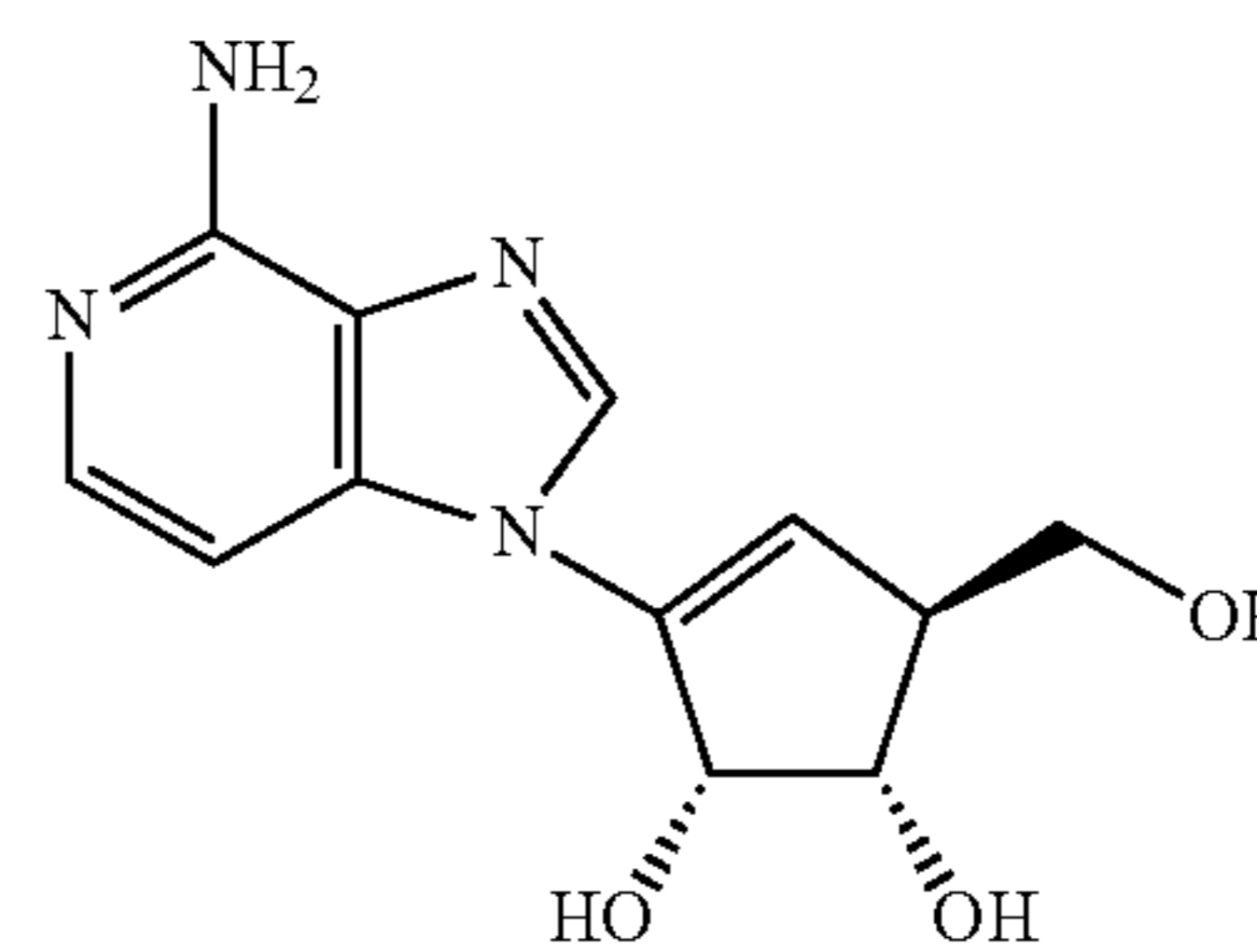
L-3-deazaisoneplanocin
