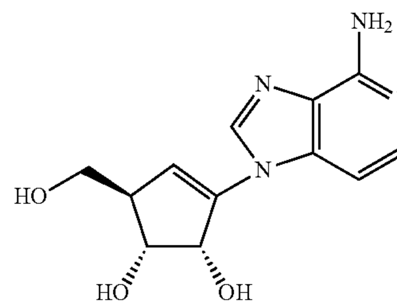
D-3-bromo-3-deazaisoneplanocin
