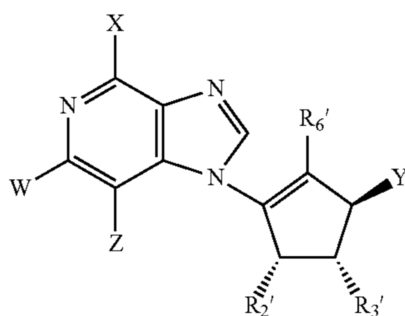
L-3-Deazaisoneplanocin analogue
