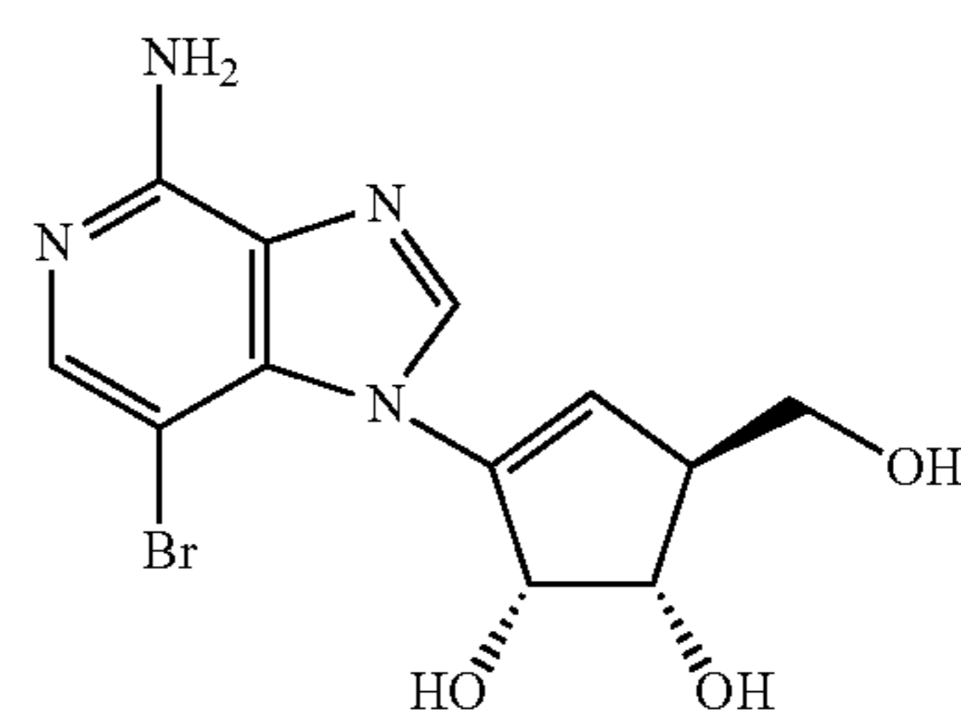
L-3-deazaisoneplanocin
