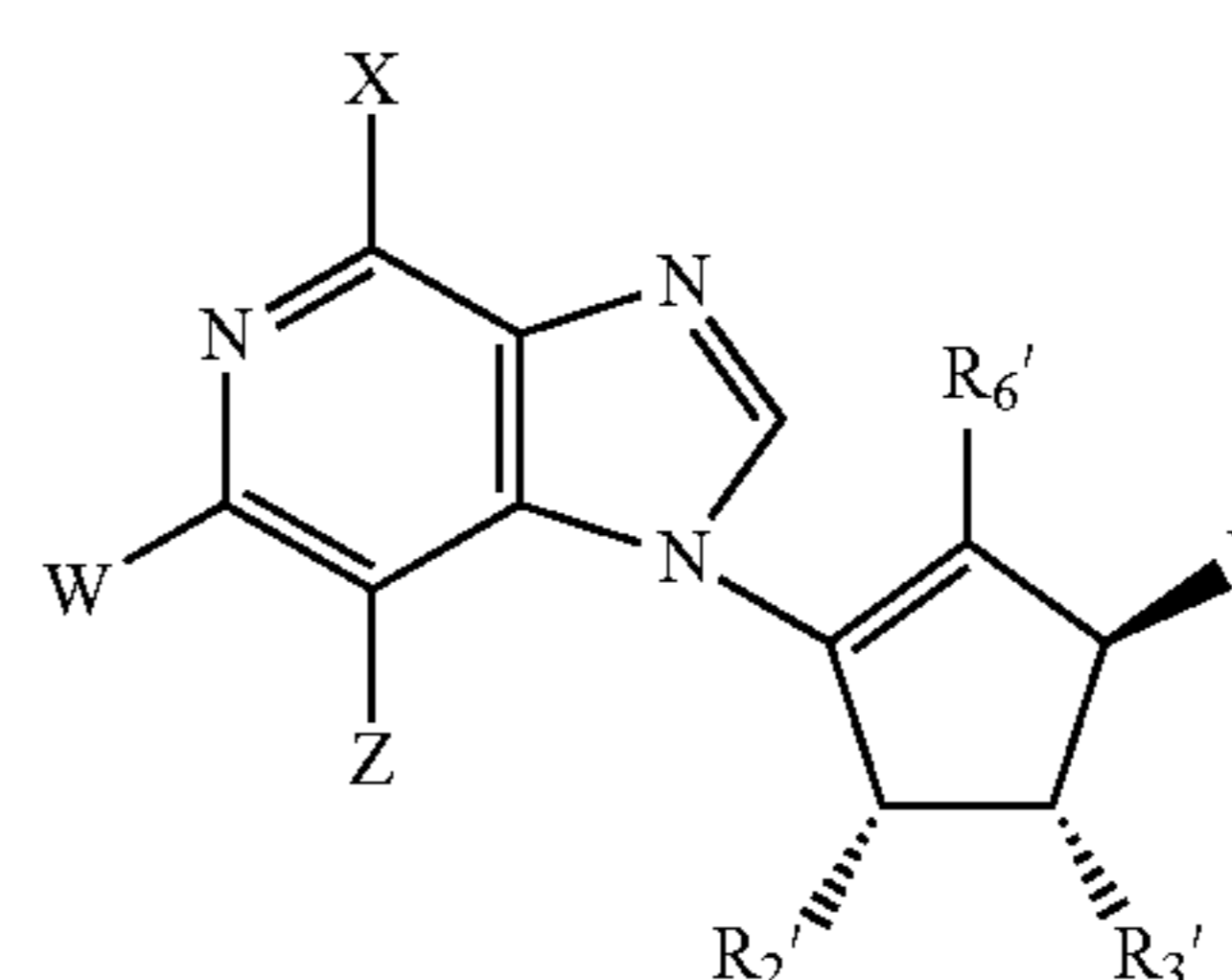
L-3-Deazaisoneplanocin analogue
