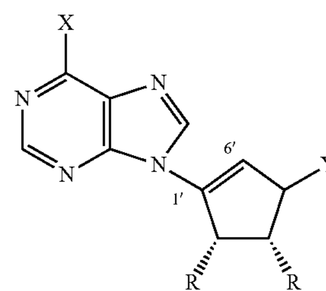
L-isoneplanocin analogue
