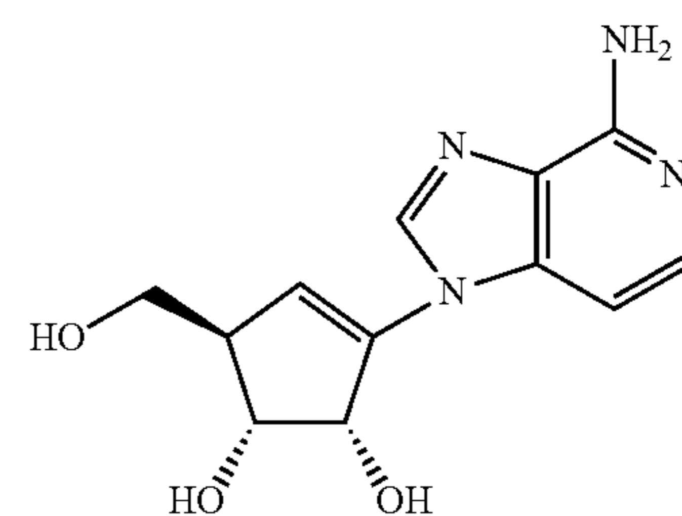
D-3-deazaisoneplanocin
