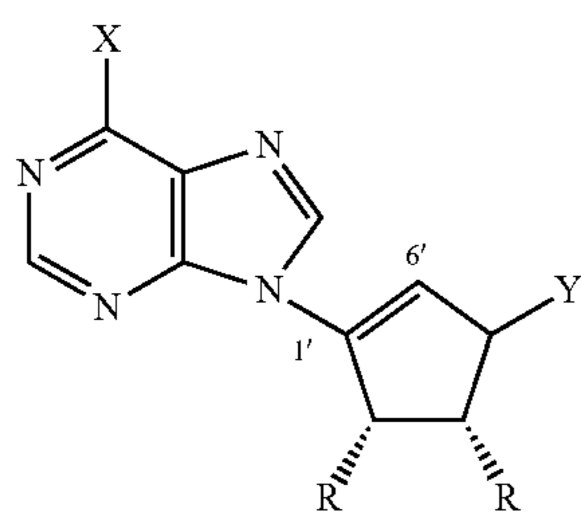
L-isoneplanocin analogue
