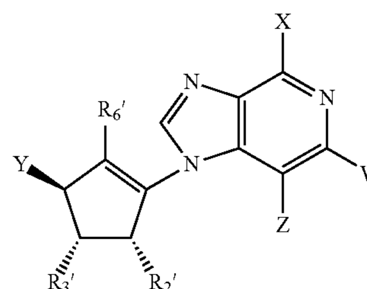
D-3-Deazaisoneplanocin analogue
