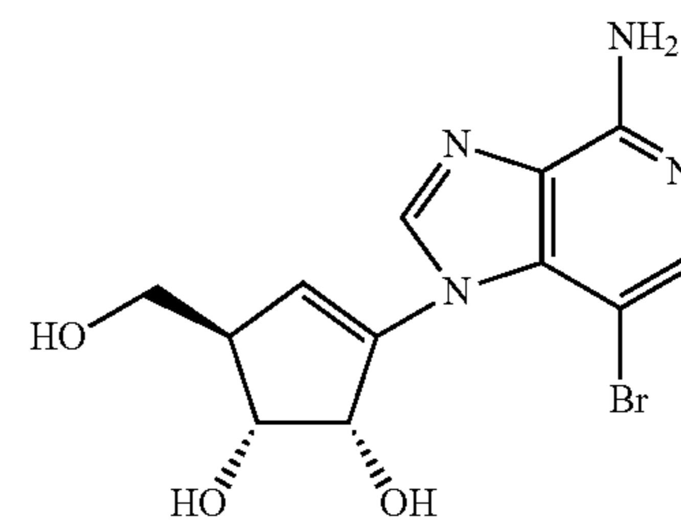
D-3-deazaisoneplanocin
