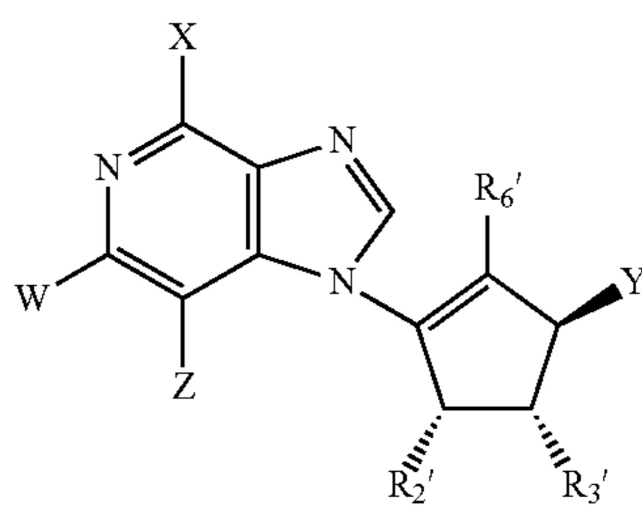
L-3-Deazaisoneplanocin analogue
