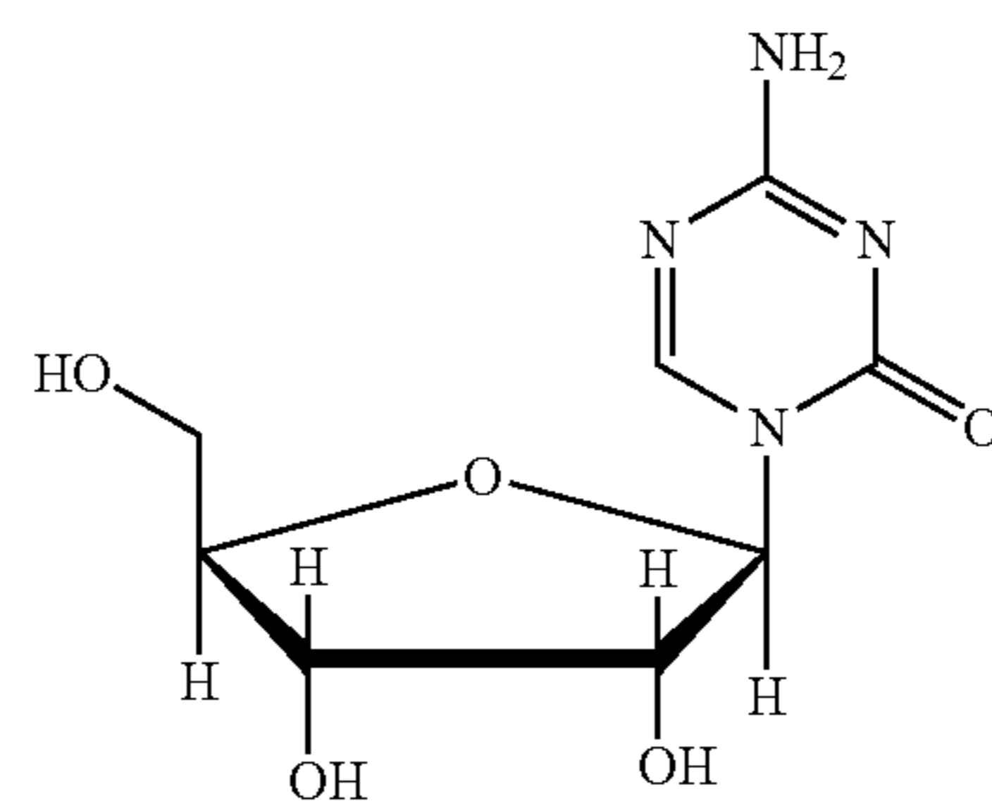
5-Azacytidine
