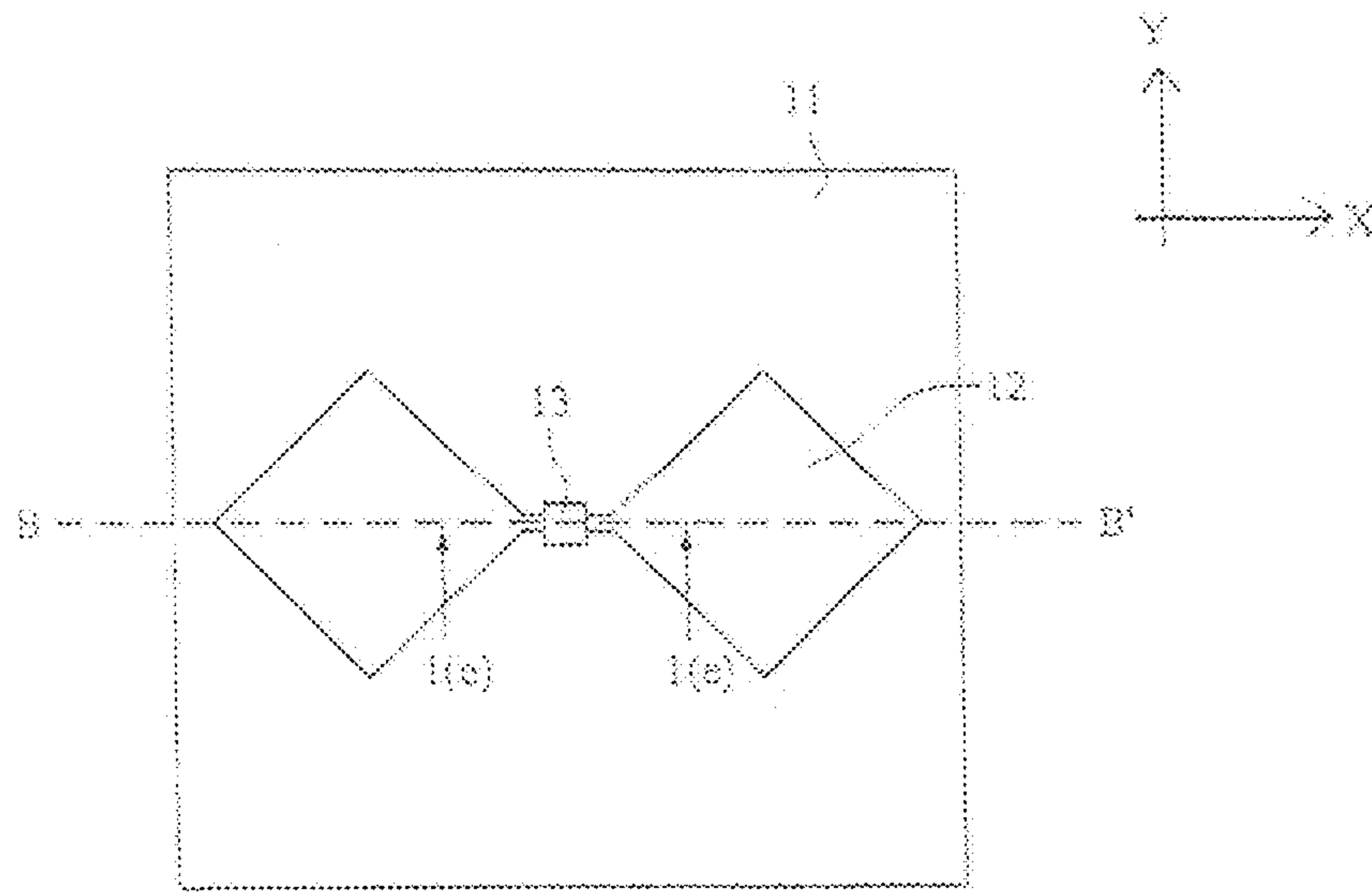
FIG. 1(d) (Related Art)
