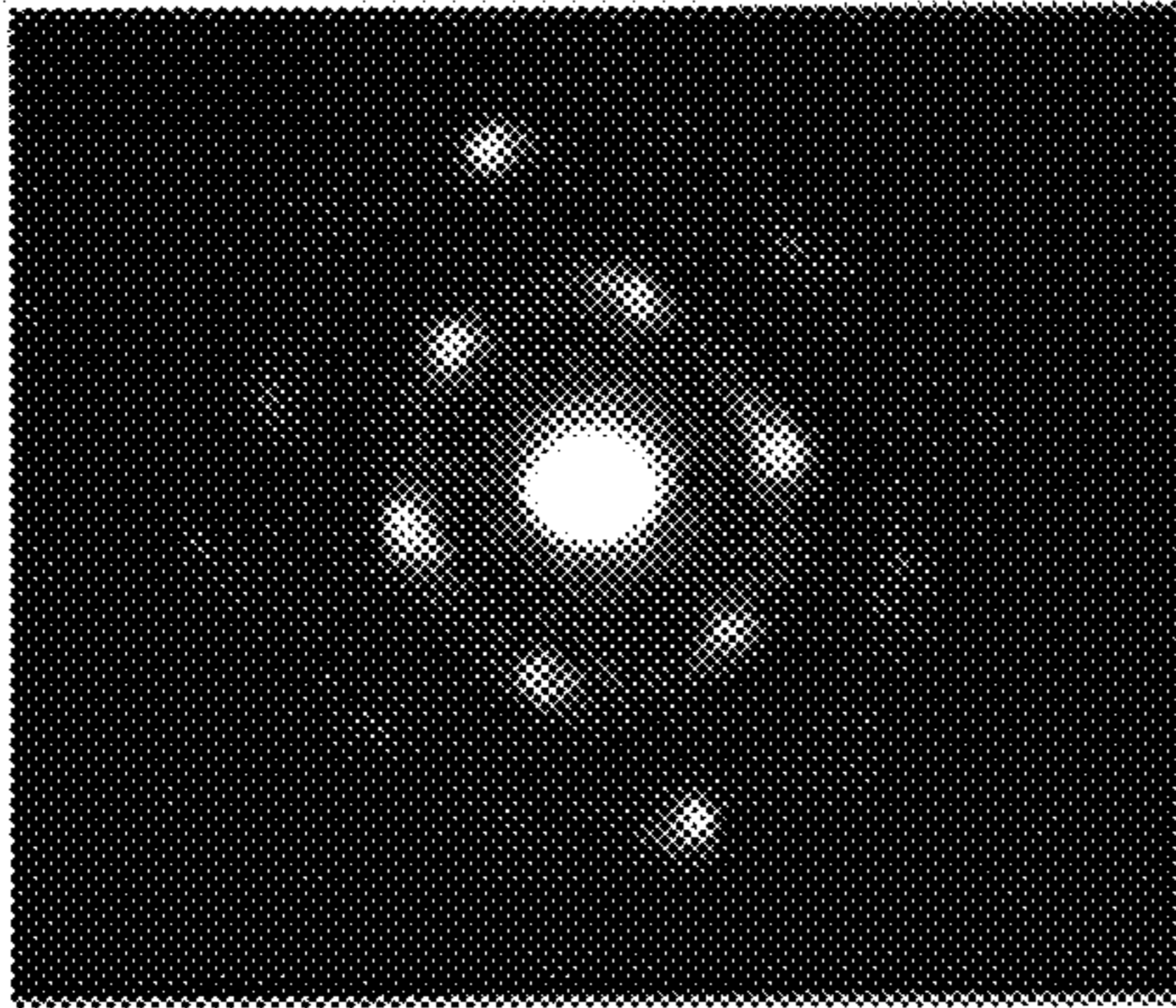
CAAC-OS
