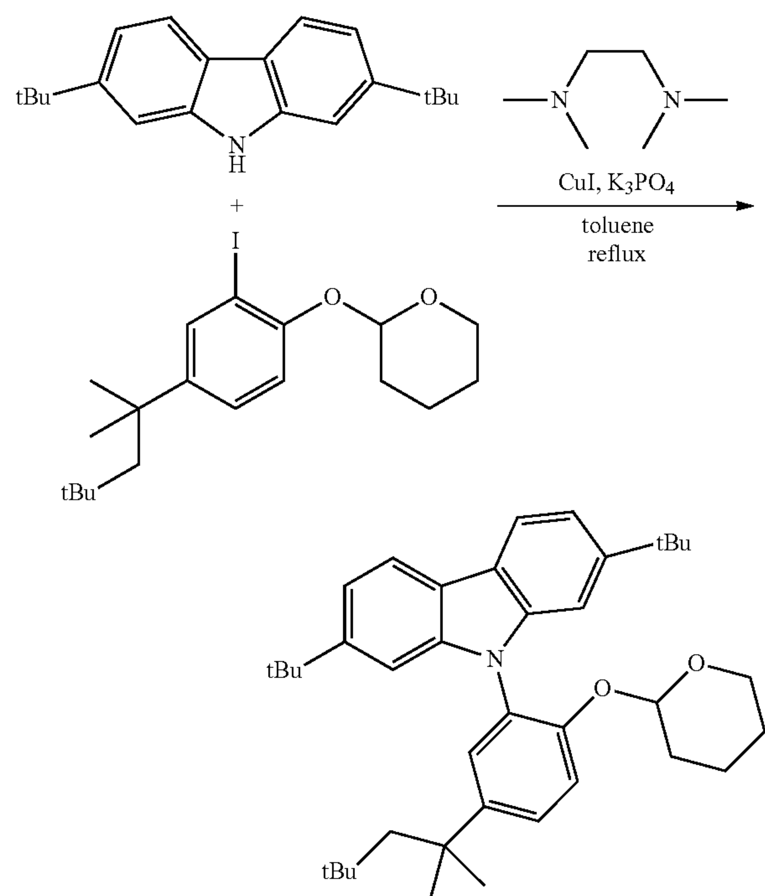
Preparation of 2,7-di-tert-butyl-9-(2-((tetrahydro-2H-pyran-2-yl)oxy)-5-(2,4,4-trimethylpentan-2-yl)phenyl)-9H-carbazole
