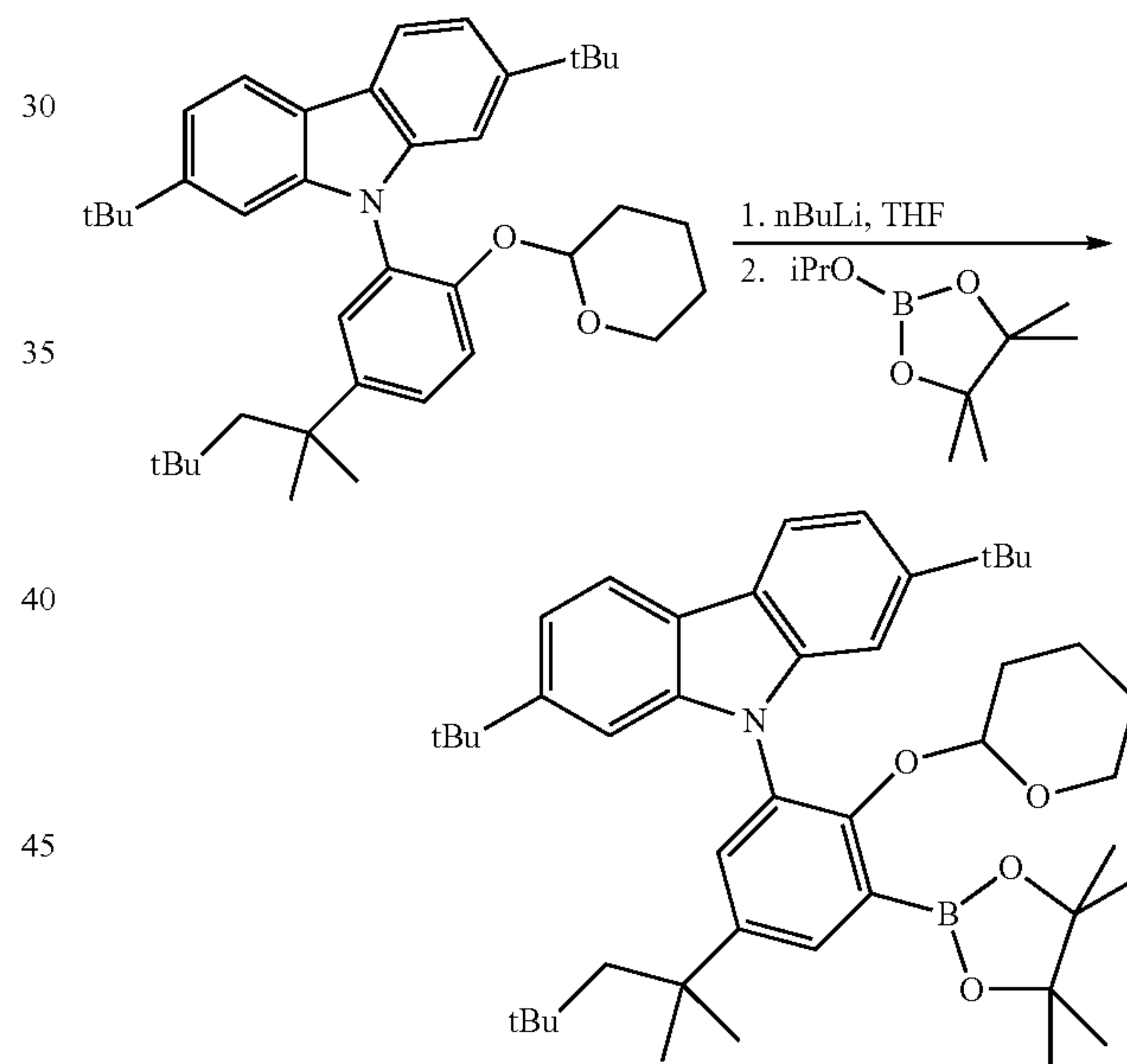
Preparation of 2,7-di-tert-butyl-9-(2-((tetrahydro-2H-pyran-2-yl)oxy)-3-(4,4,5,5-tetramethyl-1,3,2-dioxaborolan-2-yl)-5-(2,4,4-trimethylpentan-2-yl)phenyl)-9H-carbazole
