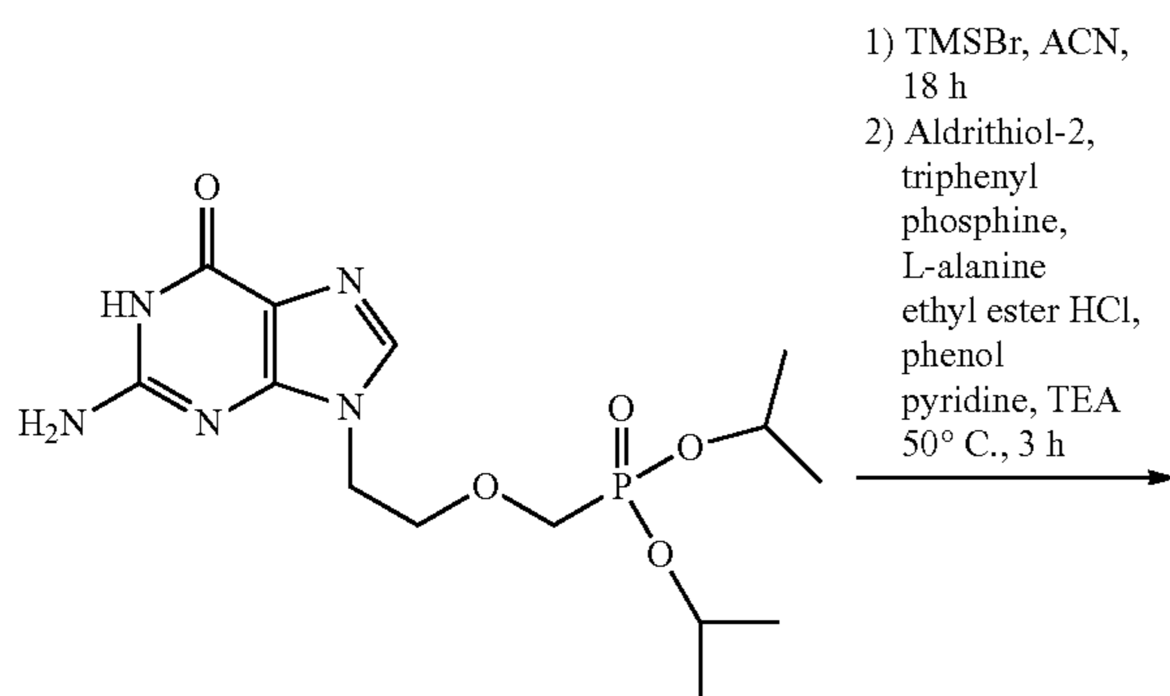
diisopropyl PMEG
