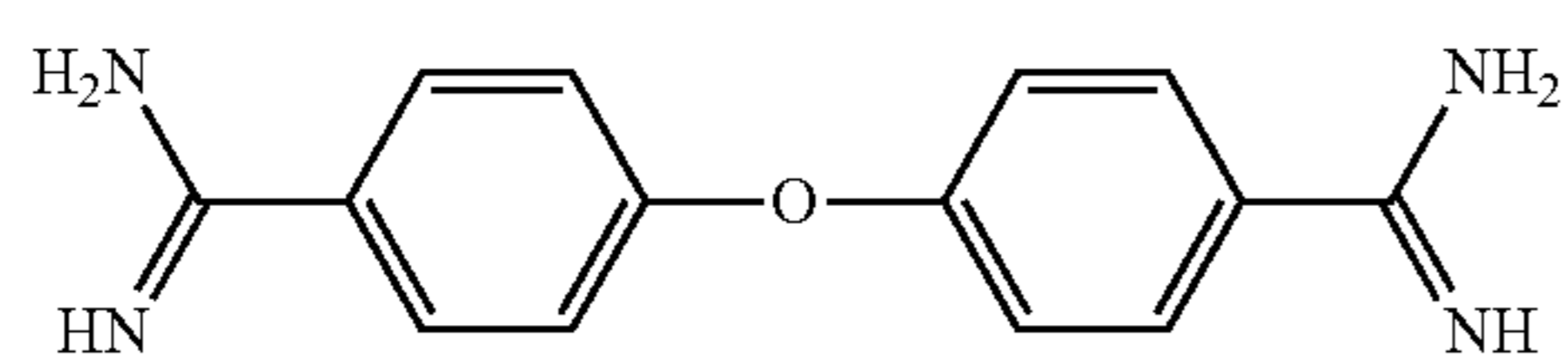
4,4'-oxy-bis-benzamidine
