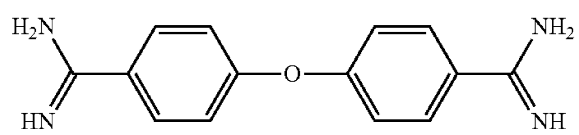
4,4'-oxy-bis-benzamidine
