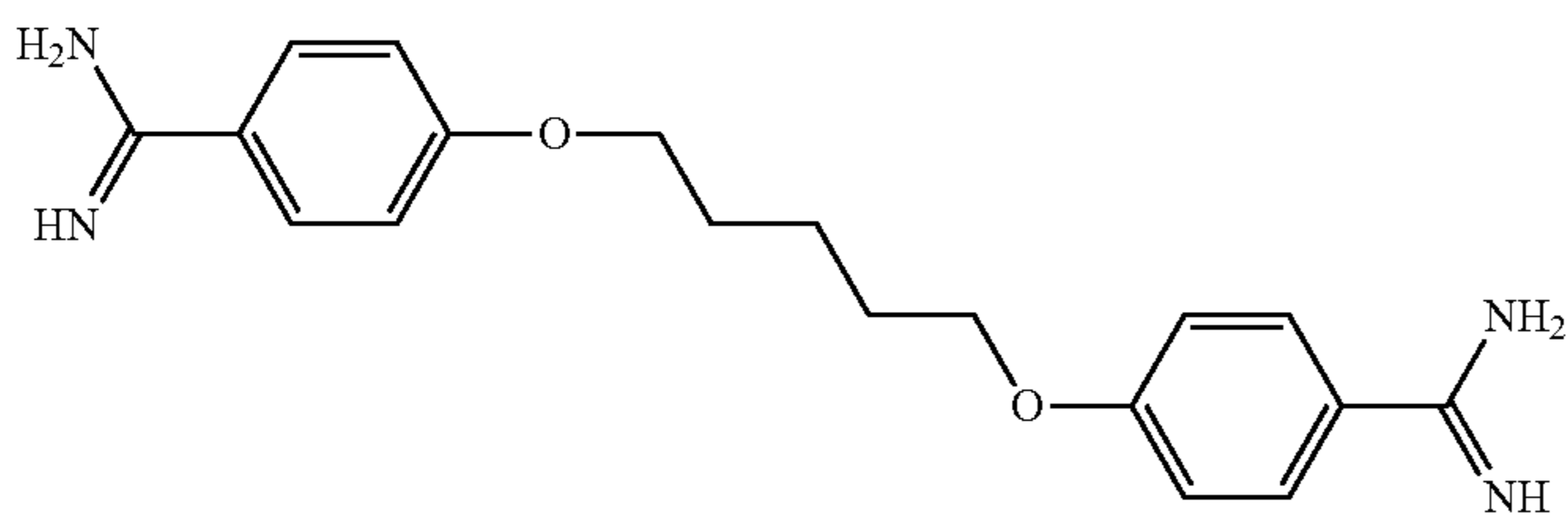
4,4'-pentanediyldioxy-bis-benzamidine
