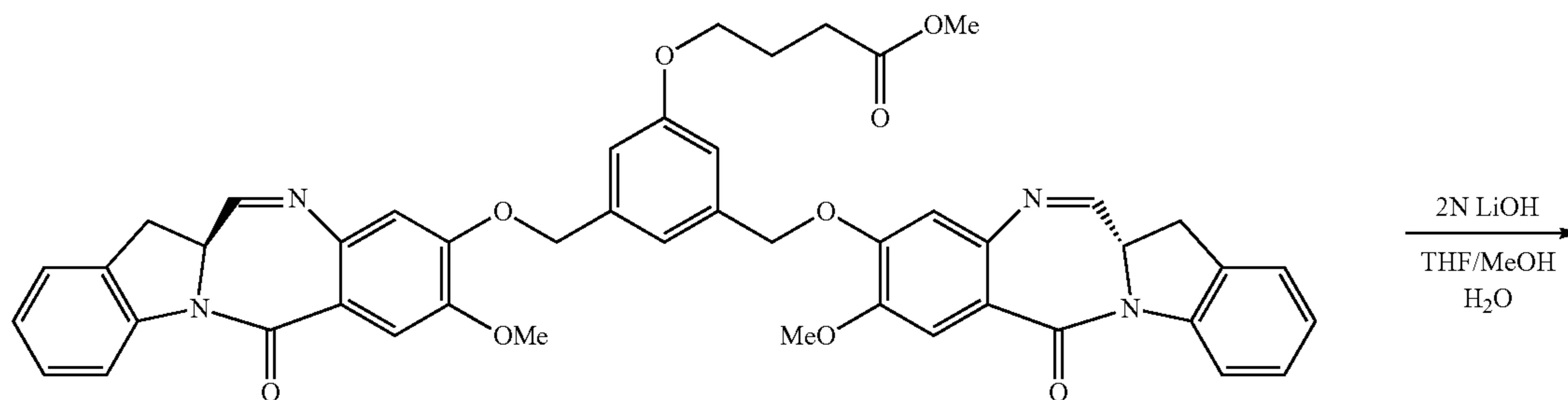
35 (IGN-04)
