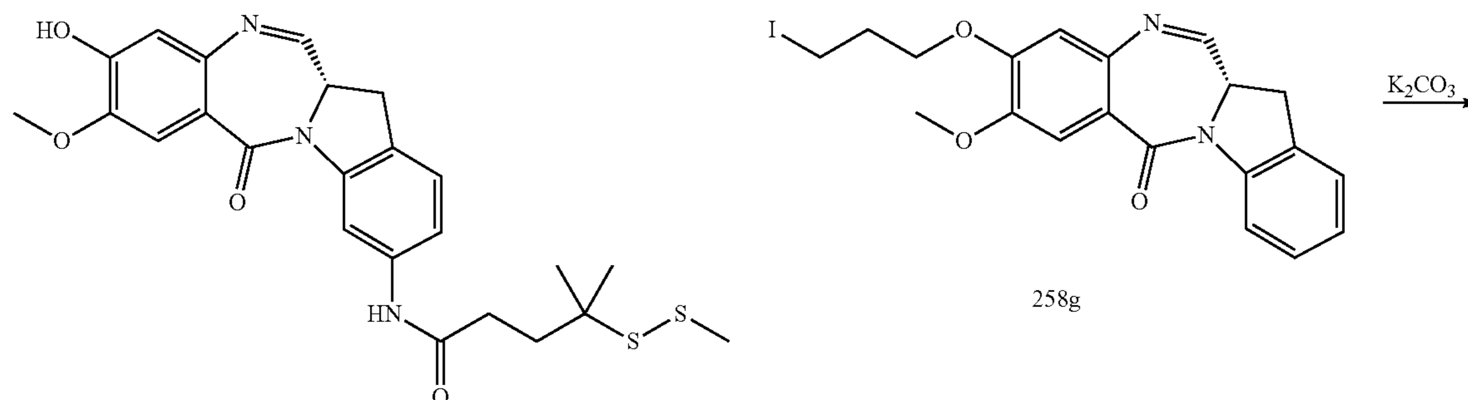
258f
