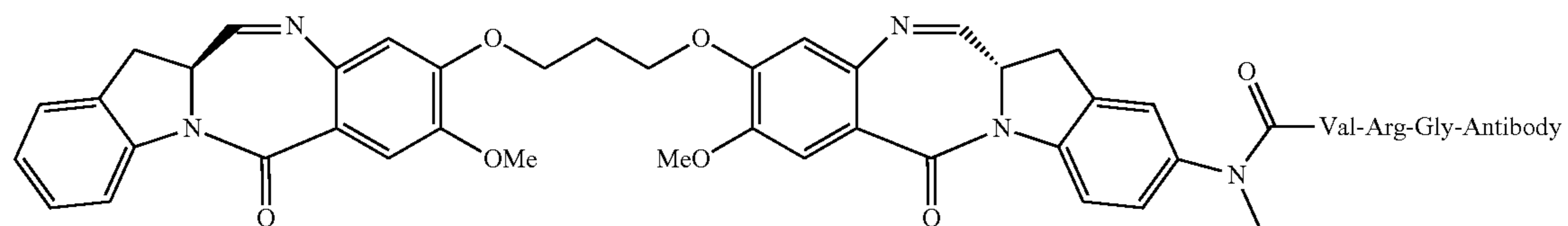
Dimer 6
