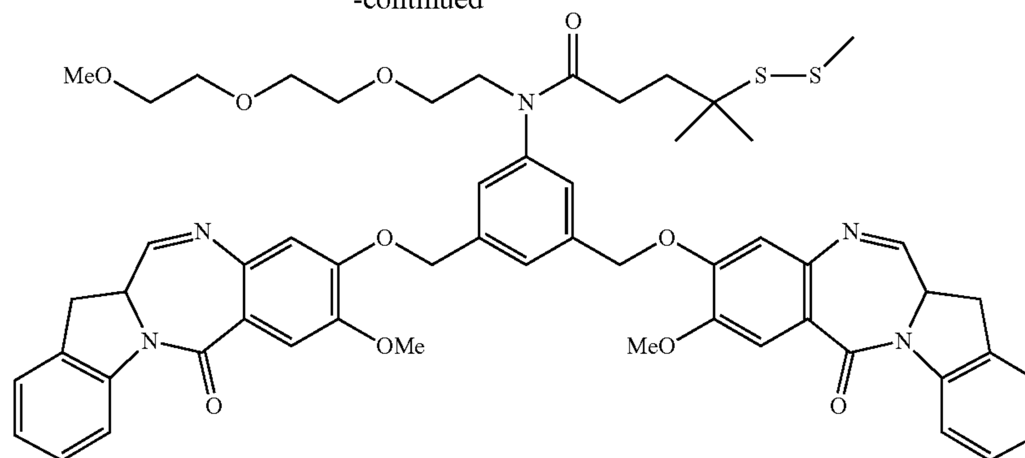
267d
