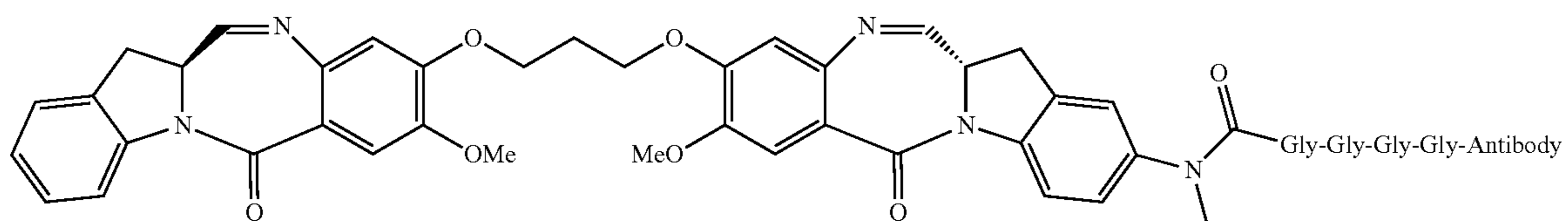
Dimer 5
