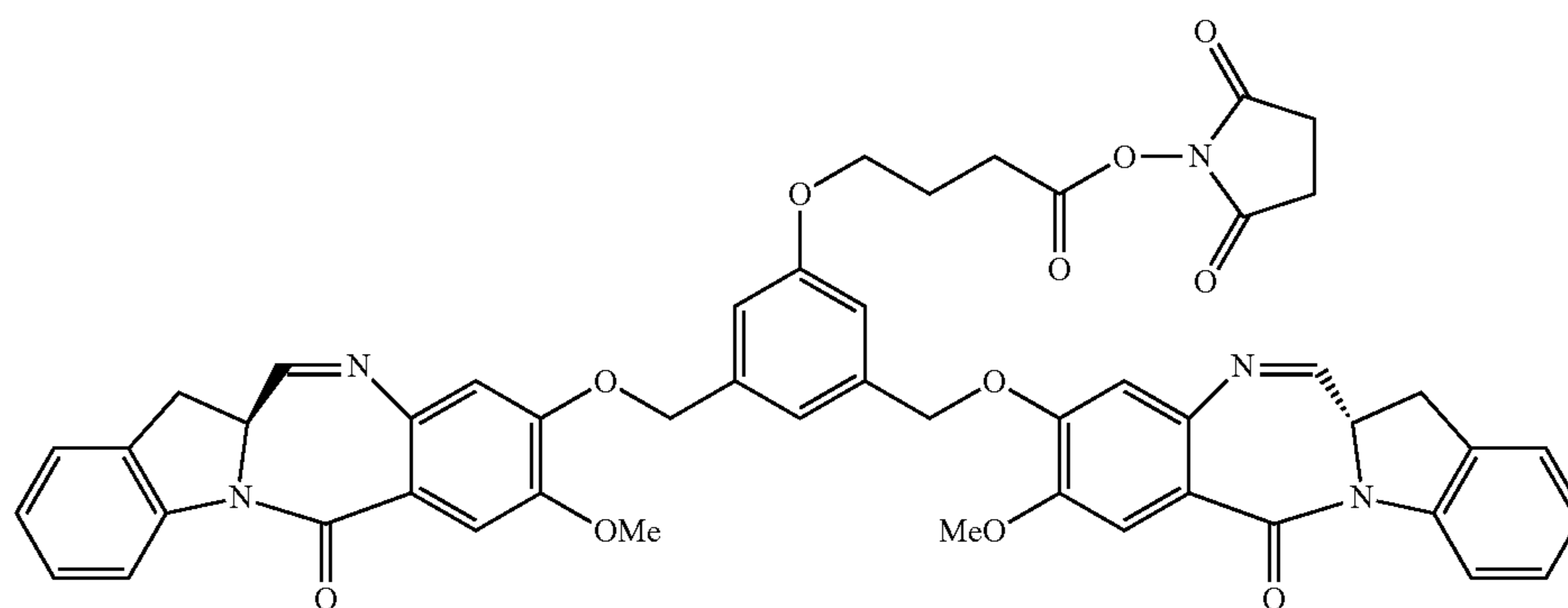
44 (IGN-04 NHS ester)
