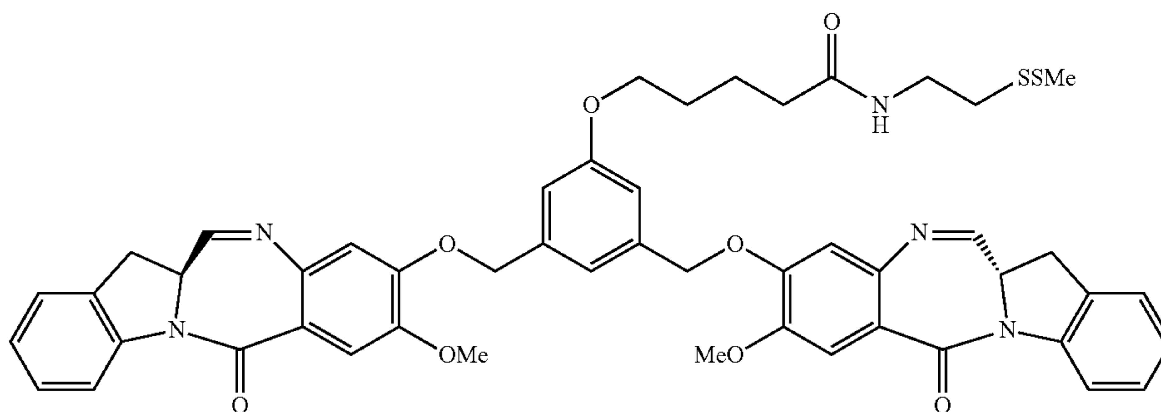
48 (IGN-08)
