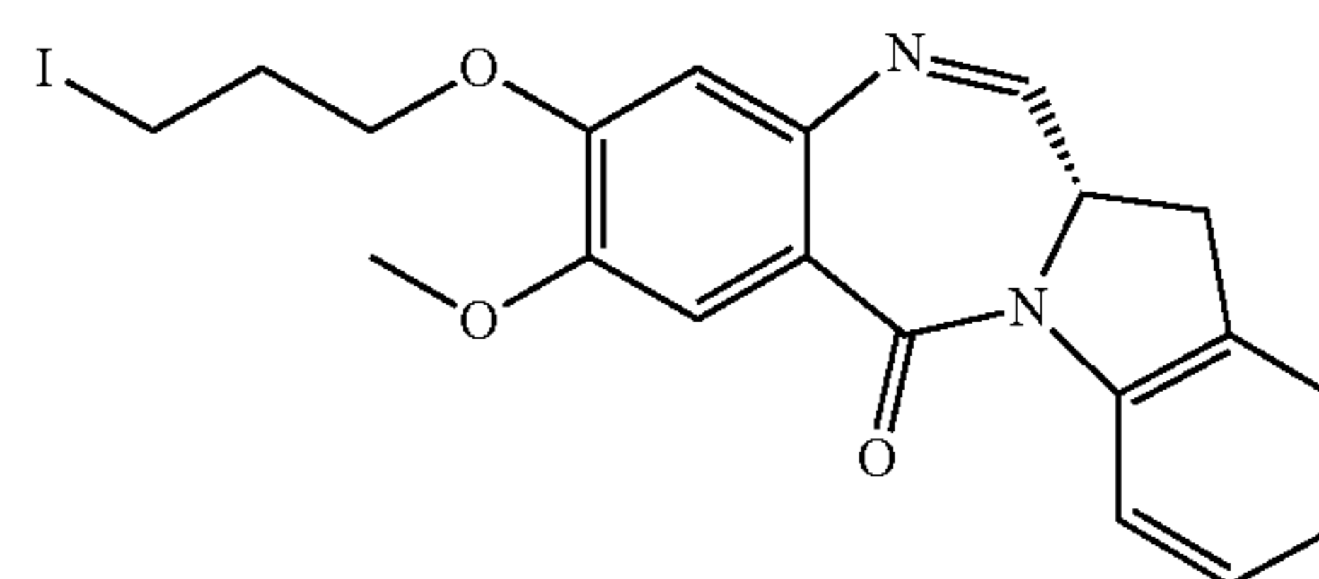
258g
