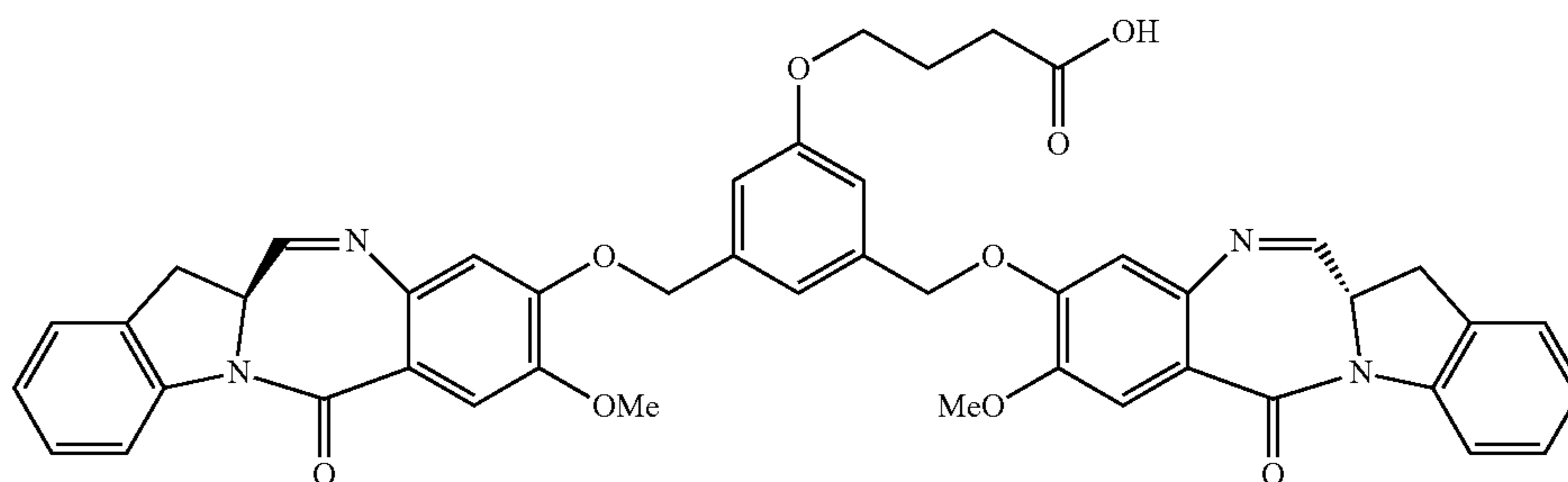
42 (IGN-04 acid)
