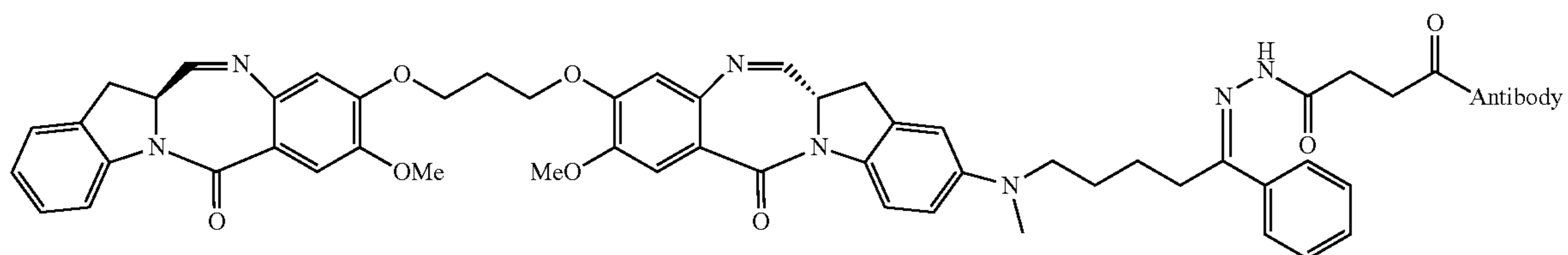
Dimer 8
