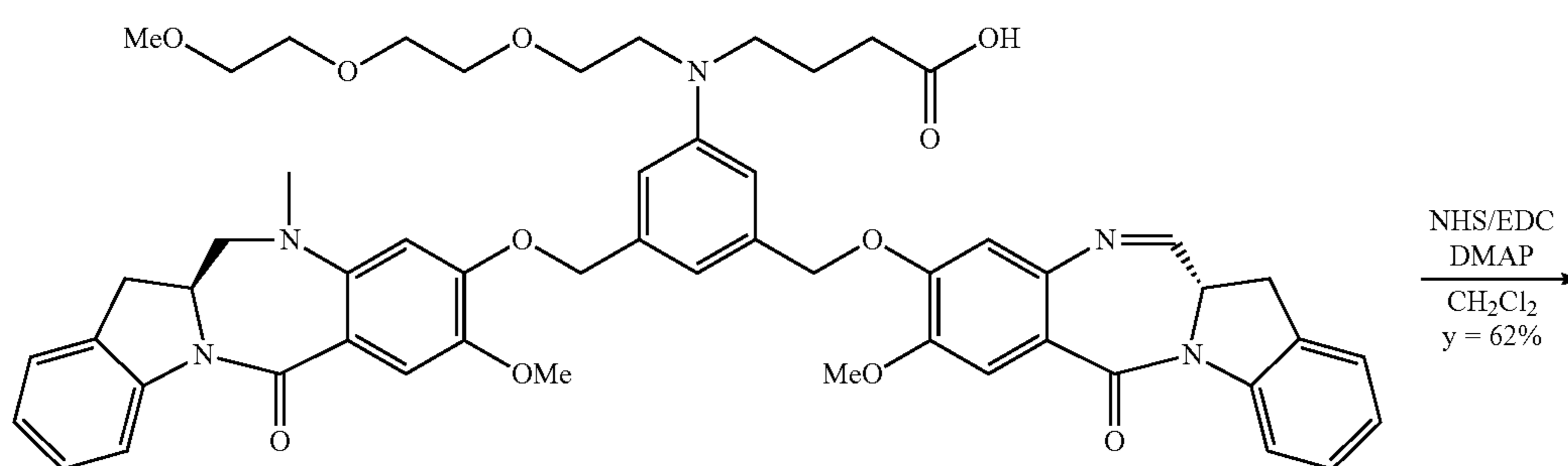
256f
