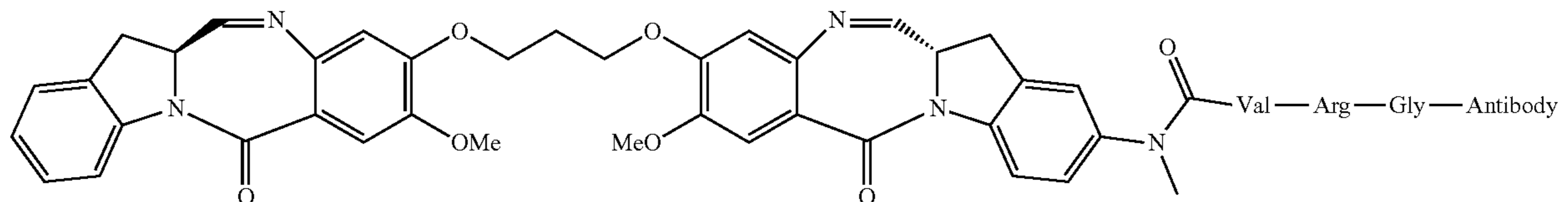
Dimer 7
