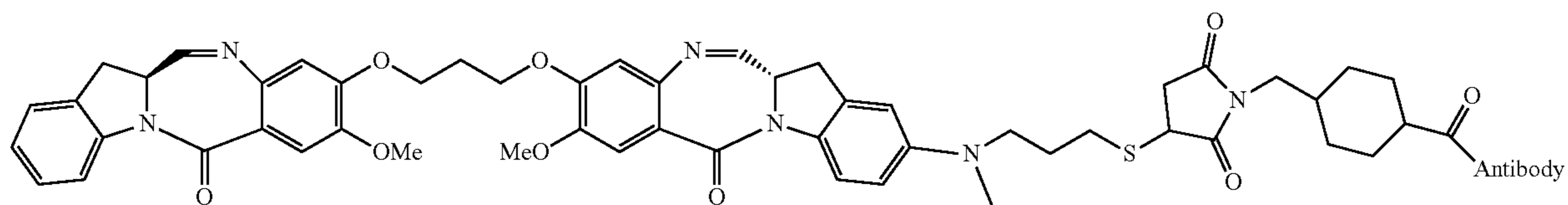
Dimer 8
