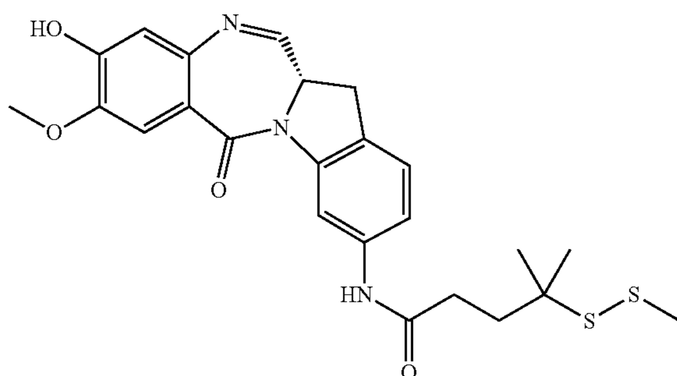
258f
