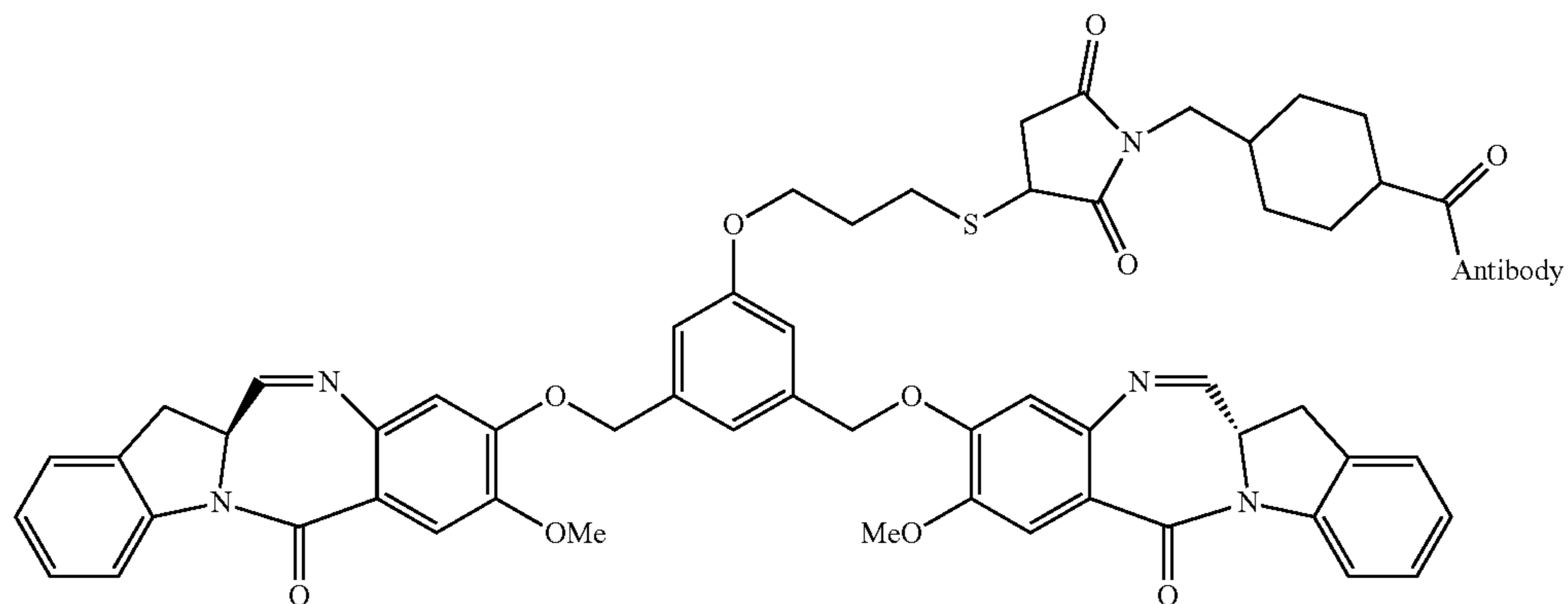
Dimer 3
