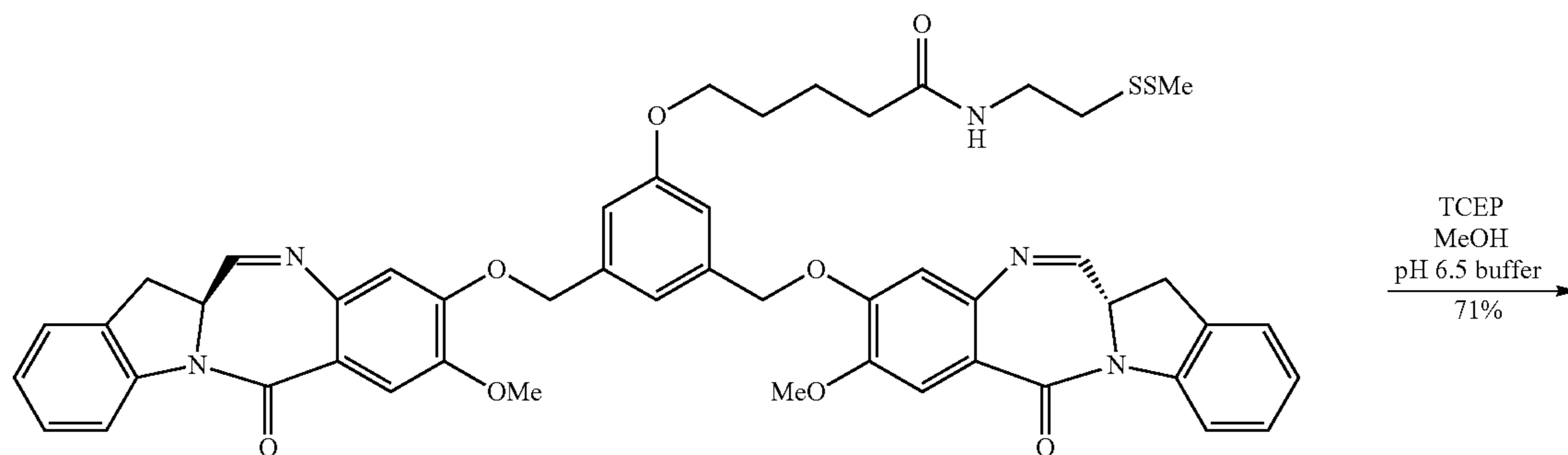
48 (IGN-08)
