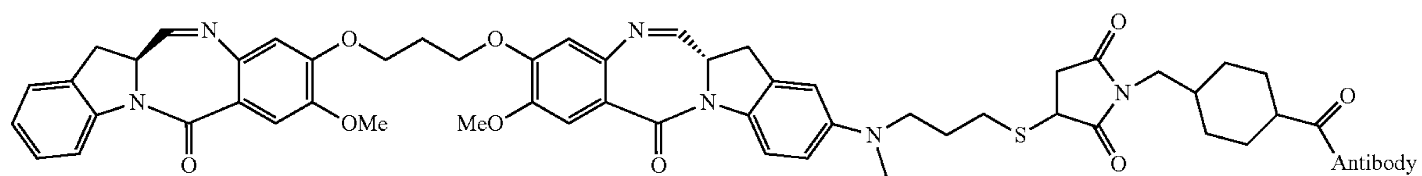
Dimer 7
