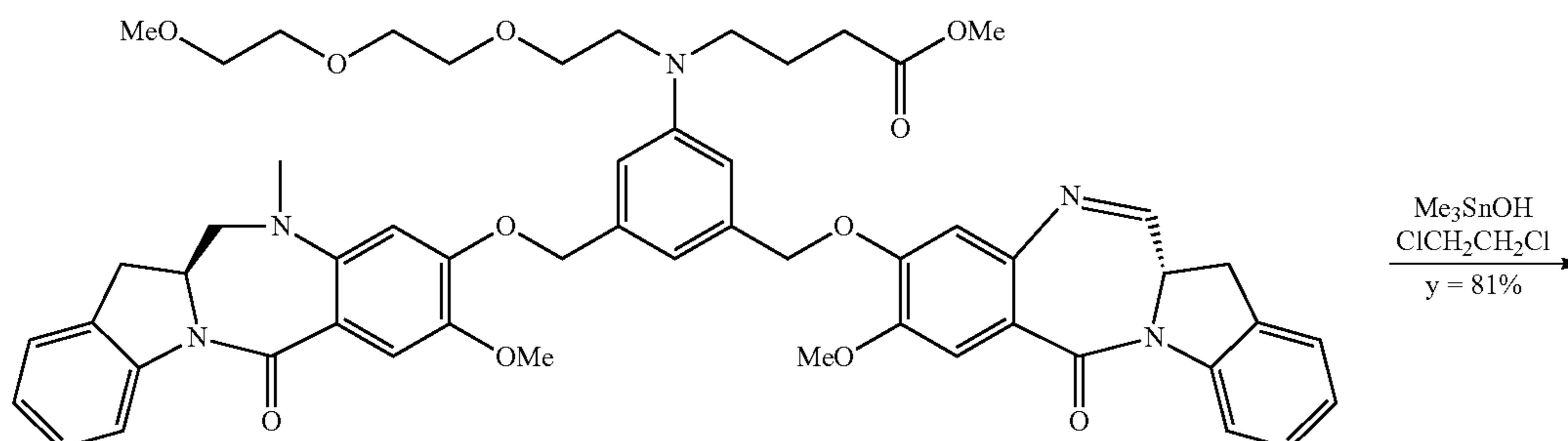
256d (IGN-29-OMe)
