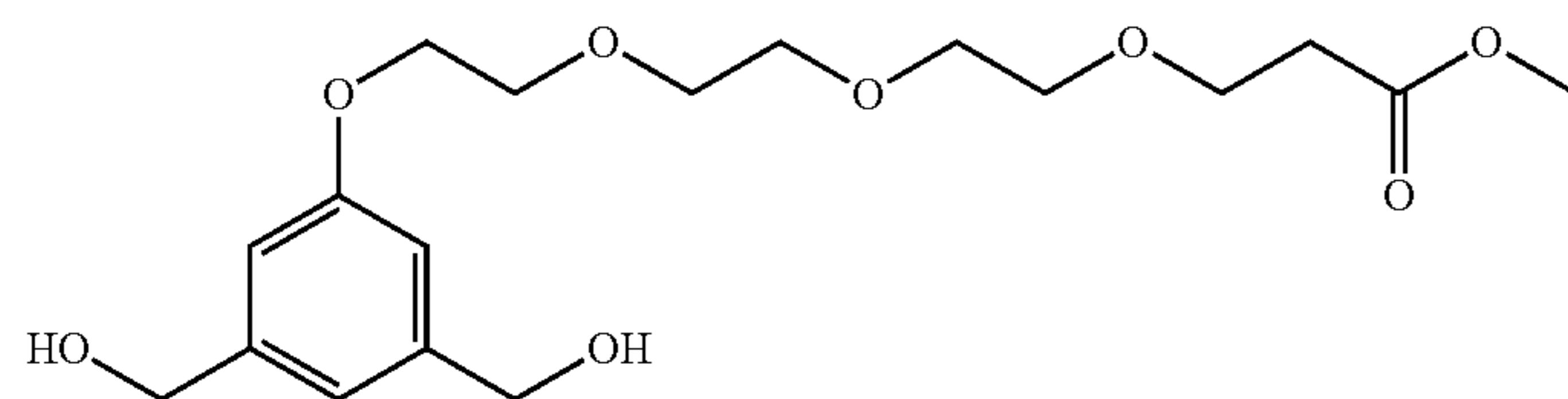
263b
