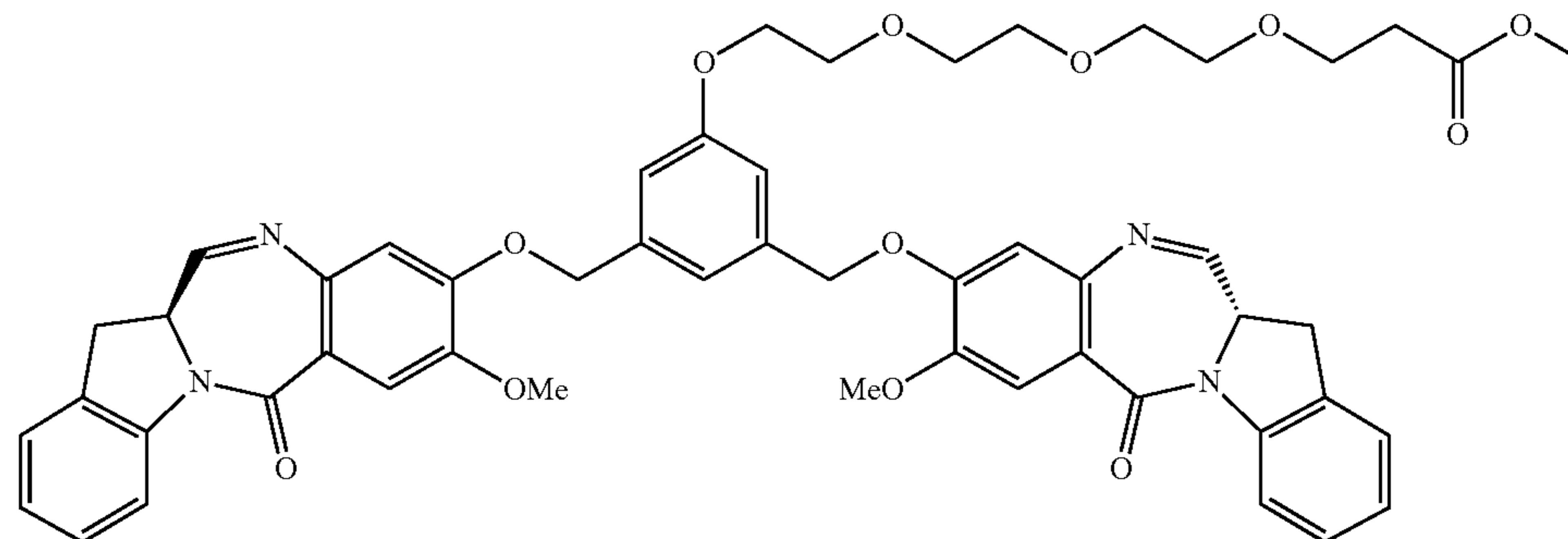
263c
