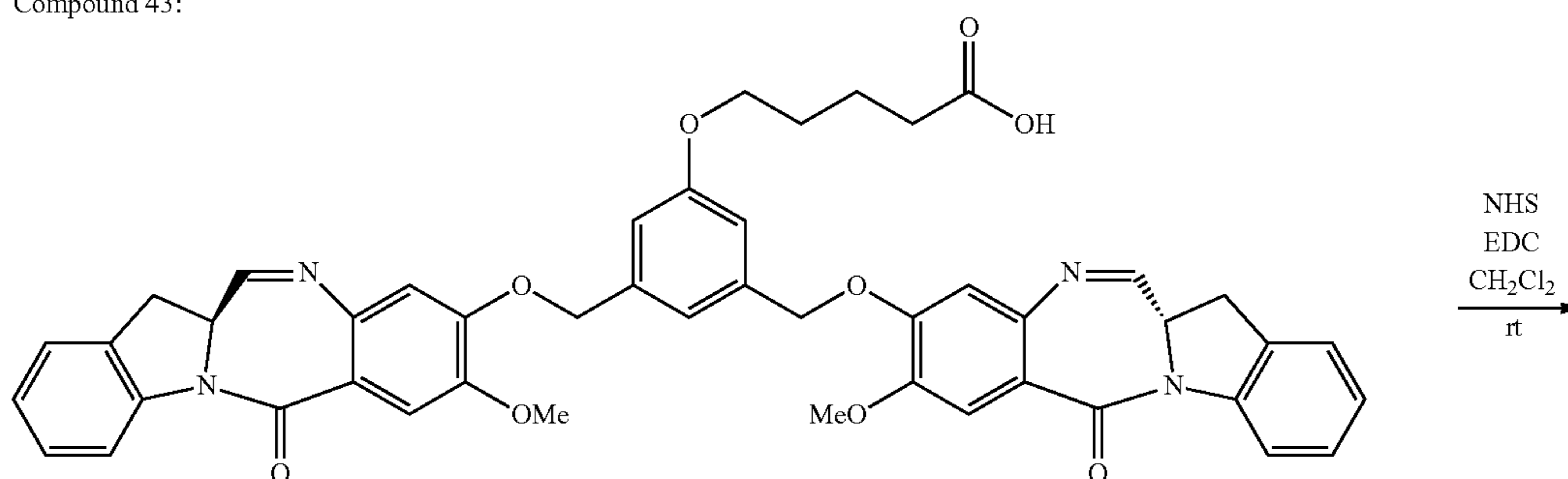
41 (IGN-03 acid)
