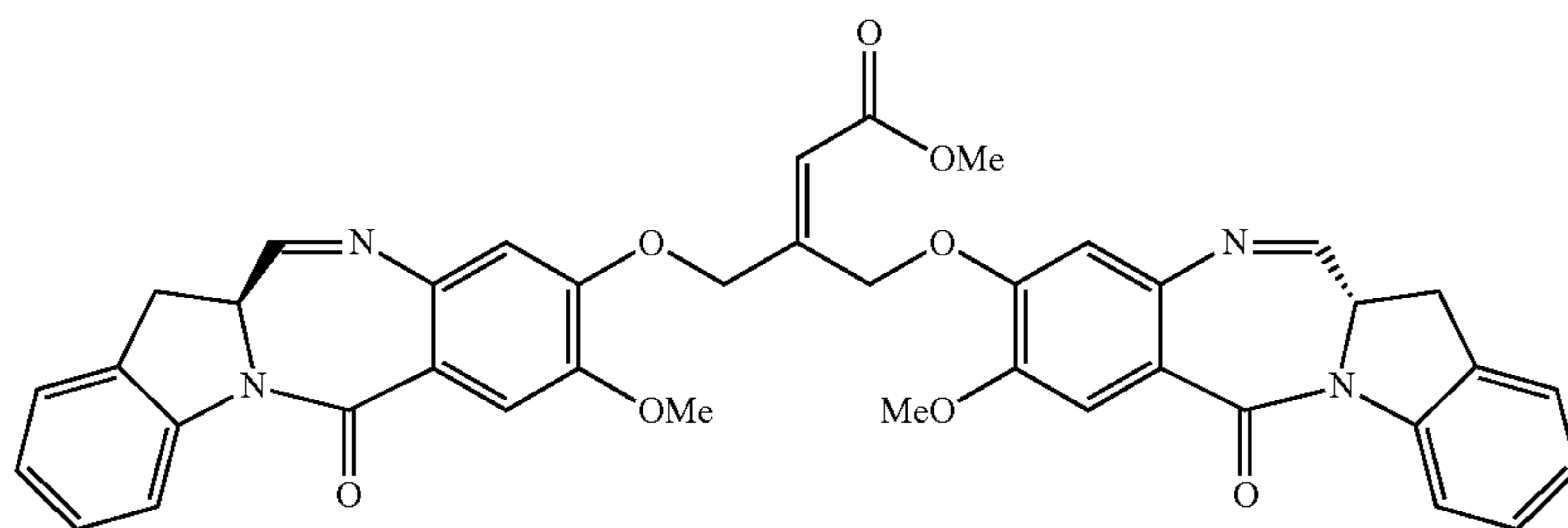
252b (IGN-19-OMe)
