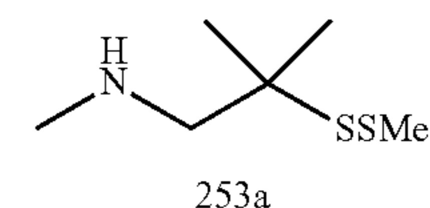
253a
