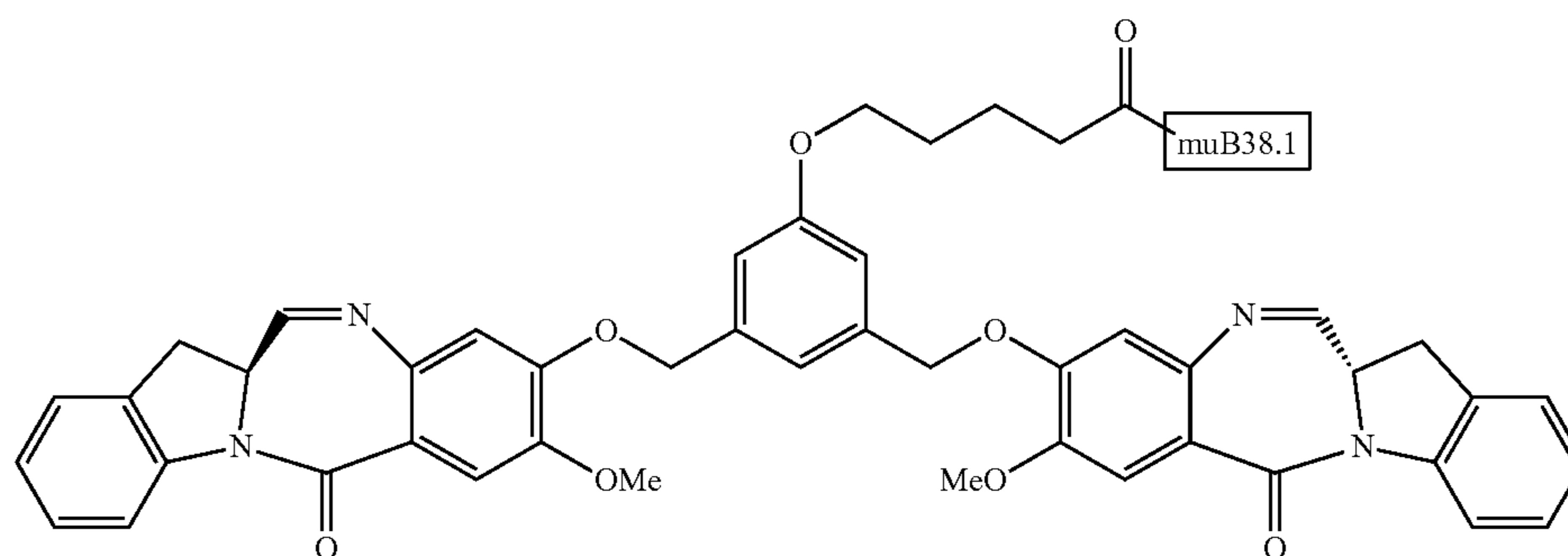
B38.1-IGN-03
