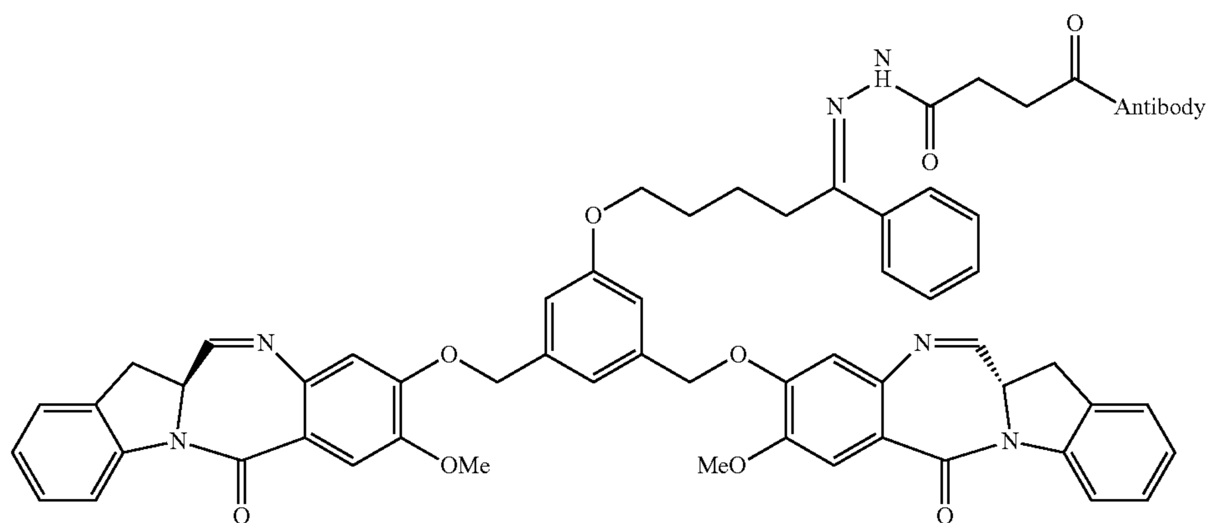
Dimer 4
