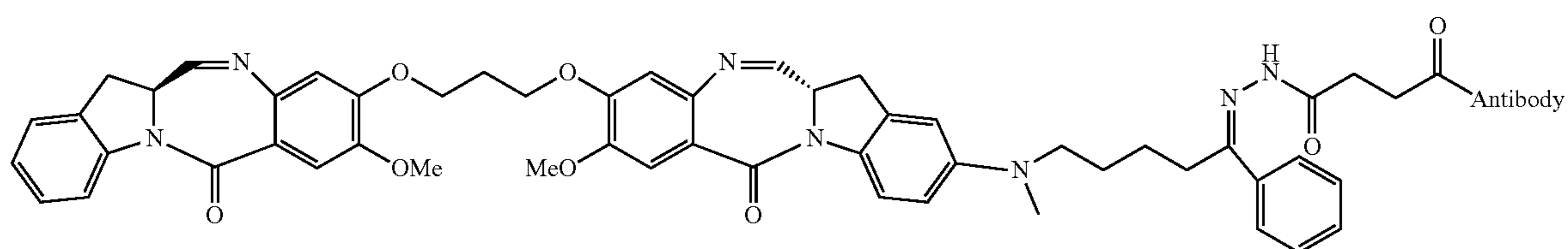
Dimer 8
