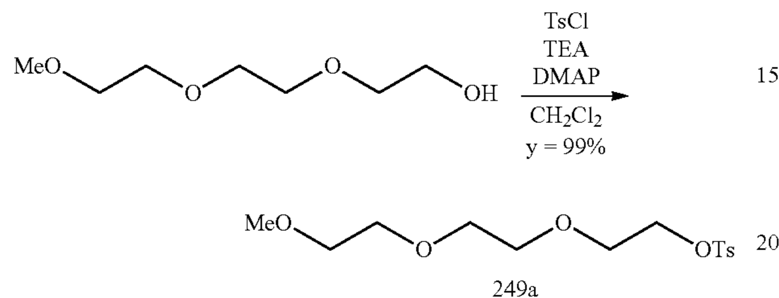
2-(2-(2-methoxyethoxy)ethoxy)ethyl 4-methylbenzenesulfonate
