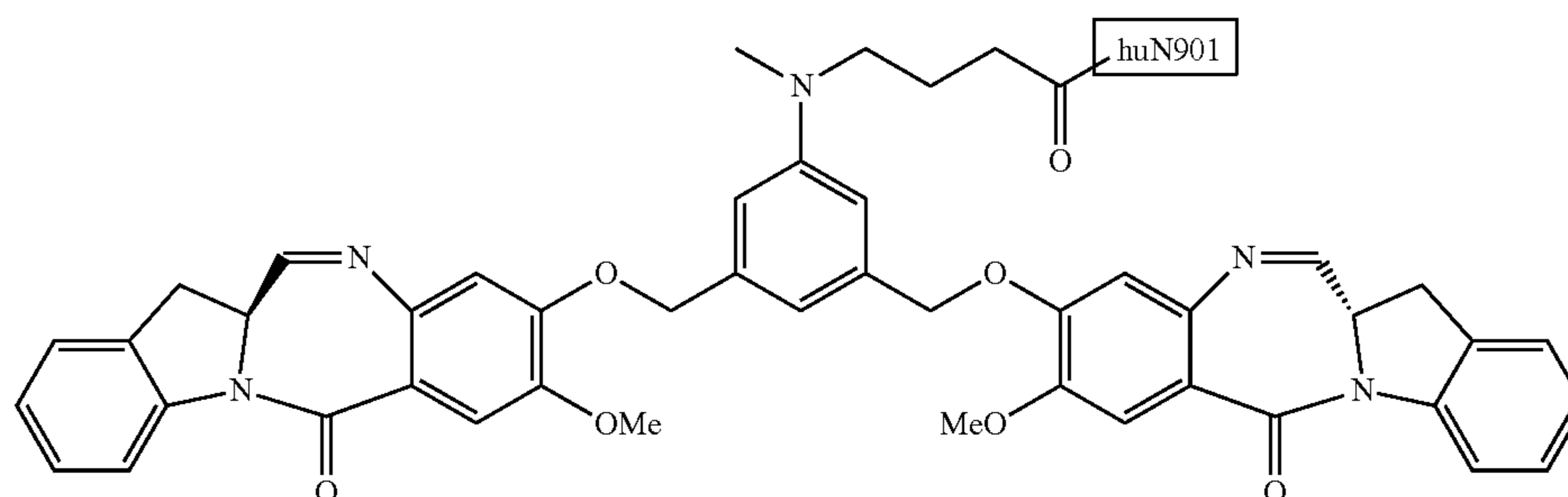
huN901-IGN-07
