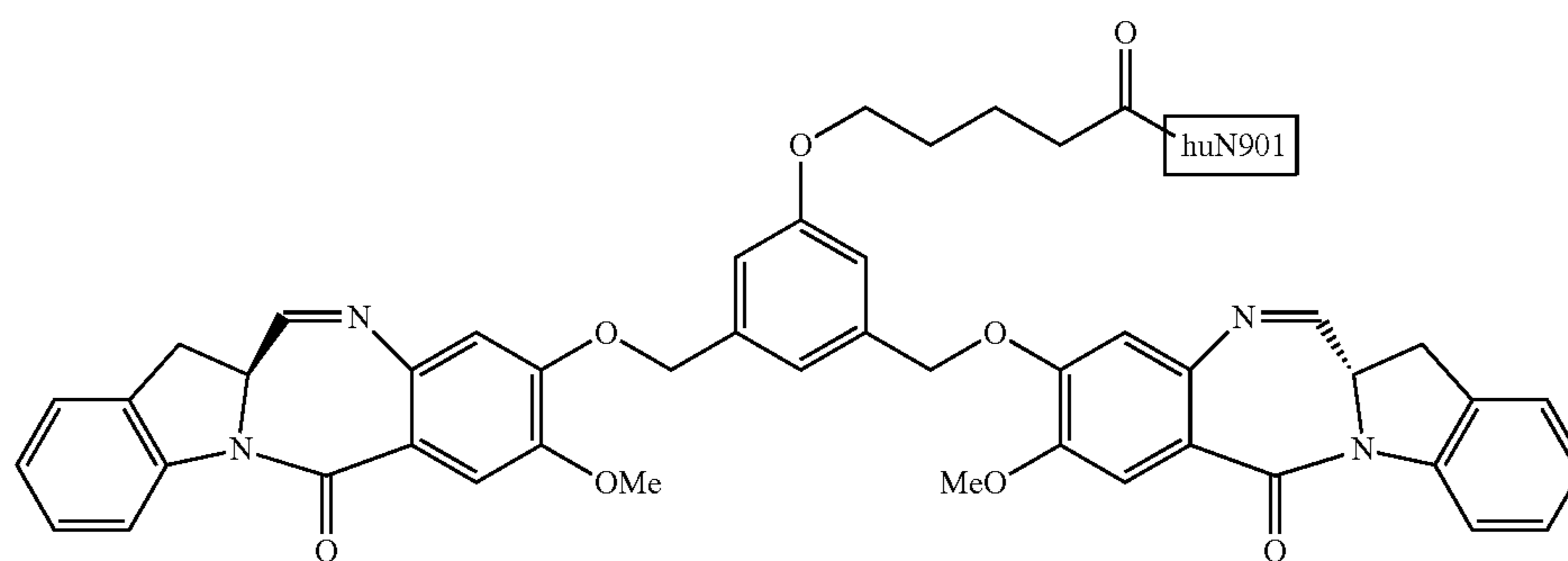
N901-IGN-03
