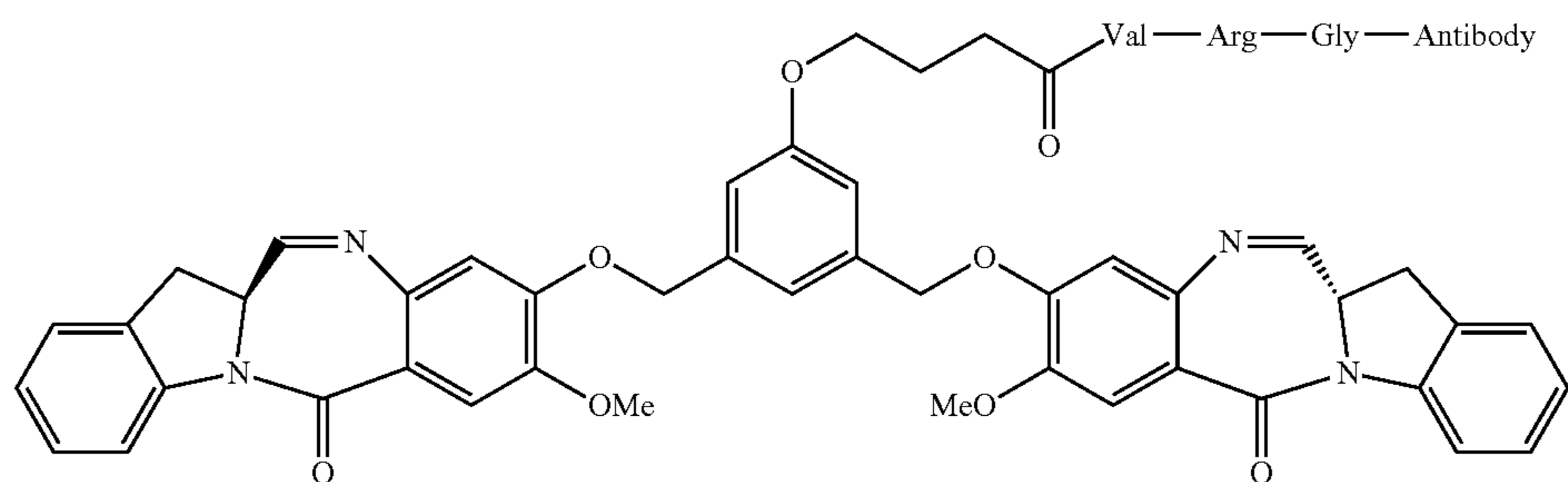
Dimer 2
