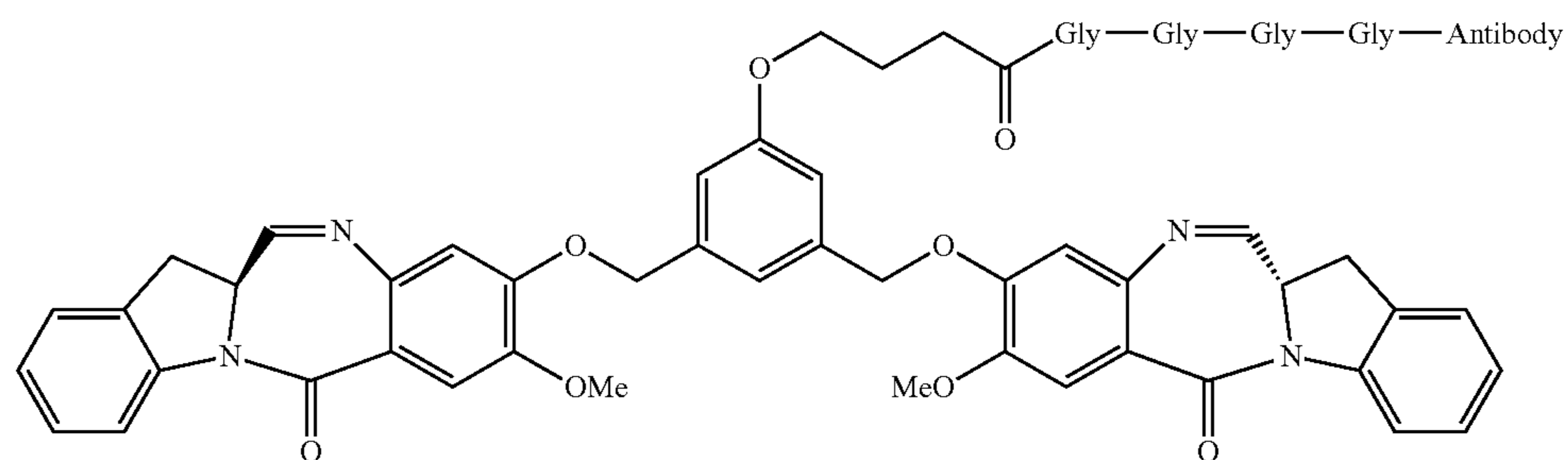
Dimer 1
