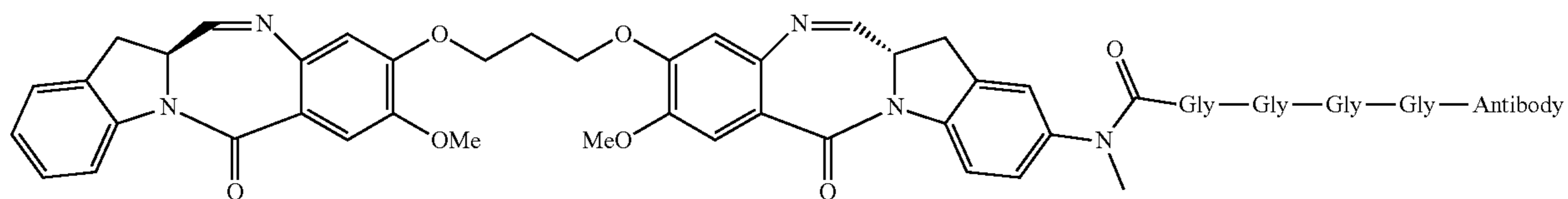
Dimer 6
