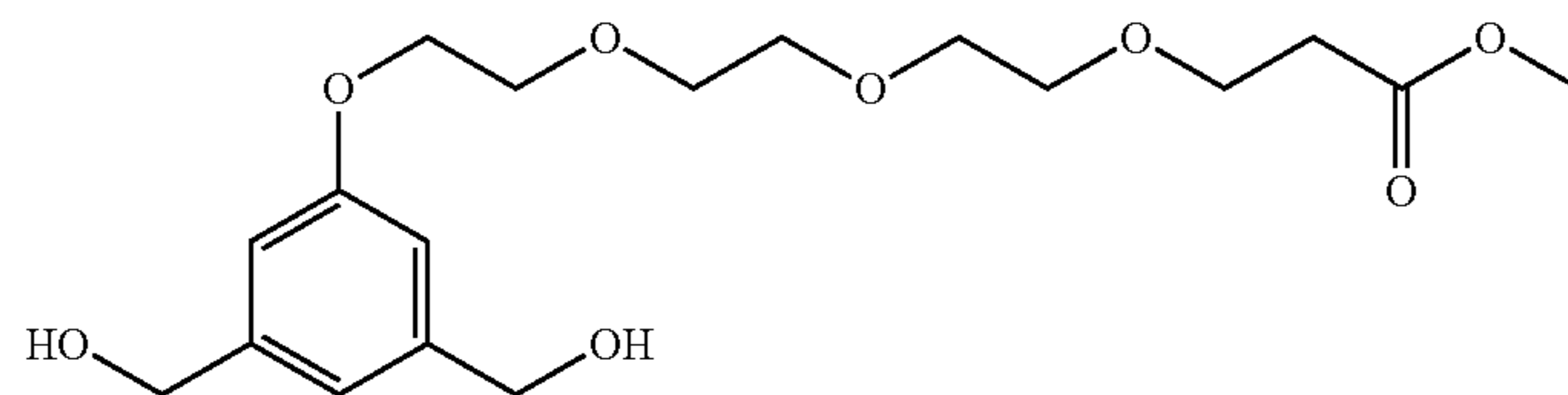
263b
