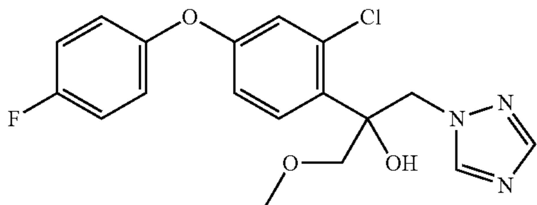
I-28 2-[4-(4-chlorophenoxy)-2-(trifluoromethyl)phenyl]-1-(1,2,4-triazol-1-yl)pentan-2-ol
