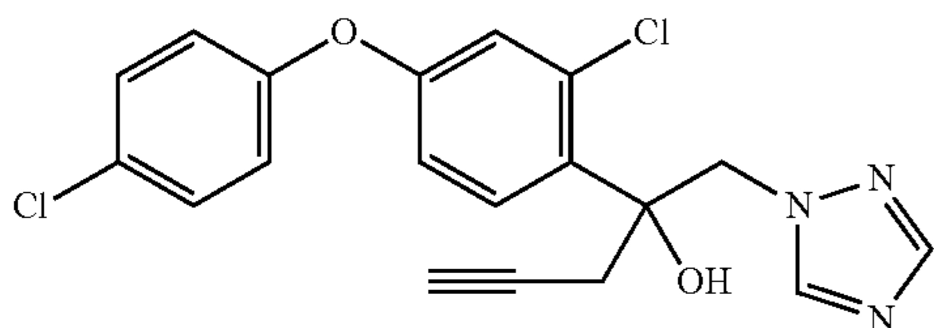
I-26 2-[2-chloro-4-(4-chlorophenoxy)phenyl]-1-methoxy-3-(1,2,4-triazol-1-yl)propan-2-ol
