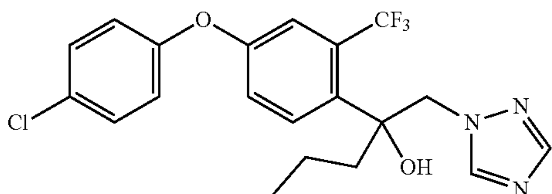
I-29 2-[4-(4-fluorophenoxy)-2-(trifluoromethyl)phenyl]-1-(1,2,4-triazol-1-yl)propan-2-ol
