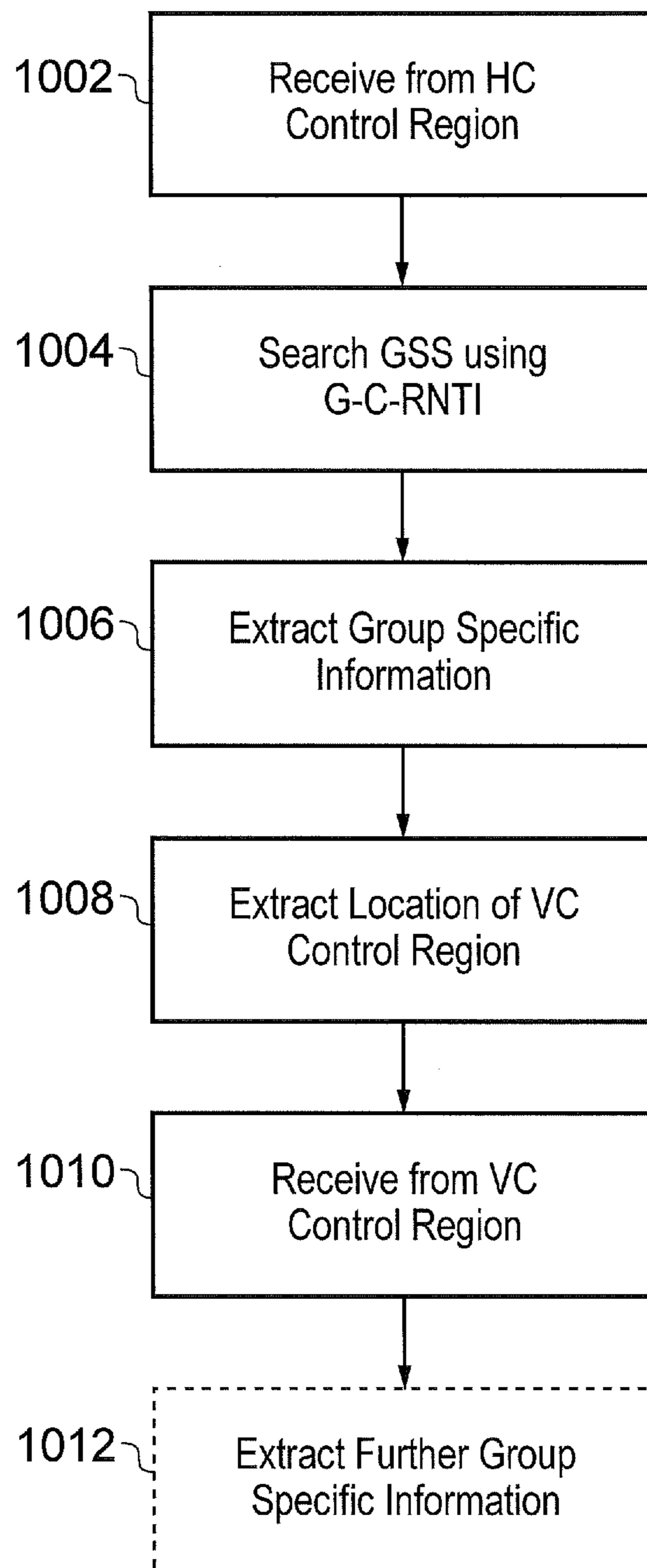
FIG. 10
