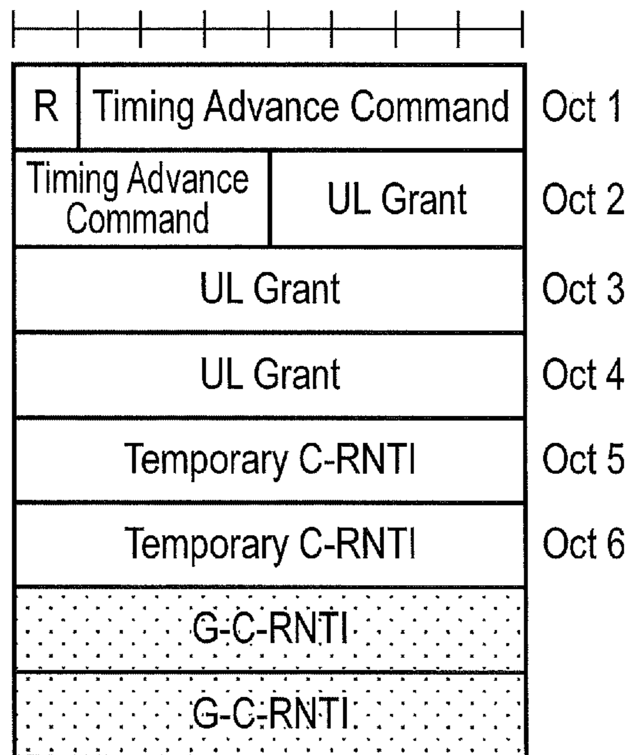
FIG. 8C
