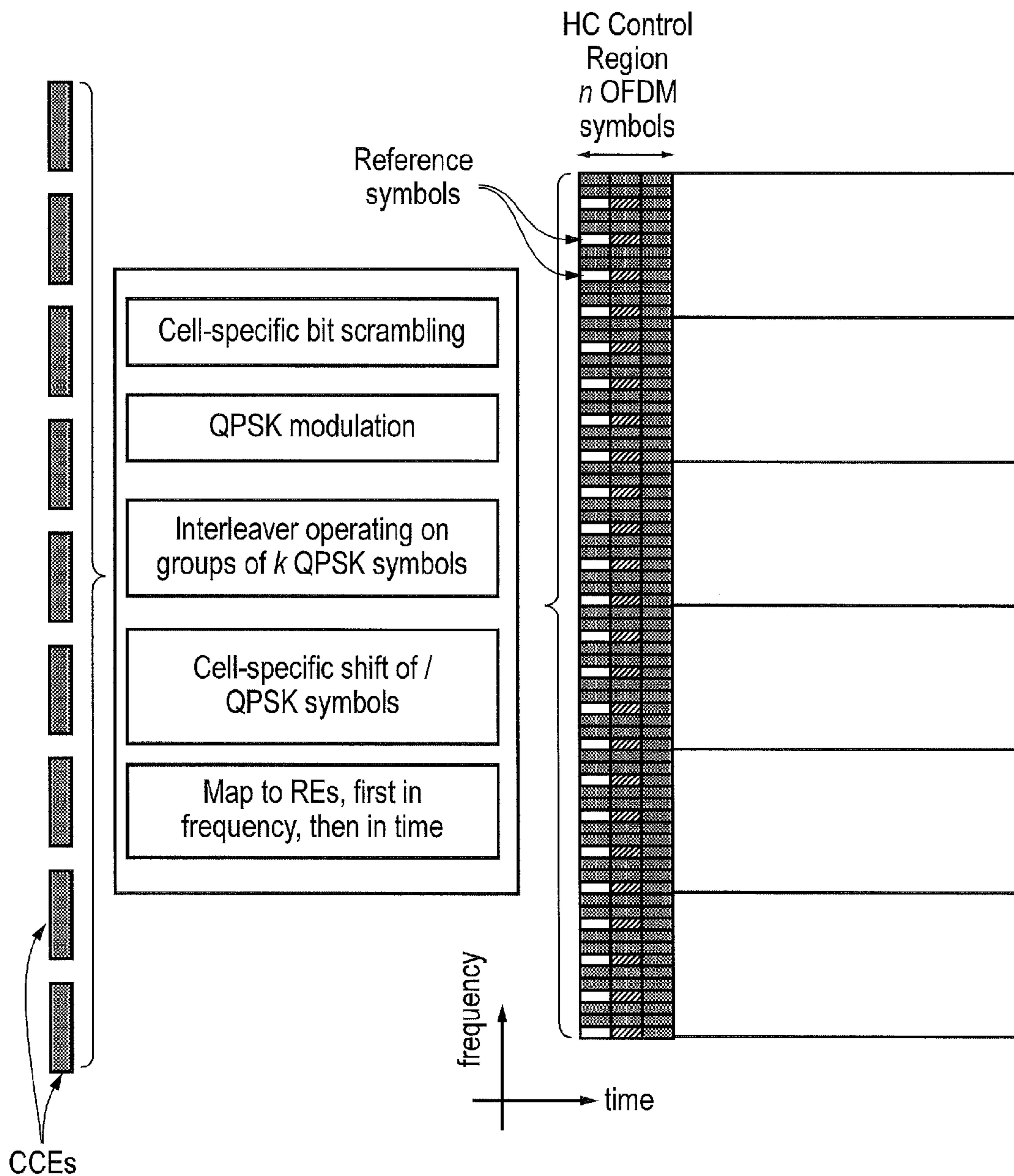
FIG. 6C
