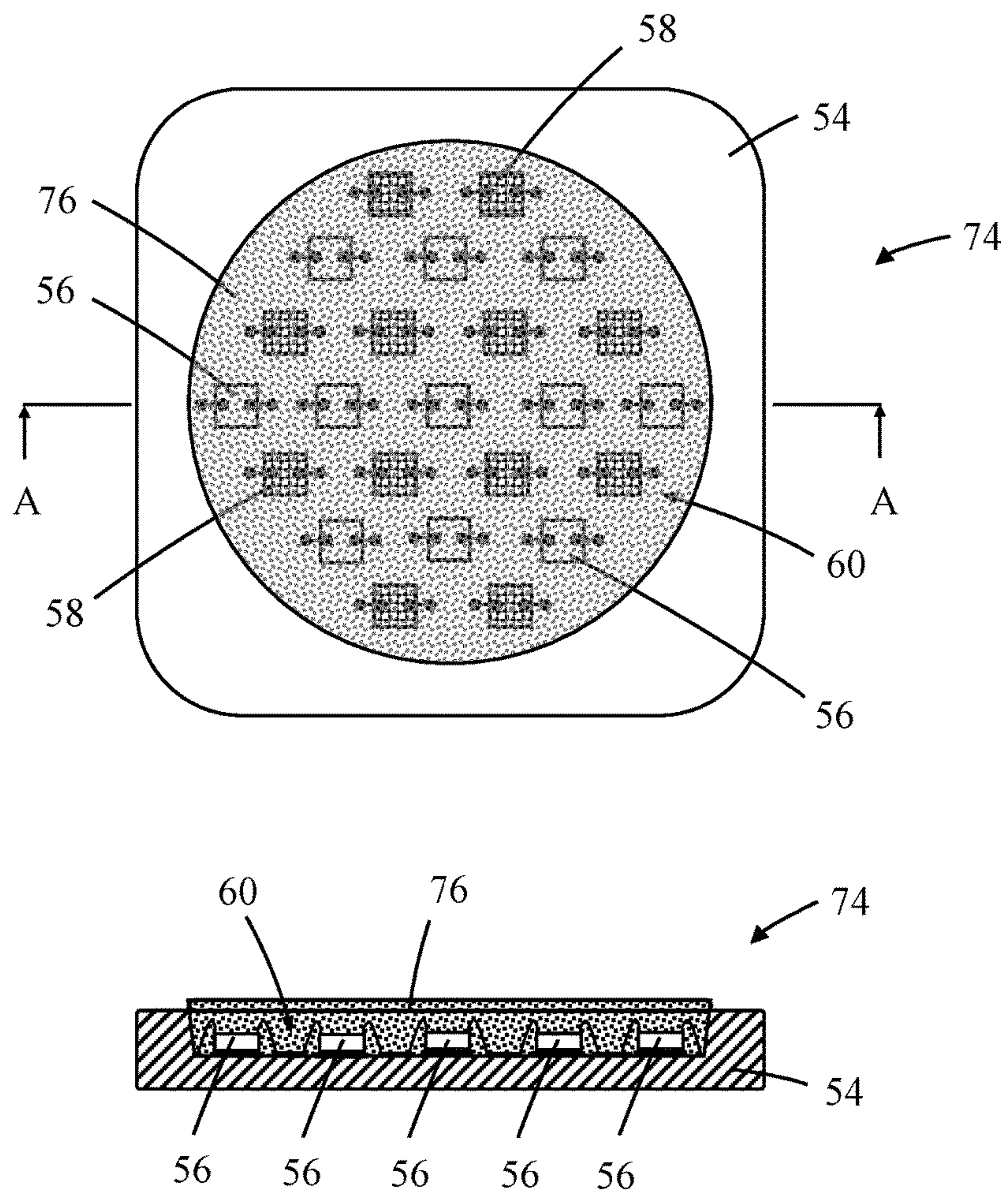
Section A-A
