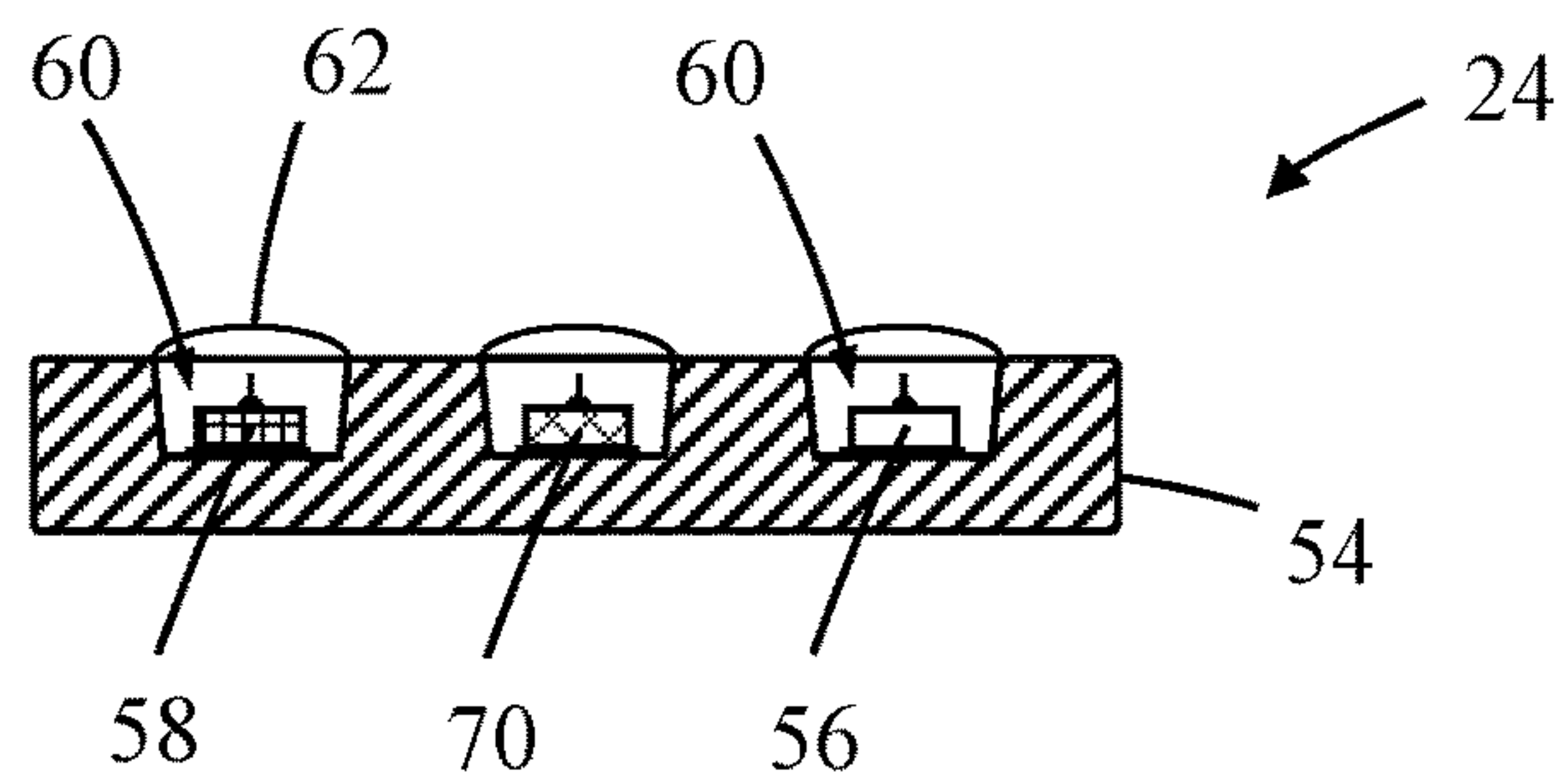
Section A-A
