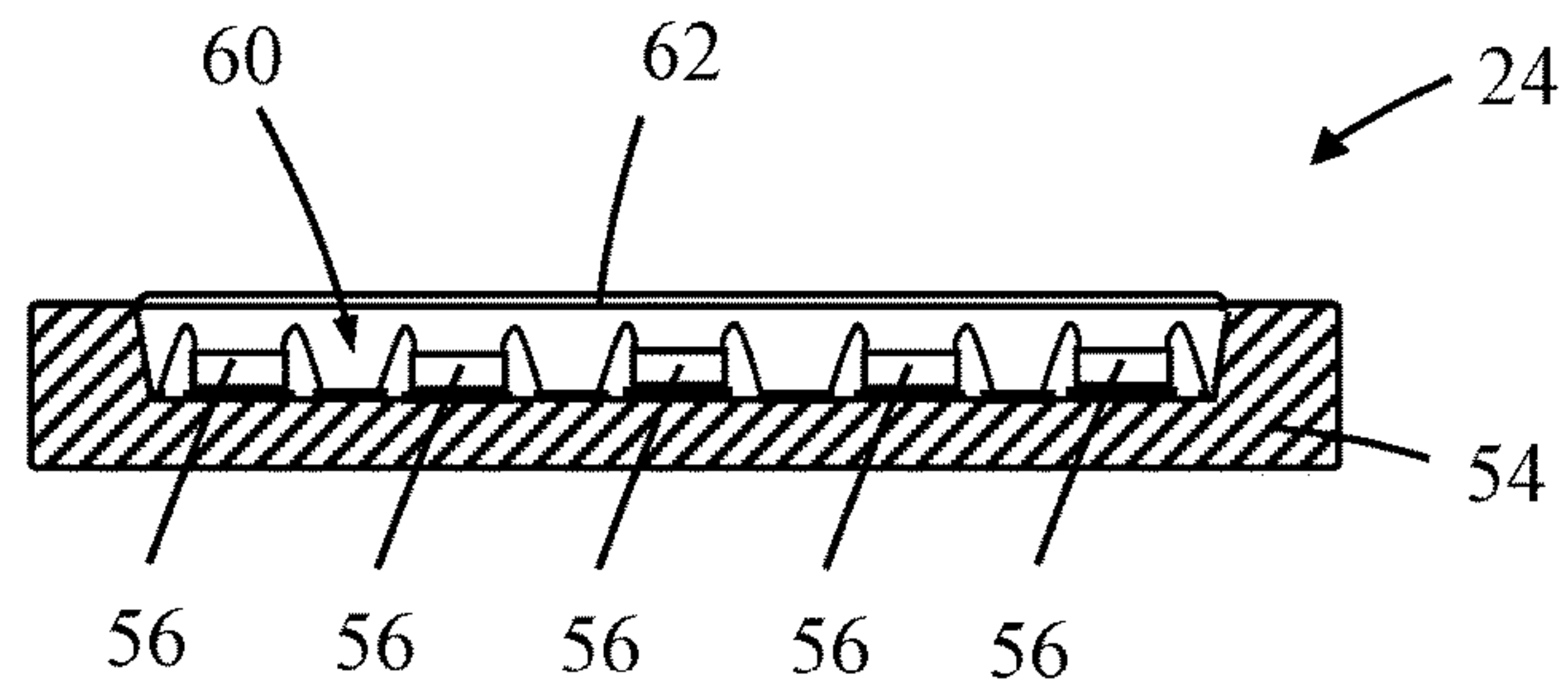
Section A-A
