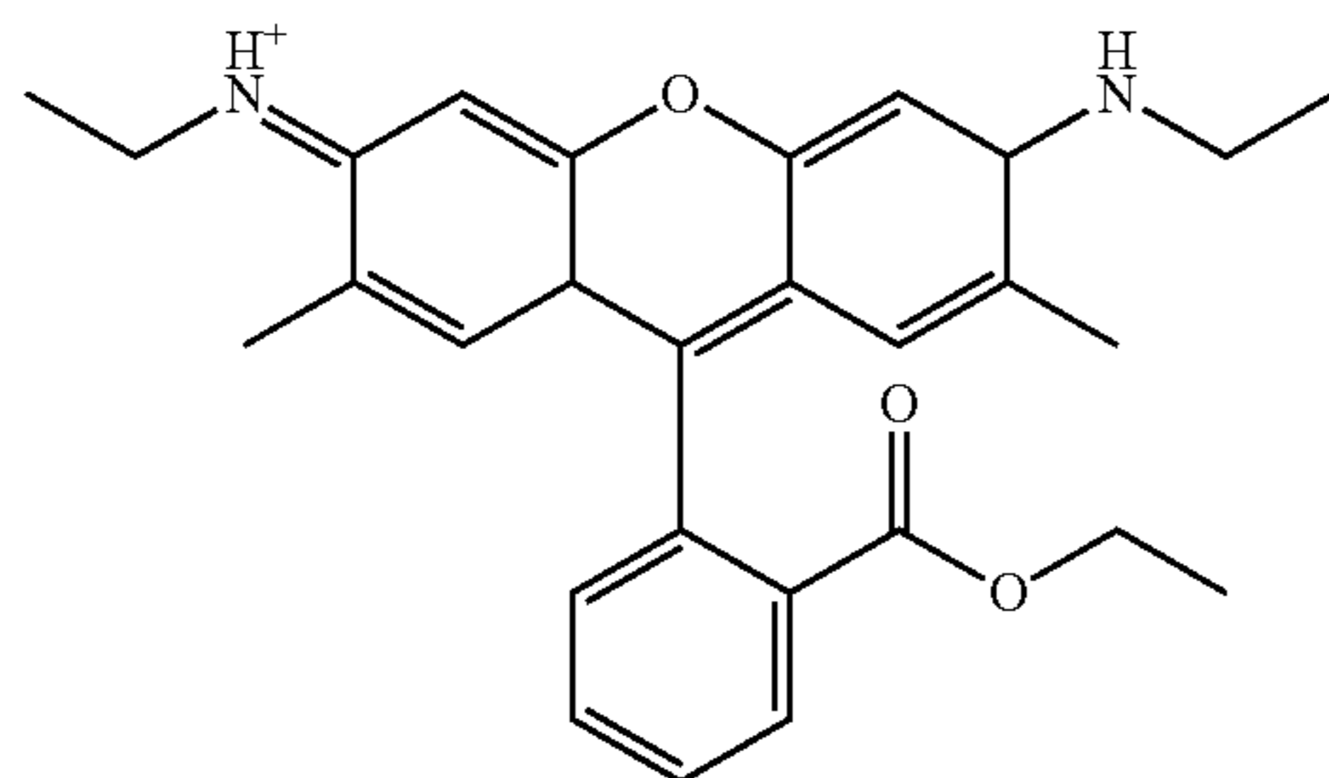
Rhodamine 6G
