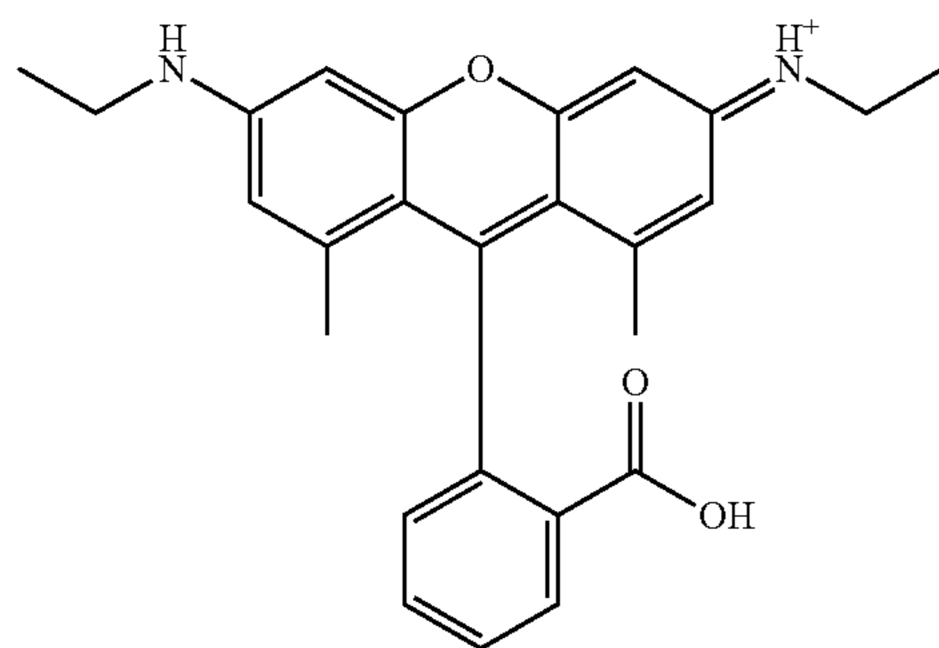
Rhodamine 575
