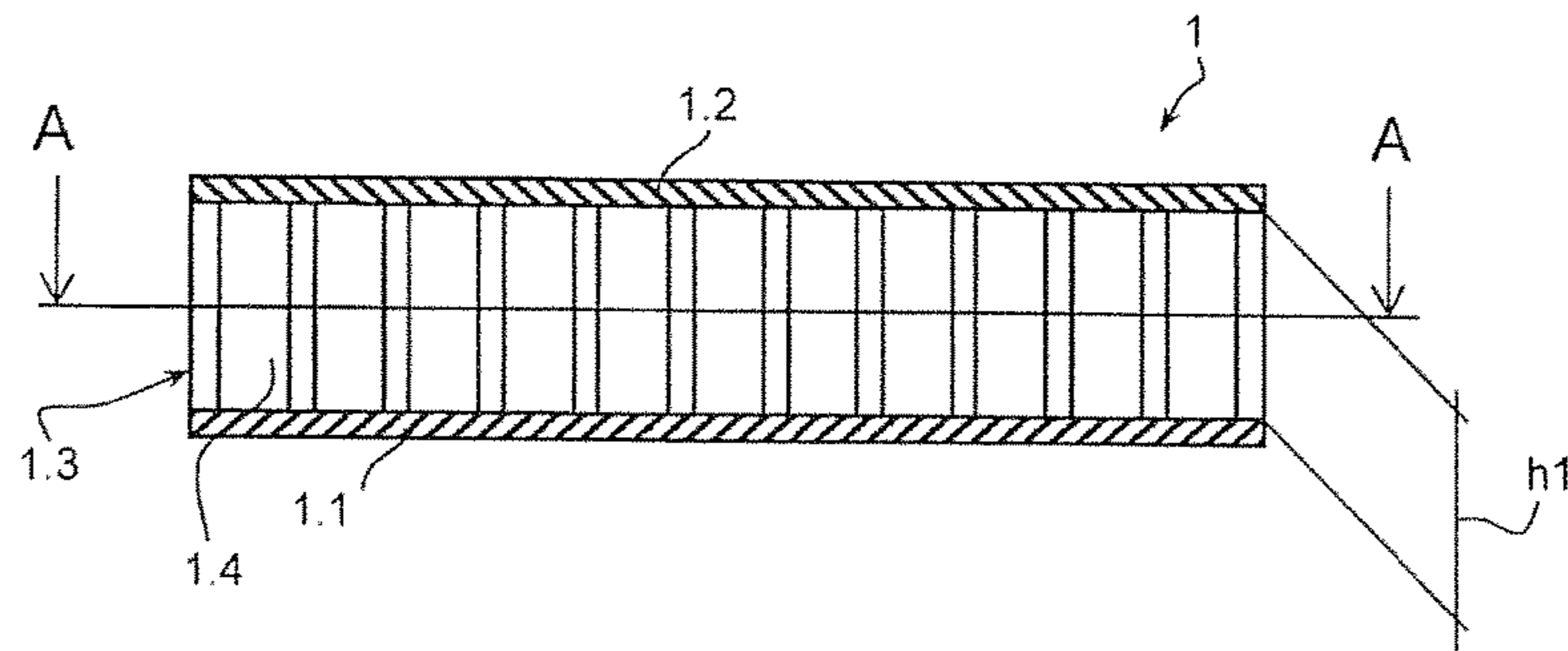
Fig. 1a B-B
