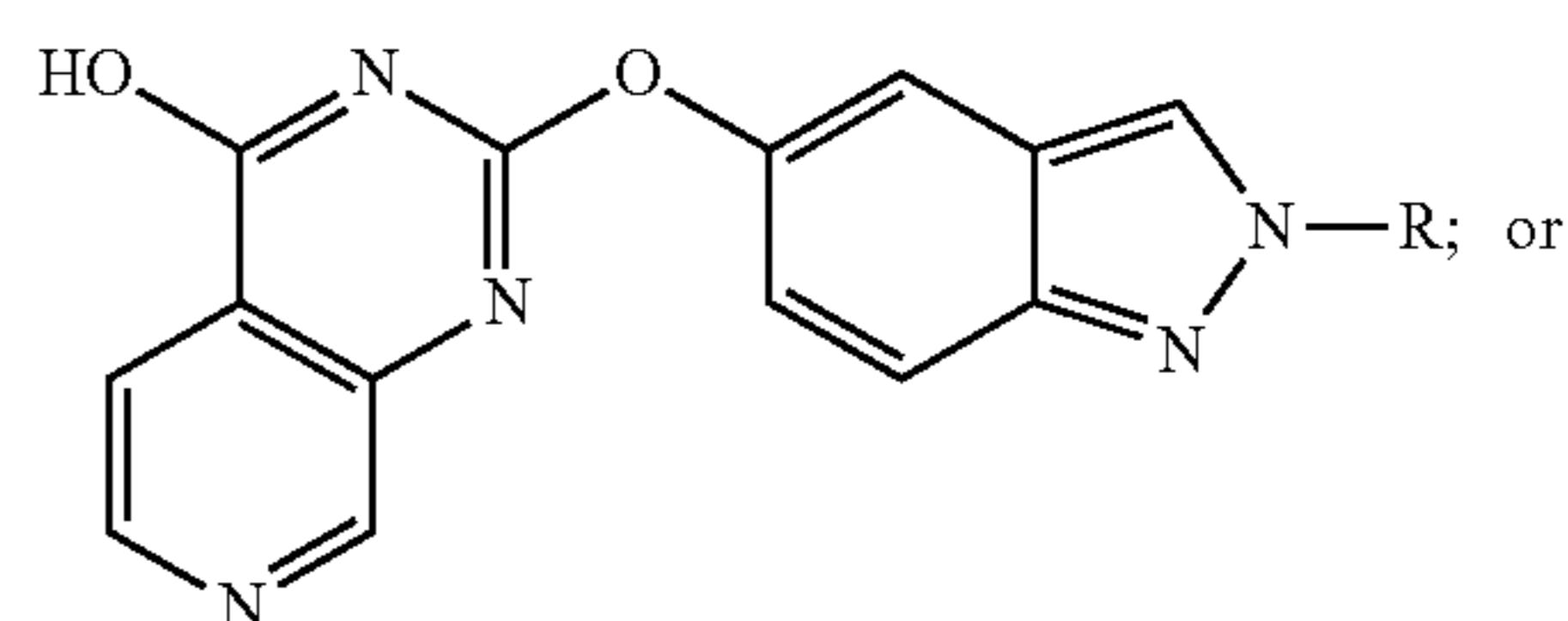
Formula (VIId)
